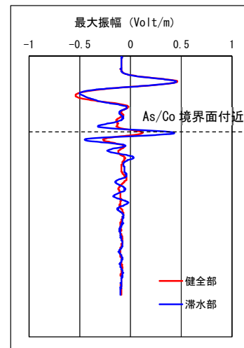
図-8 健全部と滞水部の振幅
