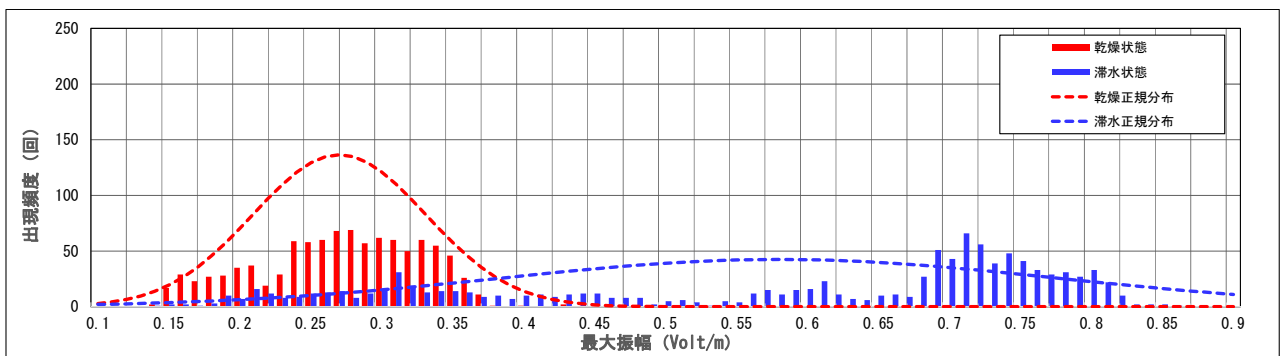
図-9 電磁反射波の最大振幅の頻度分布
