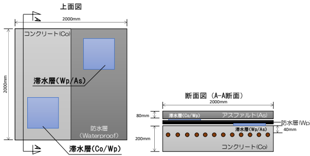
図-1 模型床版概要図
