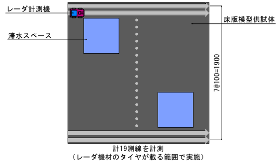
図-3 計測概要図
