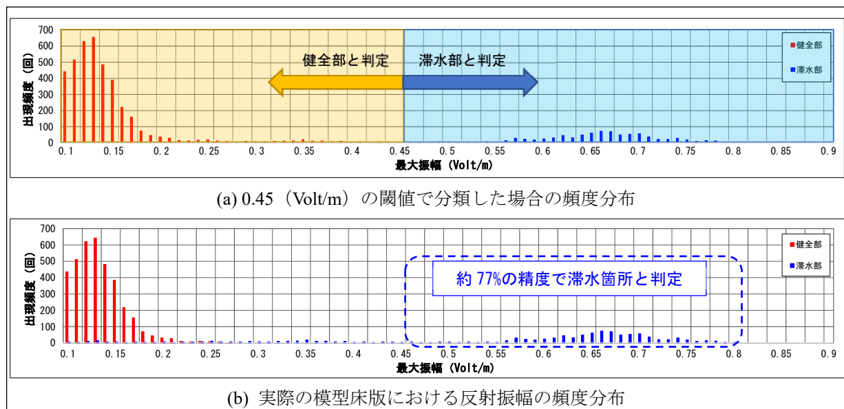
図-11 滞水検知モデルで分類した結果と模型床版の真値との比較
