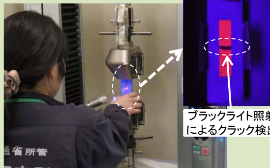
センサー機能を有する材料の実験 (センサー塗膜)
