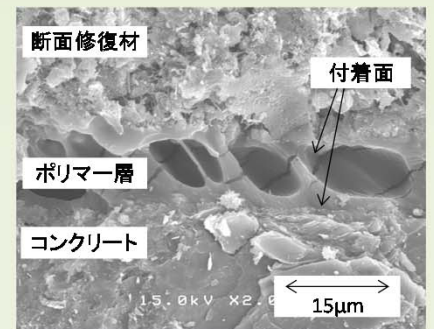
コンクリート用補修材料の付着性状調査
