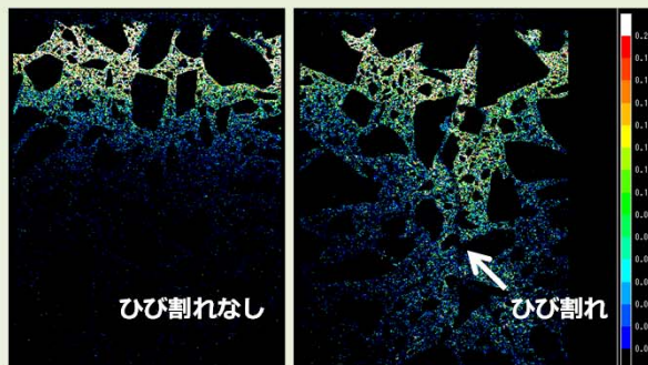
コンクリートひび割れ部の塩分侵入状況の調査
