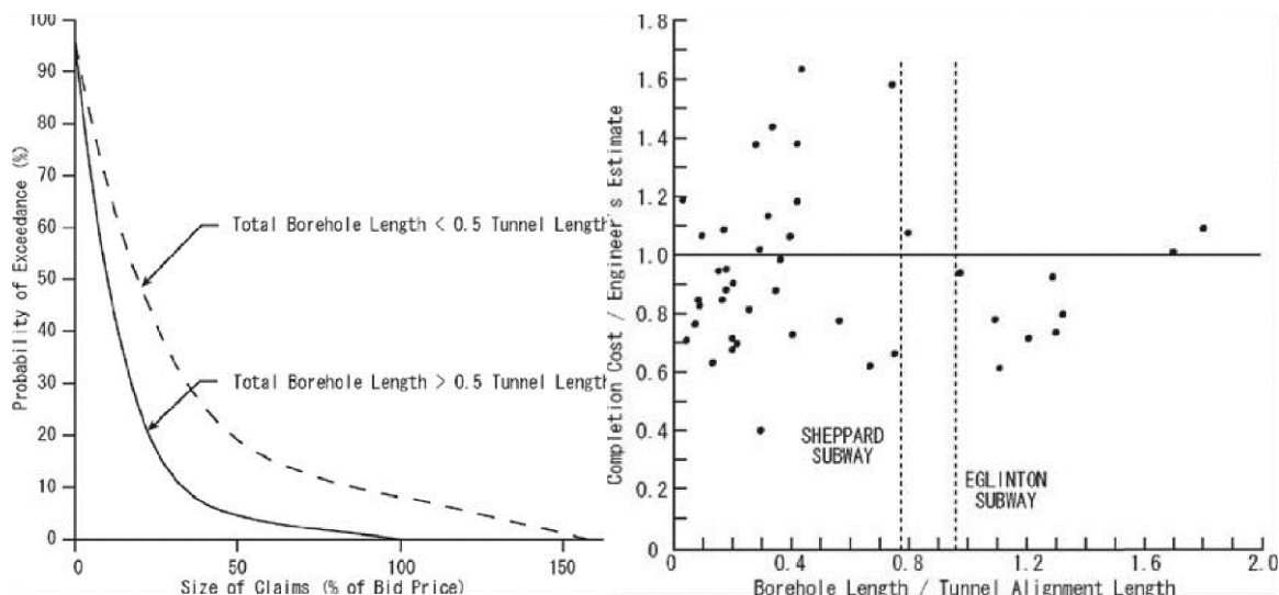
図-3 カナダの地下鉄建設における設計変更の確率と B/T の関係図（左図）及び完成工事費と B/T との関係図（右図） 3)
