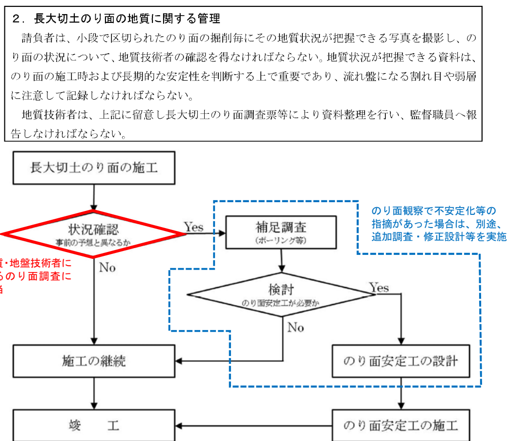
図-17 長大切土のり面の施工の流れ 4) に加筆
