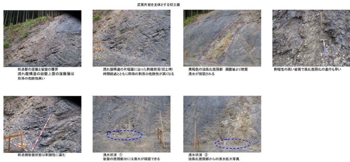
図-18 のり面調査票の作成例 4)
