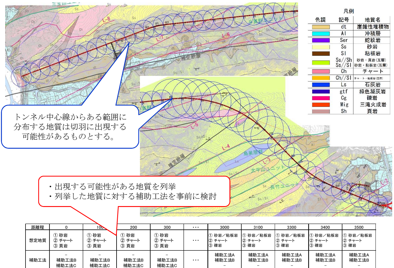
図-4 トンネル切羽に出現する可能性のある地質の幅（不確実性）の見える化 2) に加筆
