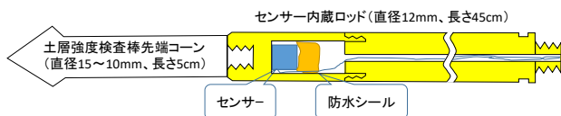
図-15 センサー入りロッド先端部の構造
