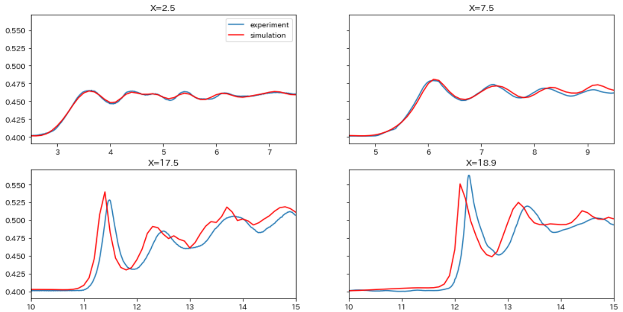
図 12 水位時系列変化の実験と数値計算の比較 (Case1)
