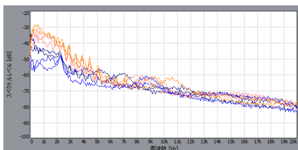
図-16 加速度センサー (X軸) のパワースペクトル (0k~20kHz) 橙、朱は砂質土、紺、青は粘性土。
