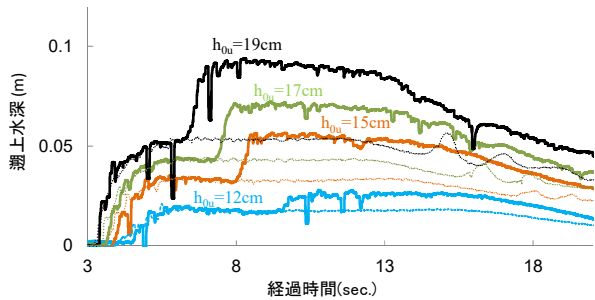
図-17 アイスジャム形成時(実線)および氷群なし(点線)の場合の潮上水深の経時変化(勾配変化点)
