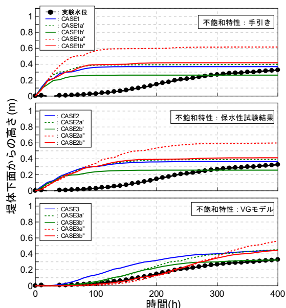
図3-4 透水係数の異方性による水位の比較
