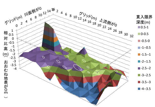
図-7 グリッド土検棒調査による3D貫入限界深度図 白丸は2017年の噴砂痕位置
