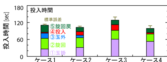
図4 ブロック投入平均時間 (1個当り)
