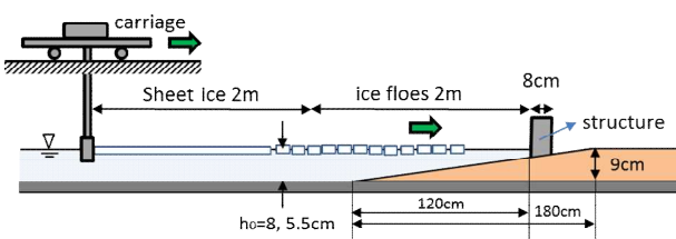
図-25 海氷の陸上遡上実験装置
