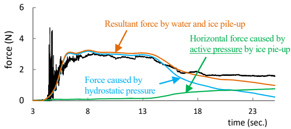
(a) 角柱構造物 (図-5 に対応)
