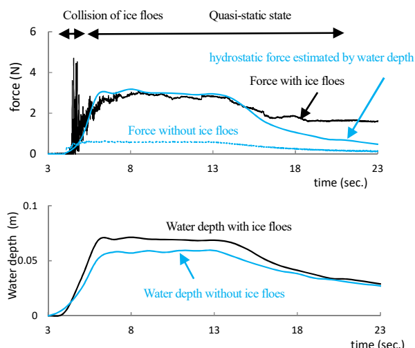
図-5 アイスジャム形成時の構造物に作用する主流方向の荷重と構造物前面水深の経時変化および氷群なしの場合との比較例 ( W=4\text{cm} , B=9\text{cm} , h_u=0.17\text{m} )
