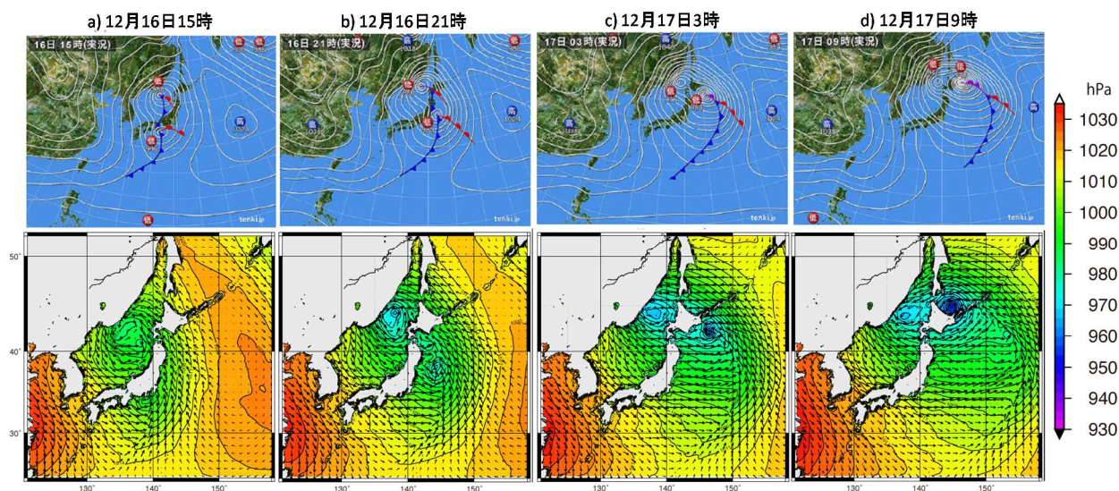
図-22 爆弾低気圧通過時の天気図 (上段) と WRF による気圧・風場の計算結果 (下段)
