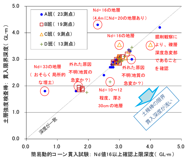
図-8 Nd 値 16 以上確認上限深度と土検棒の貫入限界深度との関係 4)
