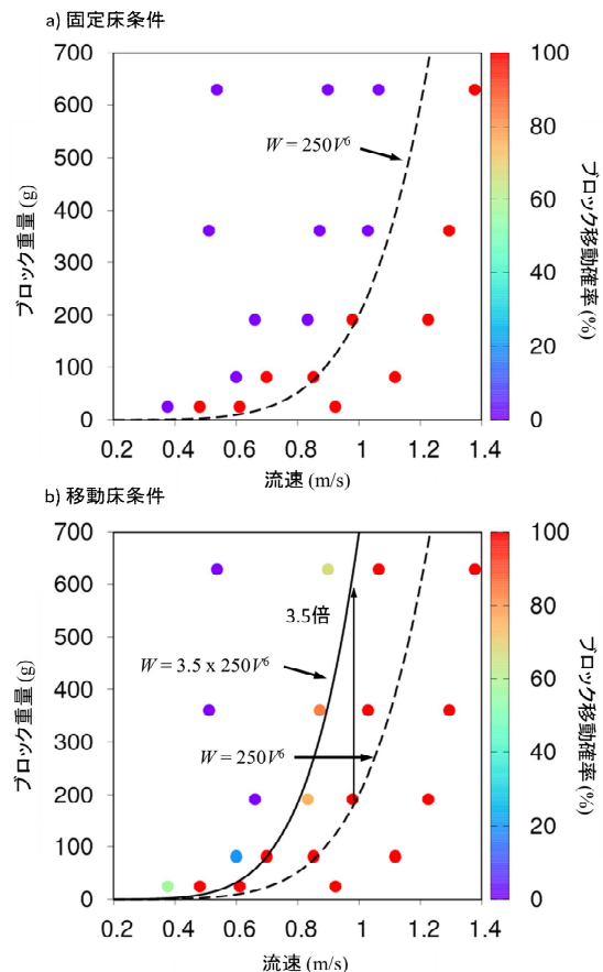
図-15 三角波発生条件におけるブロック移動確率と流速—ブロック重量の関係。 a)固定床, b)移動床。
