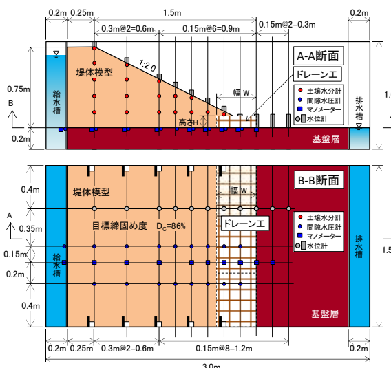
図 5-1 実験模型図
