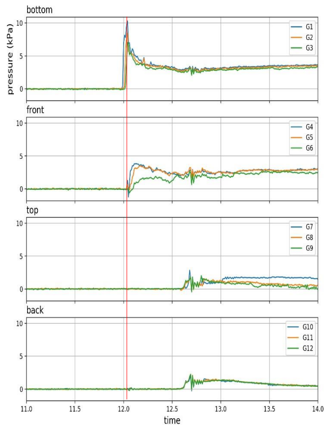
図8 実験時の波高の推移 (Case5_3)
