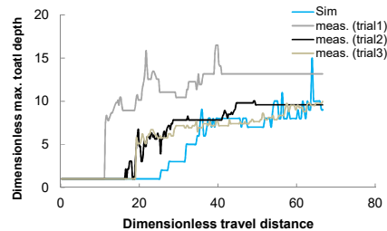
図-26 (a) 氷の遡上分布の実験と計算結果の比較例 横断方向に断続的に一列に配置した場合
