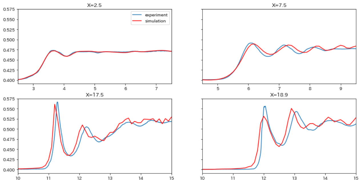
図 14 水位時系列変化の実験と数値計算の比較 (Case3)
