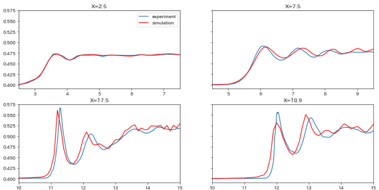
図 13 水位時系列変化の実験と数値計算の比較 (Case2)
