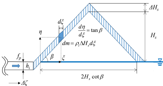
図-24 パイルアップモデル
