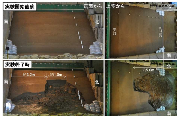
写真 2-1 実験前後の模型の状況
