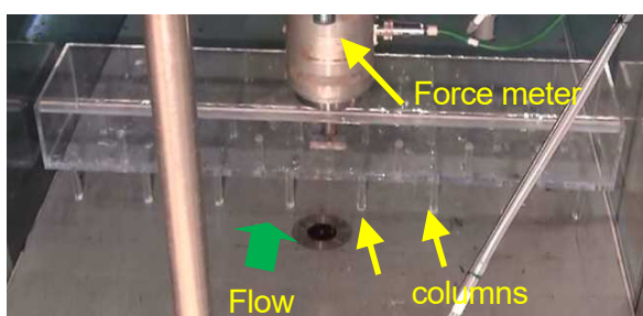
図-4 プロティ構造模型 (実験③)
