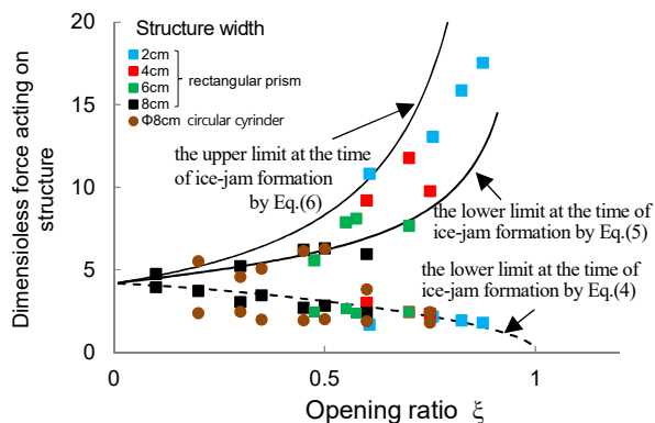
図-16 開口率 \xi と建築物に作用する主流方向の荷重(単位幅あたりの無次元量)との関係及び計算値との比較例 ( h_0=17\text{cm} )
