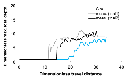
図-26 (b) 氷の遡上分布の実験と計算結果の比較例 水路半分側に連続配置した場合
