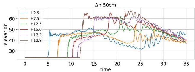
図7 実験時の波高の推移 (Case5_3)
