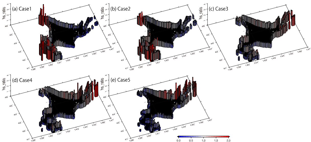
図-31 再現実験と各実験における有義波高の最大値の比 (Case1~5/CTL-run) .
