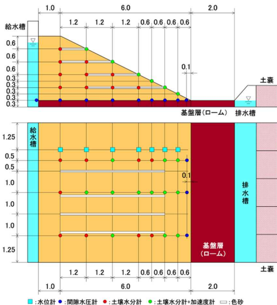
図 2-1 実験模型図
