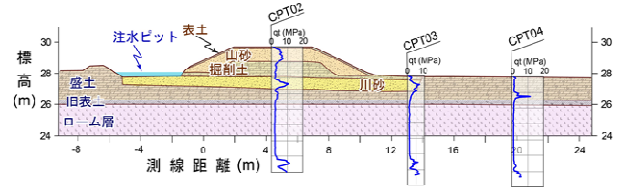
図 1.2.8 高浸透基盤を持つ模擬堤防の土質構成 16)
