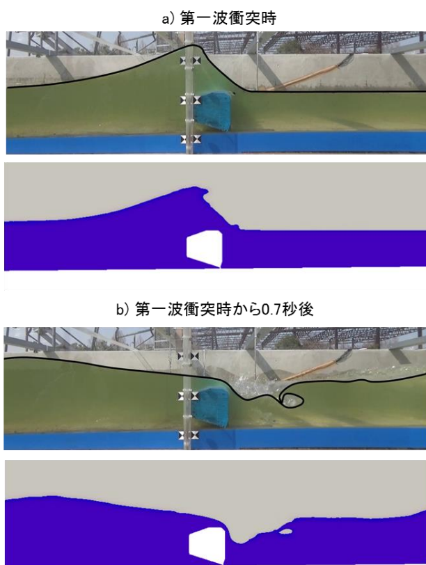
図 15 ゲート周辺での水面形詳細 (Case1) (それぞれの時刻で上: 実験動画、下: 数値計算結果。数値計算結果は青が液体でグレーが気体を表す)
