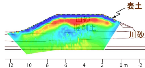
図 1.2.10 強雨時の比抵抗変化 (48時間)
