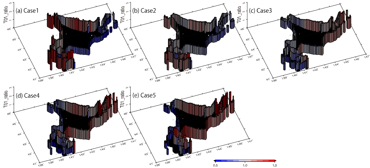
図-32 再現実験と各実験における有義波周期の最大値の比 (Case1~5/CTL-run)
