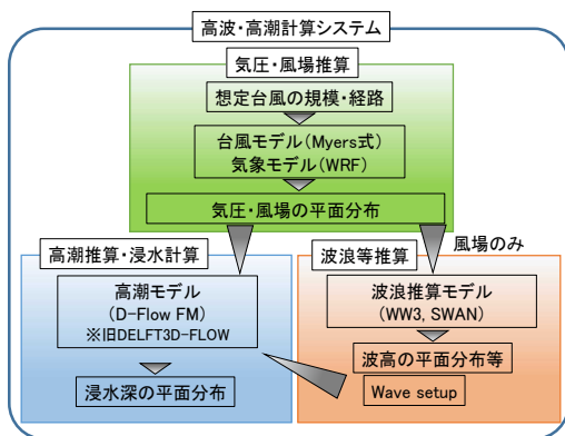
図-20 高波・高潮の計算フロー図
