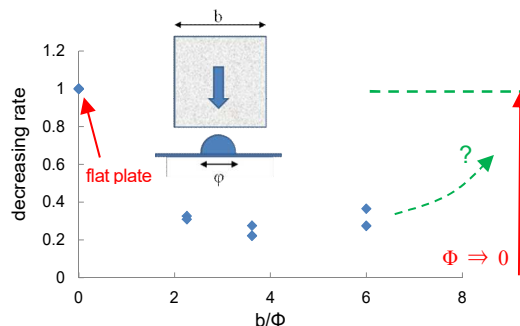
図-23 半円筒構造物径が及ぼす荷重軽減効果
