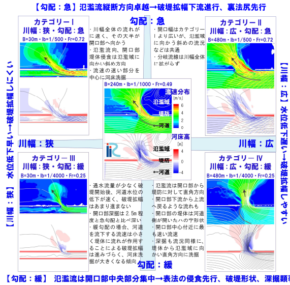
図-7 河道特性に応じた堤防決壊現象の分類
