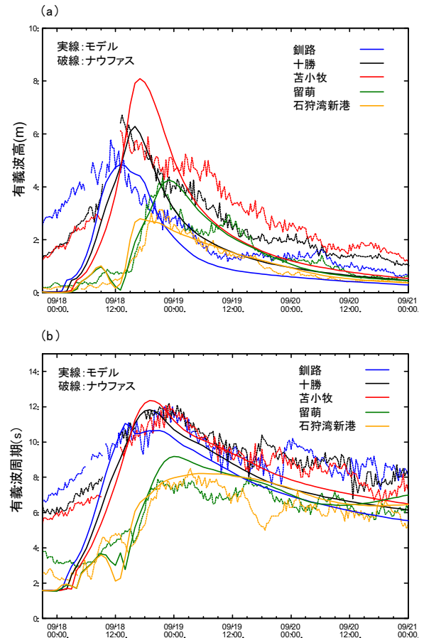
図-29 ナウファス (観測値) と CTL-run (計算値) の有義波高(a)と有義波周期(b)の時系列
