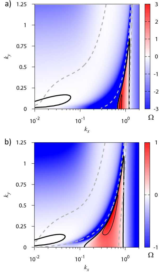
図-16 三次元擾乱に対する増幅率コンター図。a) 二次元河床波 ( k_y=0 で増幅率最大となる。 F_r=0.95 、 \tau_0=0.1 、 C_f=1/11.3^2 )、b) 三次元河床波 ( k_y \neq 0 で増幅率最大となる。 F_r=1.25 、 \tau_0=0.16 、 C_f=1/10.6^2 ) の例。黒の実線が中立曲線、グレーの破線が伝播速度がゼロとなる曲線を意味しており、三本の破線で分けられる四つの領域における擾乱の伝搬速度は、左から順に、負、正、負、正である。
