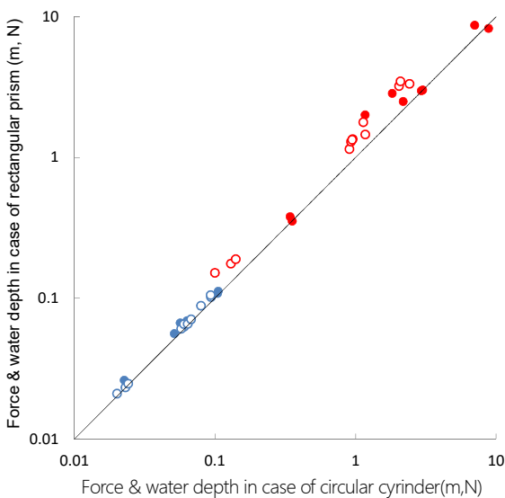
図-8 衝突力を除く準定常状態における作用力と水深の時間平均値を円柱と角柱との比較
