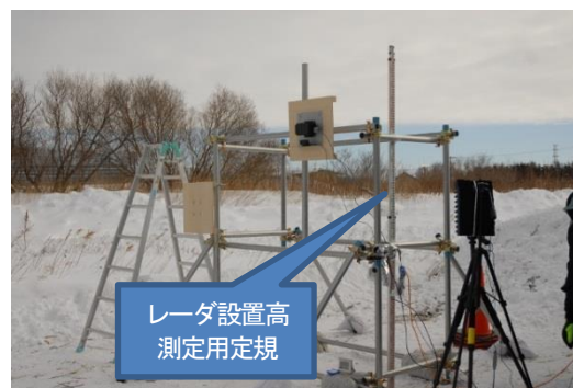
写真-22 ミリ波レーダ設置状況
