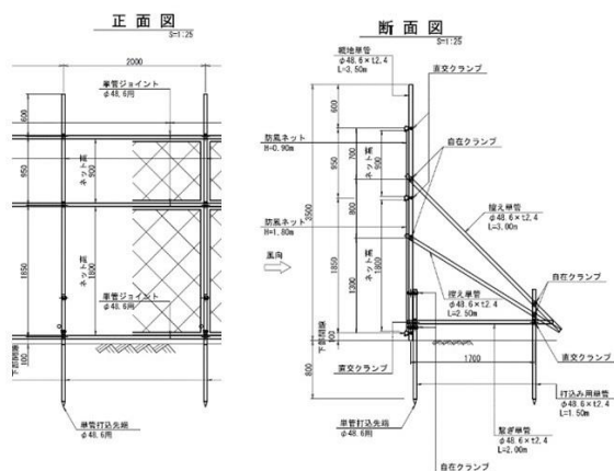
図 80 ネット柵工の一般図の例 (高さ 2.7m の場合)
