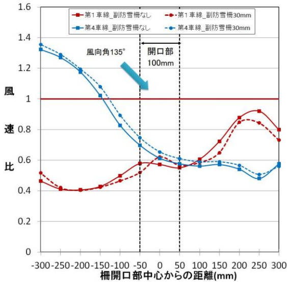
図 41 道路上の縦断方向における風速比 (風向角 135°、開口幅 100mm)
