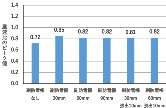
図 64 風向角 67.5°のピーク値 (開口幅 100mm、第4車線)
