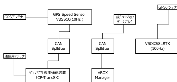
図-1 機器構成
