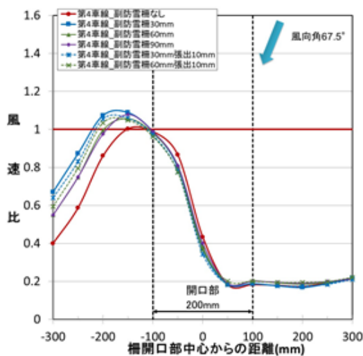
図 72 道路上の縦断方向における風速比 (実験条件 20、風向角 67.5°、開口幅 200mm、第 4 車線)
