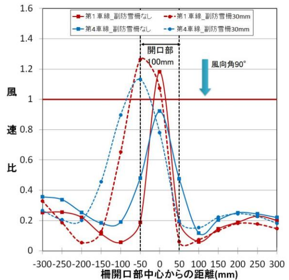
図 39 道路上の縦断方向における風速比 (風向角 90°、開口幅 100mm)
