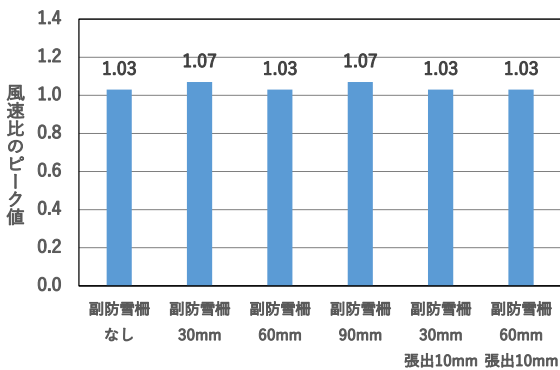
図 63 風向角 67.5°のピーク値 (開口幅 100mm、第1車線)
