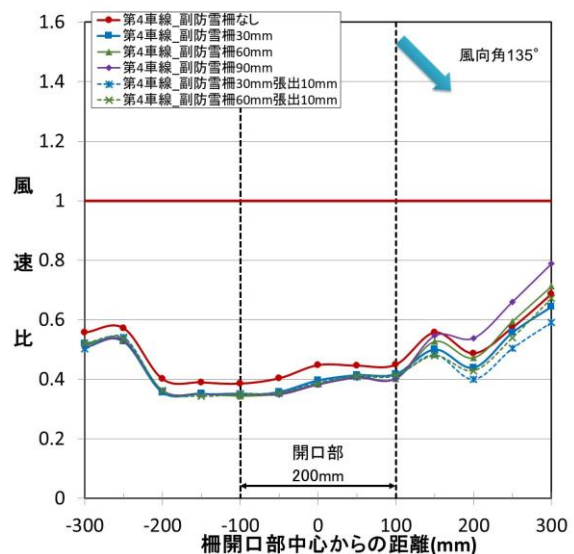
図 54 道路上の縦断方向における風速比 (実験条件8、風向角 135°、開口幅 200mm、第4車線)
