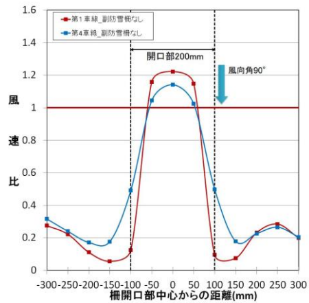
図 31 道路上の縦断方向における風速比
