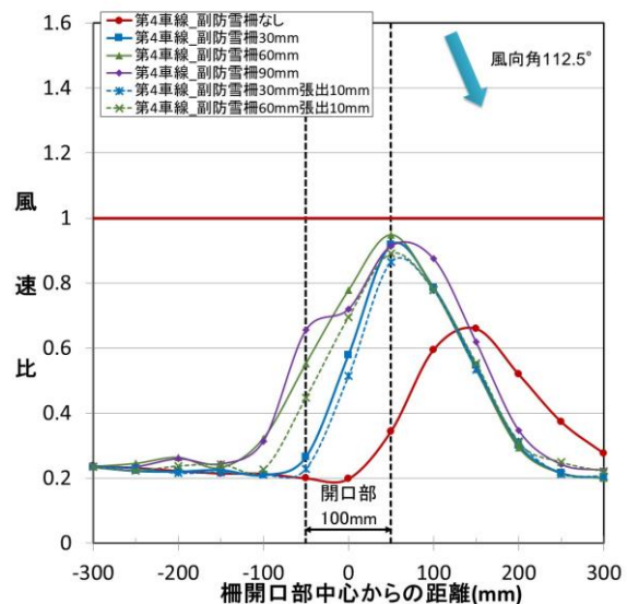
図 62 道路上の縦断方向における風速比 (実験条件 14、風向角 112.5°、開口幅 100mm、第 4 車線)
