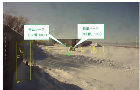
写真-33 実験⑦車両検出状況
