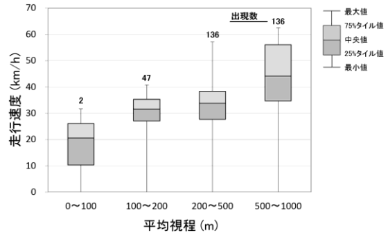
図 11 平均視程と走行速度
