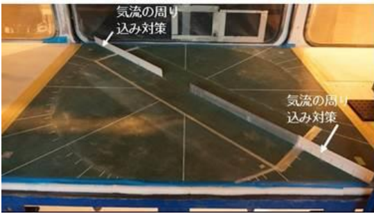
図 50 気流の周り込み対策をした防雪柵模型
