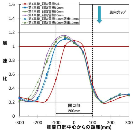
図 49 道路上の縦断方向における風速比 (実験条件 4、風向角 90°、開口幅 200mm、第 4 車線)
