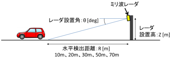
図-17 実験①概略図
