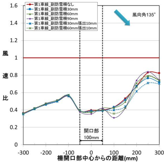
図 51 道路上の縦断方向における風速比 (実験条件5、風向角 135°、開口幅 100mm、第1車線)
