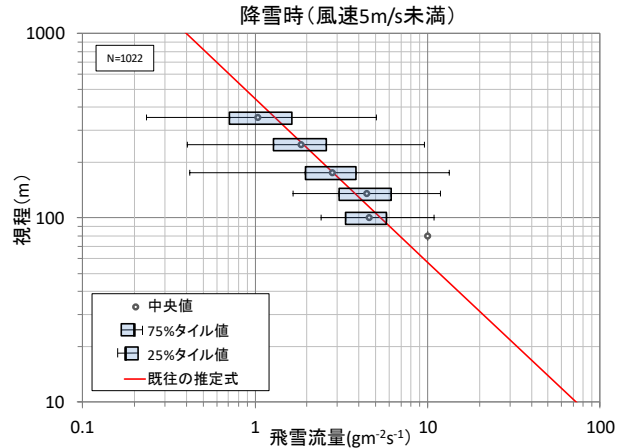
図 18 飛雪流量と視程の関係 (風速 5m/s 未満)
