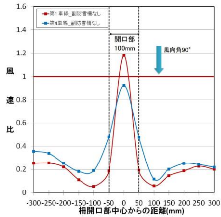
図 30 道路上の縦断方向における風速比（風向角 90^\circ 、開口幅 100mm）
