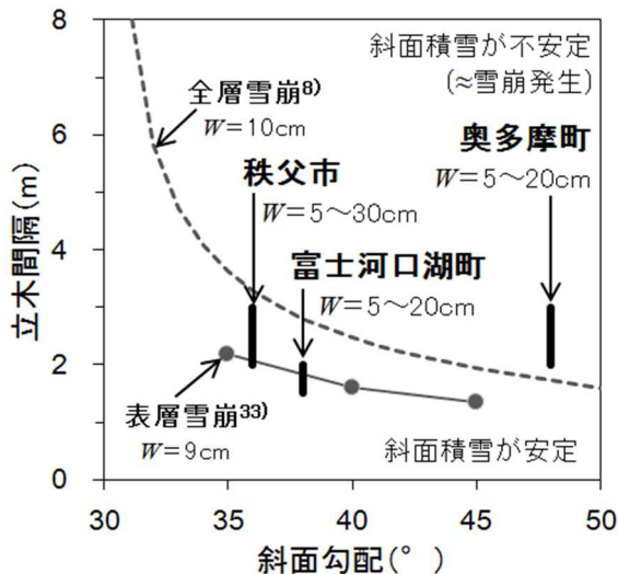
図-17 雪崩発生箇所の立木間隔と斜面勾配、雪崩発生防止に必要な立木間隔と斜面勾配の関係 8),33) 、 W は胸高直径。
