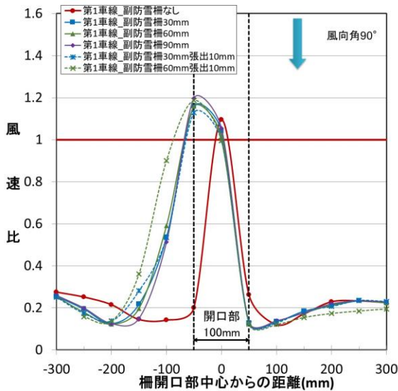
図 46 道路上の縦断方向における風速比 (実験条件 1、風向角 90°、開口幅 100mm、第 1 車線)
