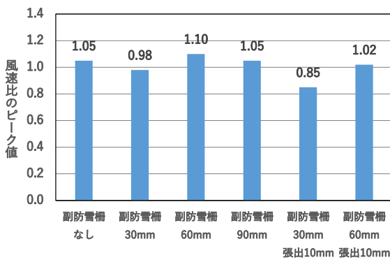
図 59 風向角 112.5° のピーク値 (開口幅 100mm、第 1 車線)
