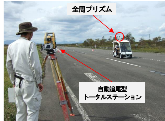
写真-10 TSによる計測状況(直線部)
