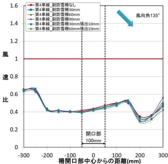
図 52 道路上の縦断方向における風速比 (実験条件6、風向角 135°、開口幅 100mm、第4車線)
