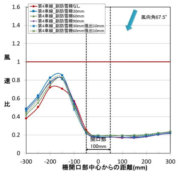
図 66 道路上の縦断方向における風速比 (実験条件 18、風向角 67.5°、開口幅 100mm、第4車線)
