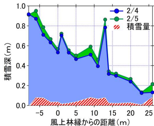
図 85 雄信内防雪林が 1 イベントで捕捉した飛雪量
