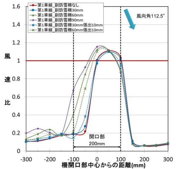
図 69 道路上の縦断方向における風速比 (実験条件 15、風向角 112.5°、開口幅 200mm、第1車線)
