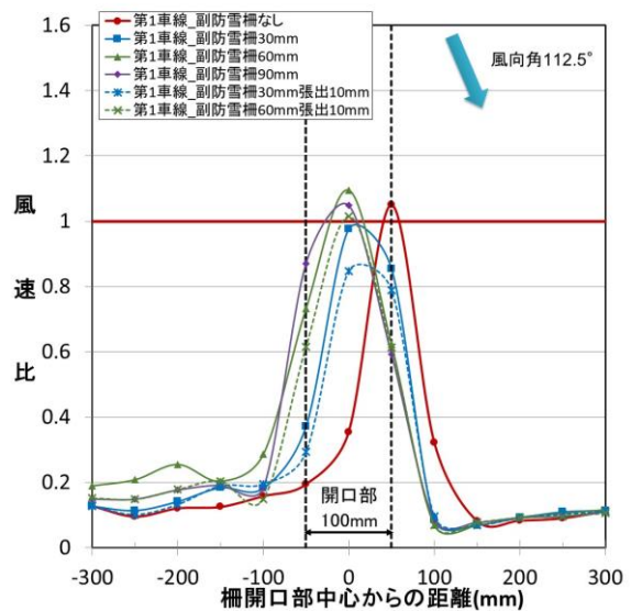
図 61 道路上の縦断方向における風速比 (実験条件 13、風向角 112.5°、開口幅 100mm、第 1 車線)
