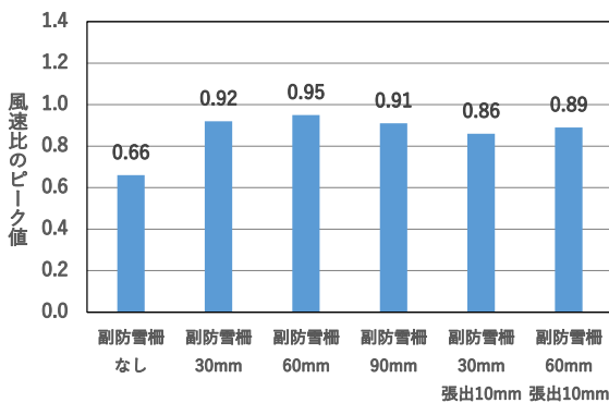
図 60 風向角 112.5° のピーク値 (開口幅 100mm、第 4 車線)
