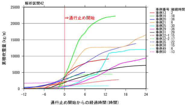
図28 通行止め前後における累積吹雪量の一例
