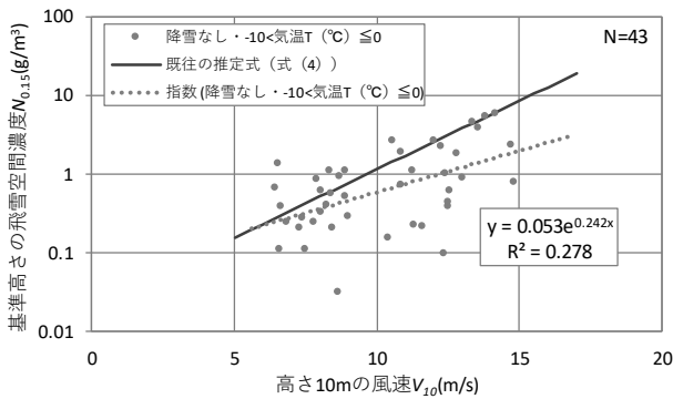
図 27 基準高さの飛雪空間密度と高さ 10m の風速 (降雪なし)
