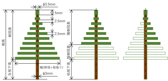
a) 枯れ上り無し模型 b) 枯れ上り模型(下枝) c) 枯れ上り模型(下枝・奥側)
