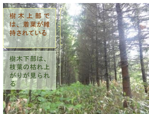
図1 防雪林内の下枝の枯れ上がり状況
