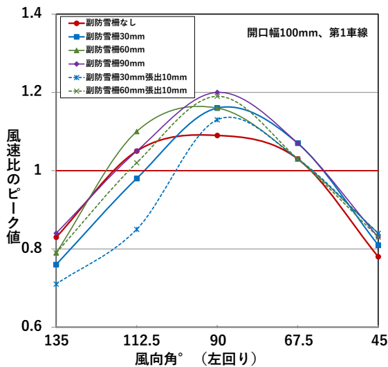
図 67 風向角と風速比のピーク値 (開口幅 100mm、第1車線)
