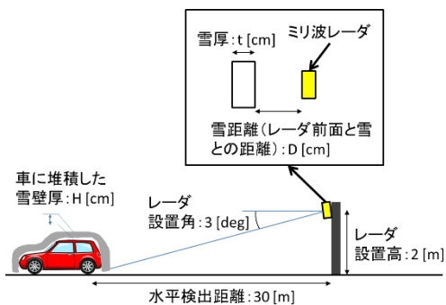
図-20 実験④概略図
