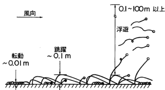
図6 吹雪の運動形態(転動・跳躍・浮遊) 16) より抜粋
