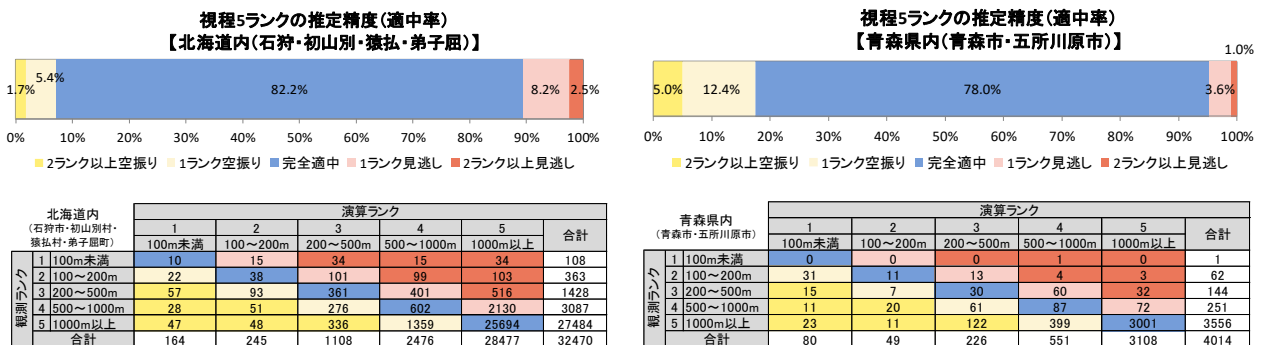
図 28 視程 5 ランクでの適中率
