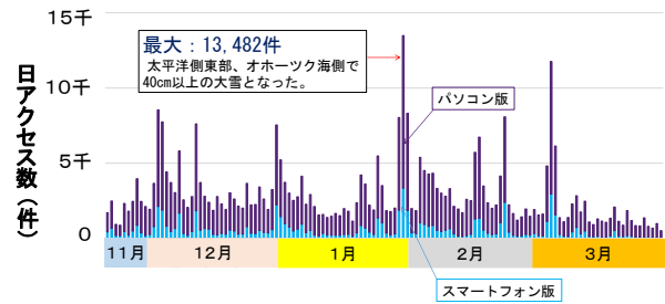
図 38 令和元年度「吹雪の視界情報」アクセス数
