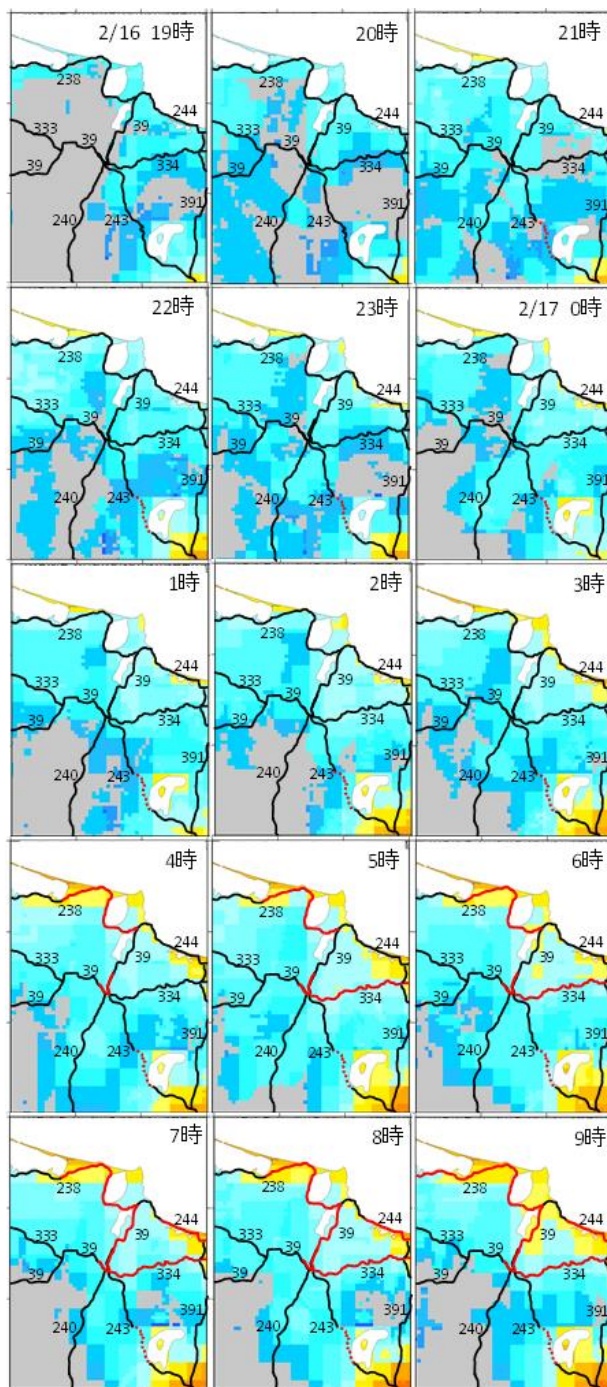
図21 通行止め実施有無と時間吹雪量の関係 (2014年2月16日19時～17日9時)
