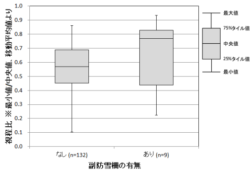
図 36 副防雪柵の有無と視程比の関係
