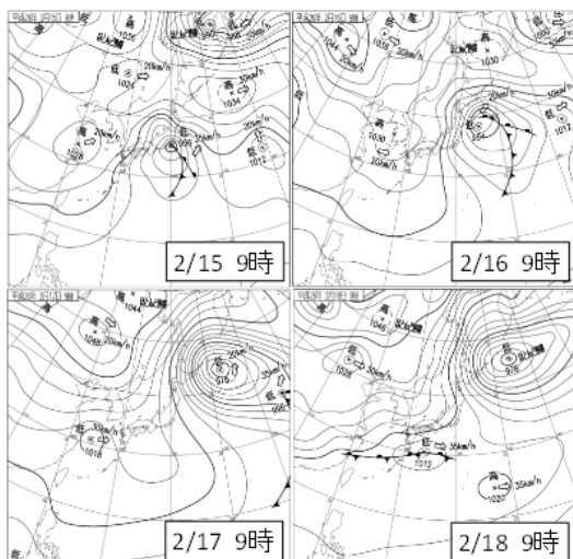
図18 2014年2月15日～18日の9時の地上天気図
