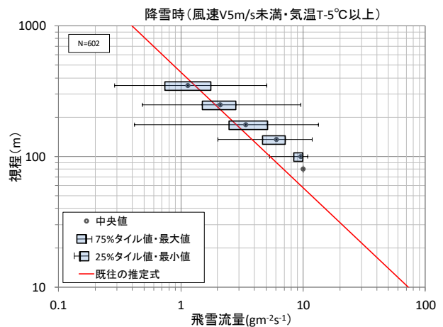
図 20 飛雪流量と視程の関係 (風速 5m/s 未満)
