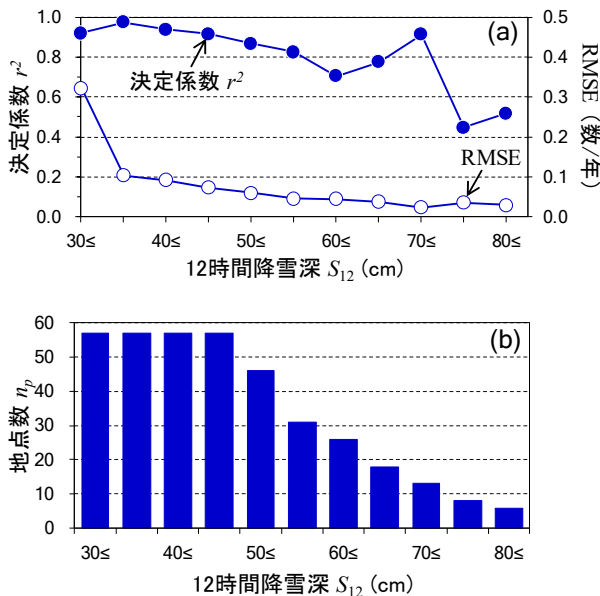
図-25 12 時間降雪深 S_{12} の 5cm ごと (a) 決定係数と RMSE、(b) 観測地点数。
