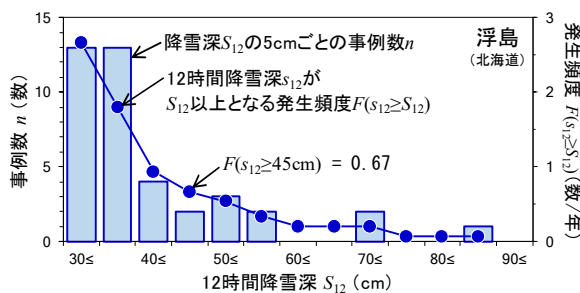
図-21 12 時間降雪深 S_{12} の 5cm ごとの事例数 n と発生頻度 F(S_{12} \geq S_{12}) の算出例。
