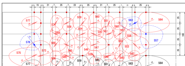
図 50 一般国道 40 号線沿い雄信内防雪林の調査結果から製作した植栽配置構成図
