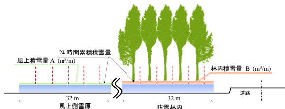
図 86 防雪林だけで捕捉した飛雪量（吹きだまり量） 捕捉した飛雪量＝林内積雪量 A－風上積雪量 B（単位： m³/m）
