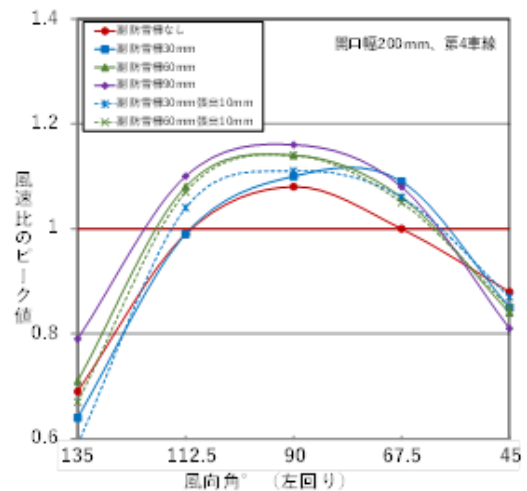
図 74 風向角と風速比のピーク値 (開口幅 200mm、第 4 車線)
