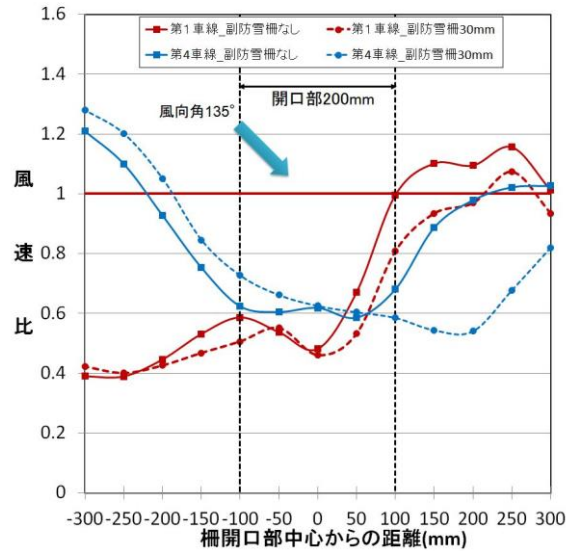
図 42 道路上の縦断方向における風速比 (風向角 135°、開口幅 200mm)
