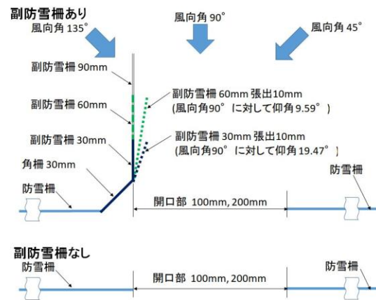
図 45 副防雪柵の設置状況
