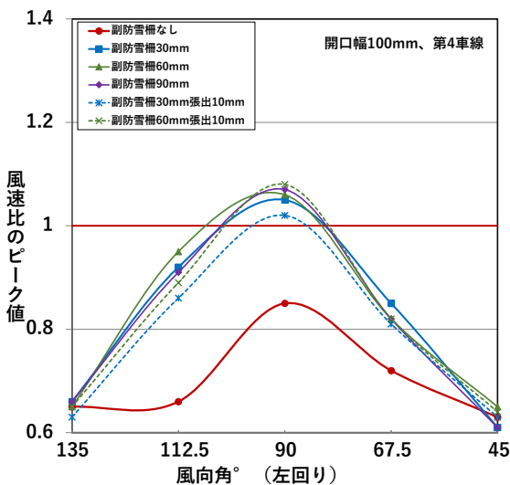
図 68 風向角と風速比のピーク値 (開口幅 100mm、第4車線)
