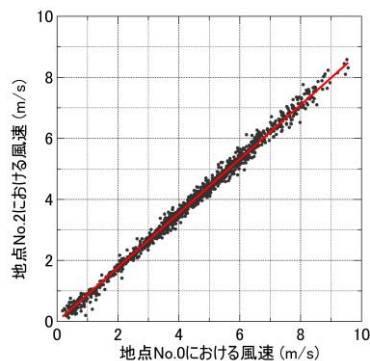
図 19 林風上の基準点 No.0 と林縁 No.2 地点における風速の比較（高さ:3m）
