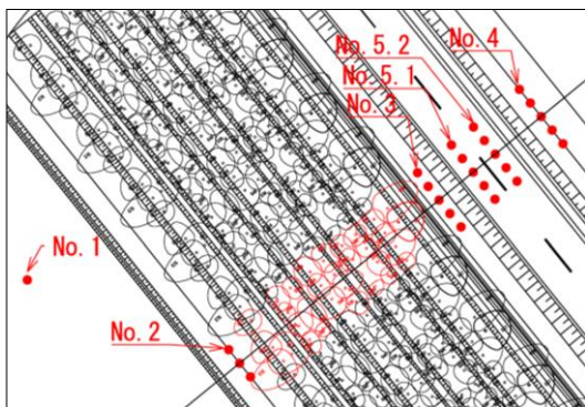
図 52 風速計測点位置図
