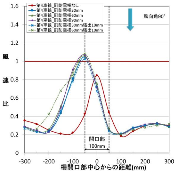
図 47 道路上の縦断方向における風速比 (実験条件 2、風向角 90°、開口幅 100mm、第 4 車線)
