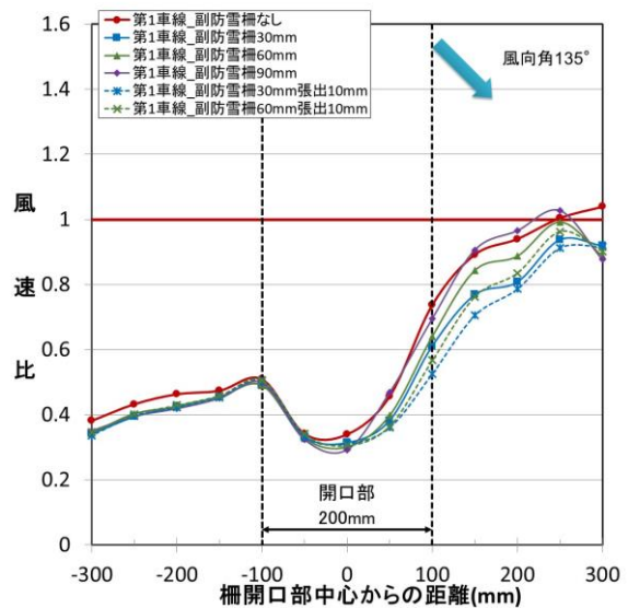
図 53 道路上の縦断方向における風速比 (実験条件7、風向角 135°、開口幅 200mm、第1車線)
