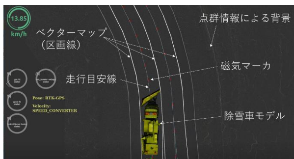
図-14 ガイダンス画面例（2D ビュー）
