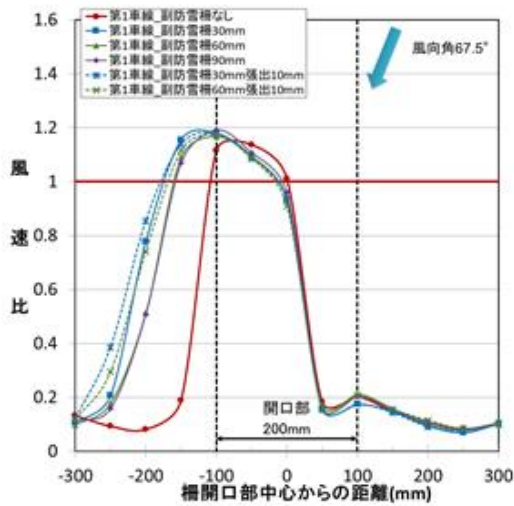
図 71 道路上の縦断方向における風速比 (実験条件 19、風向角 67.5°、開口幅 200mm、第 1 車線)
