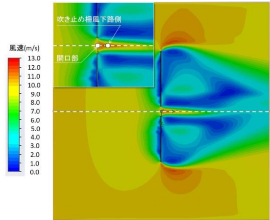
図 21 吹き止め柵まわりを再現した風速分布
