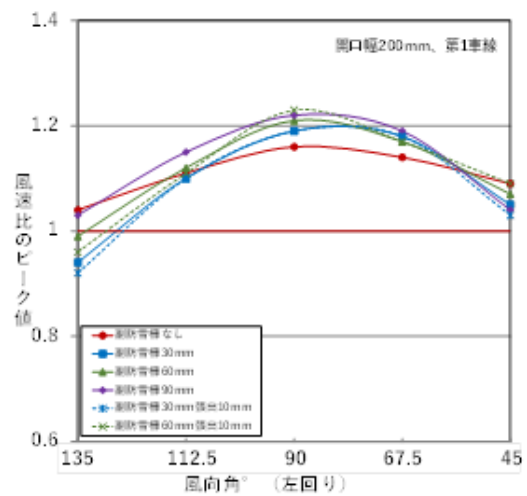
図 73 風向角と風速比のピーク値 (開口幅 200mm、第 1 車線)
