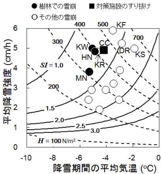
図-5 各気象観測地点における降雪期間のうち降雪強度が最大となった連続する12時間の平均気温と平均降雪強度の関係。斜面積雪の安定度 SI (実線) と硬度 H (破線) は、平均気温と平均降雪強度を用いた計算値。平均気温は図-3 の標高との回帰式から求めた標高1100mの値。地点の略記号は図-1に同じ。
