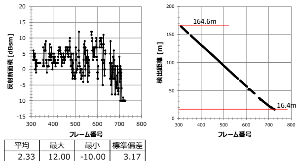
図-30 実験⑧車両検出結果 (降雪無し)
