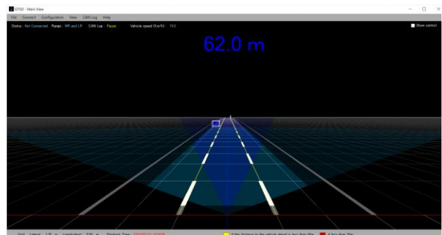
図-44 ガイダンス画面例 (注意 60m 警告 30m 時_通常)
