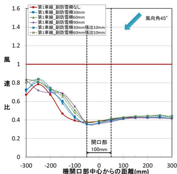
図 55 道路上の縦断方向における風速比 (実験条件 9、風向角 45°、開口幅 100mm、第 1 車線)
