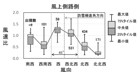
図 18 風下路側における風向別の風速比
