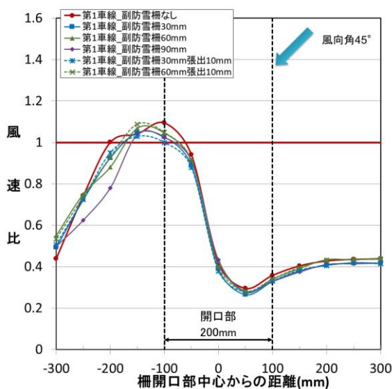
図 57 道路上の縦断方向における風速比 (実験条件 11、風向角 45°、開口幅 200mm、第 1 車線)
