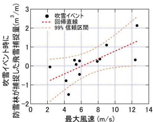
図 87 防雪林が捕捉した飛雪捕捉量と最大風速
