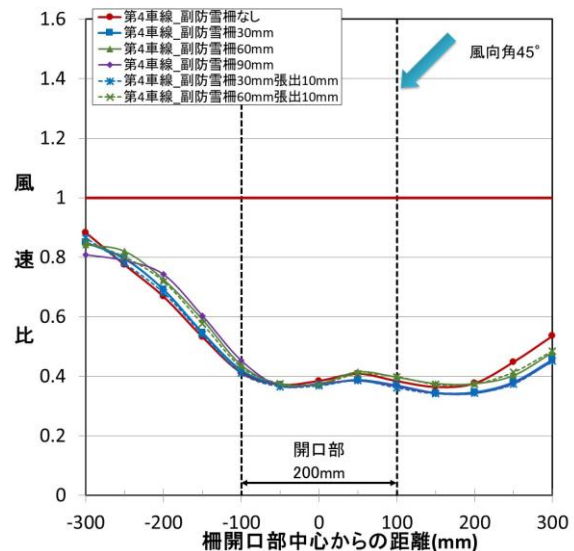
図 58 道路上の縦断方向における風速比 (実験条件 12、風向角 45°、開口幅 200mm、第 4 車線)
