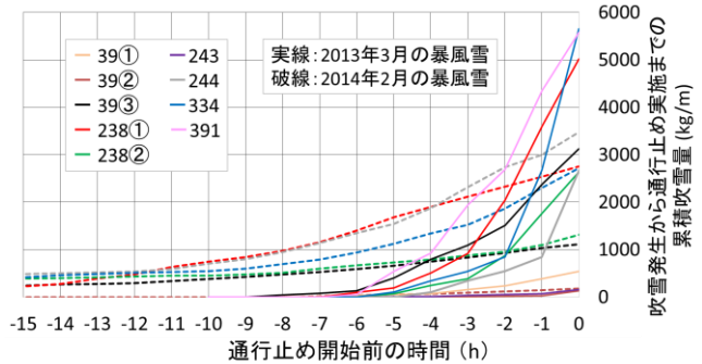
図 24 通行止め開始までの累積吹雪量の変化
