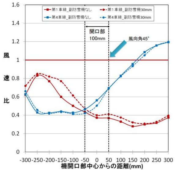
図 43 道路上の縦断方向における風速比 (風向角 45°、開口幅 100mm)
