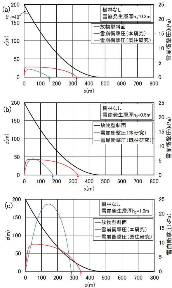
図-28 斜面高さ z_0 が200m、雪崩発生区の傾斜角 \theta_0 が40°の放物型斜面(黒)、雪崩の衝撃圧 P (青：既往研究、赤：本研究)、雪崩到達点(青矢印：既往研究、赤矢印：本研究)
