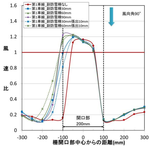
図 48 道路上の縦断方向における風速比 (実験条件 3、風向角 90°、開口幅 200mm、第 1 車線)
