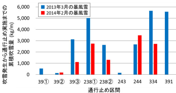
図 23 吹雪発生から通行止め実施までの累積吹雪量
