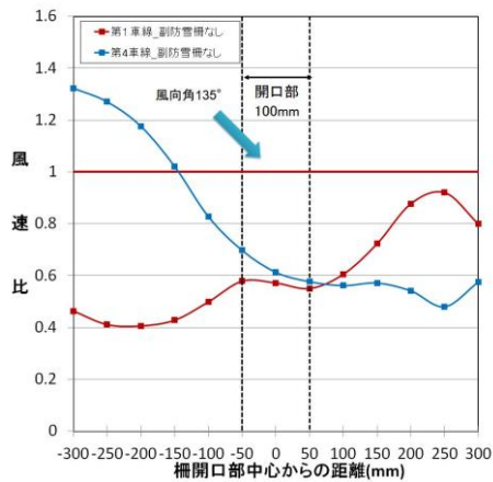
図 32 道路上の縦断方向における風速比（風向角 135^\circ 、開口幅 100mm）
