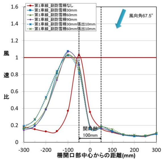
図 65 道路上の縦断方向における風速比 (実験条件 17、風向角 67.5°、開口幅 100mm、第1車線)
