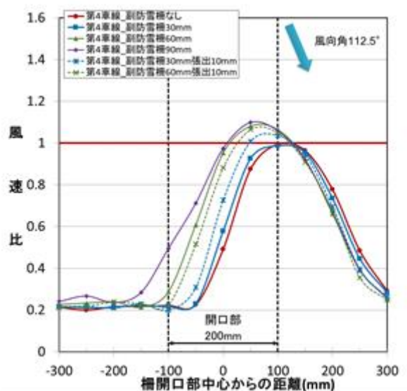
図 70 道路上の縦断方向における風速比 (実験条件 20、風向角 67.5°、開口幅 200mm、第4車線)
