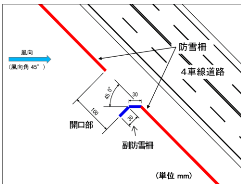
図 37 副防雪柵配置例 (風向角 45°、開口幅 100mm、副防雪柵 30mm)
