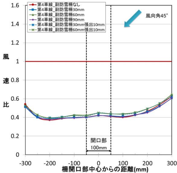
図 56 道路上の縦断方向における風速比 (実験条件 10、風向角 45°、開口幅 100mm、第 4 車線)
