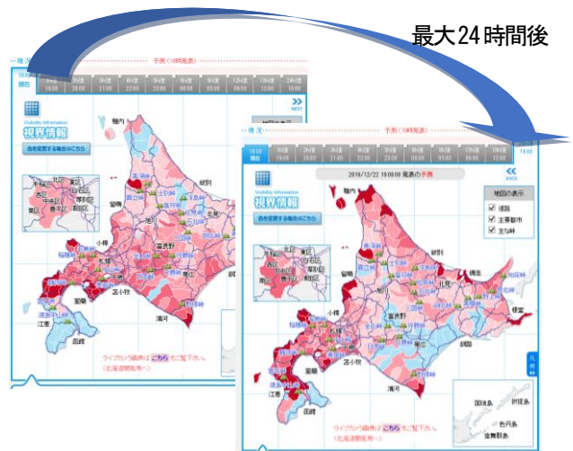
図32 吹雪の視界情報のエリアと予測時間 (平成28年12月22日18時発表)
