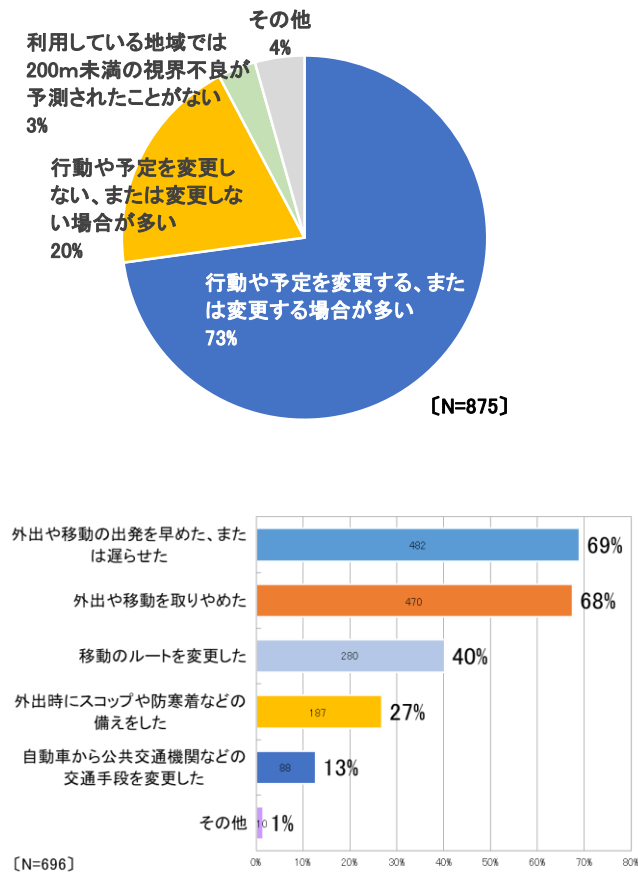
図 37 「吹雪の視界情報」アンケート回答結果 視界不良予測時の行動変更について
