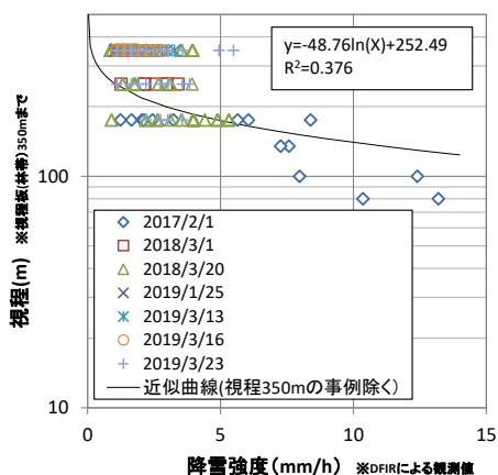
図 17 降雪強度と視程の関係（風速 5m/s 未満）
