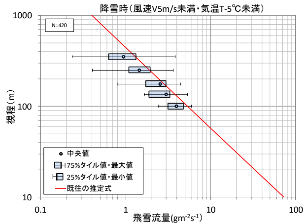
図 19 飛雪流量と視程の関係 (風速 5m/s 未満)
