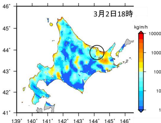
図19 3月2日18時における時間吹雪量
