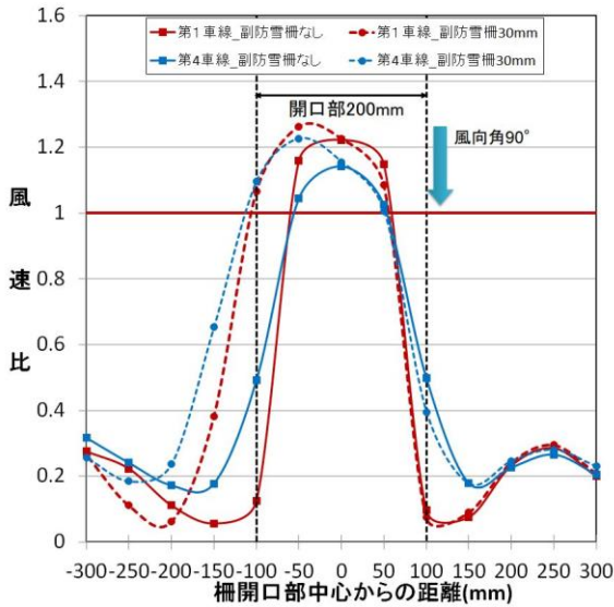
図 40 道路上の縦断方向における風速比 (風向角 90°、開口幅 200mm)
