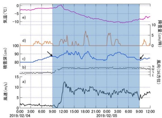
図 84 吹雪発生時の気象データ
