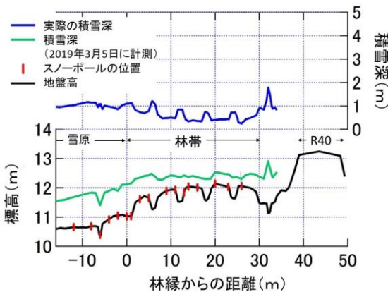
図 83 雄信内防雪林の積雪深（平成 31 年 3 月 5 日）と林縁からの距離
