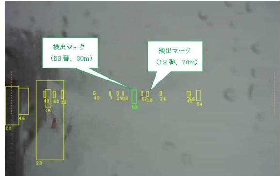
写真-32 実験⑥車両検出状況
