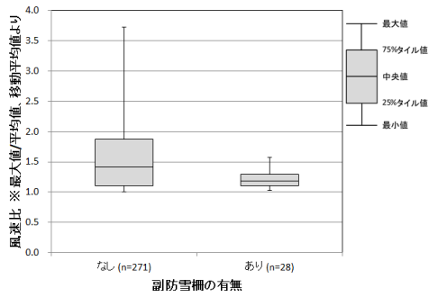
図 35 副防雪柵の有無と風速比の関係
