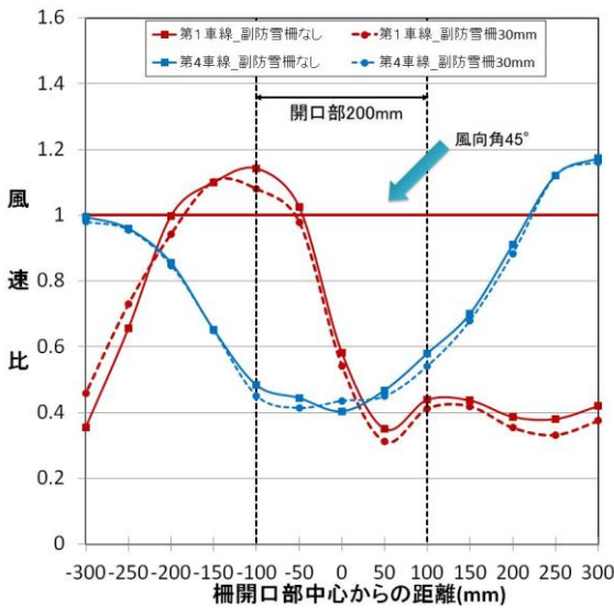
図 44 道路上の縦断方向における風速比 (風向角 45°、開口幅 200mm)
