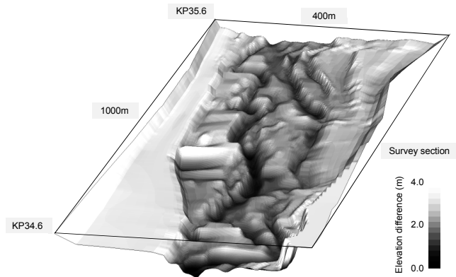
図-12 初期河床形状 (2011年11月測量)
