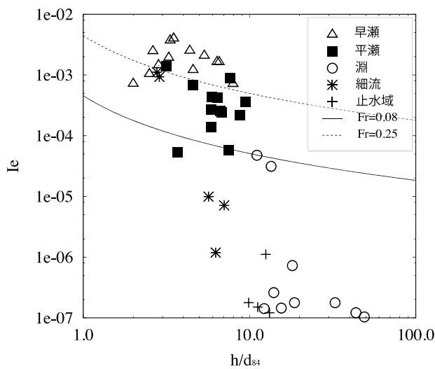
図-5 境界フルード数の推定
