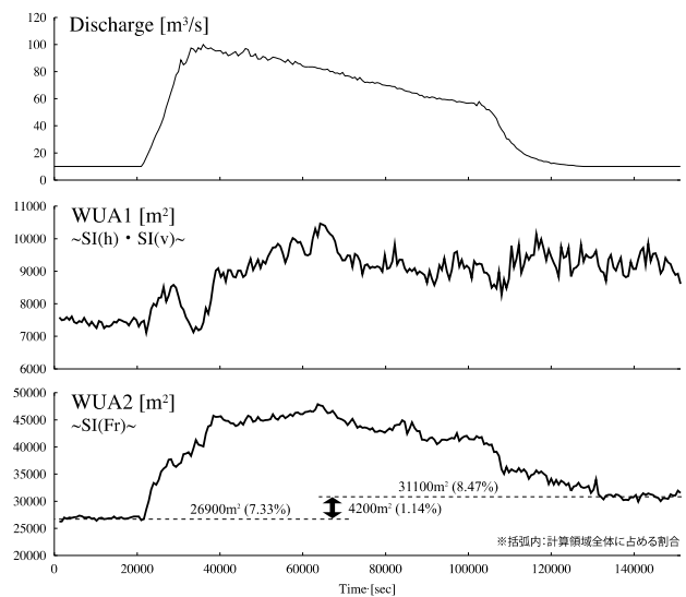
図-13 2012年ダム放流時の流量及びWUAの時間変化
