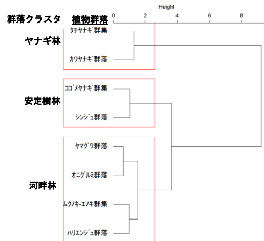
図-3 木本群落の群落クラスタ
