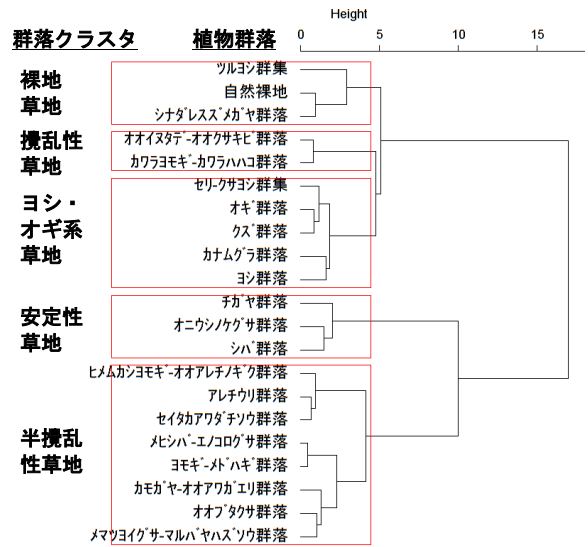
図-2 草本群落の群落クラスタ
