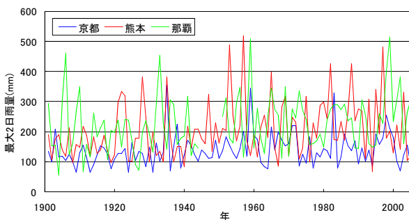
図5(2) 年最大2日雨量の経年変化
