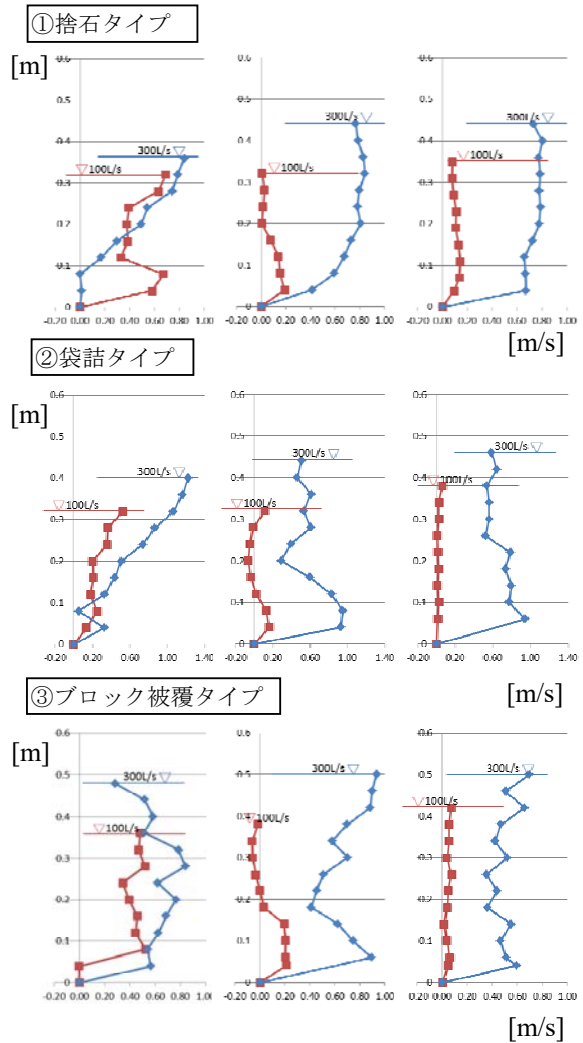
図4.2 河道中心における主流速鉛直分布 (左列:模型1m下流, 中列:2m下流, 右列:3m下流)
