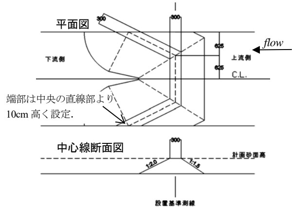
図4.1 大型模型の基本形状
