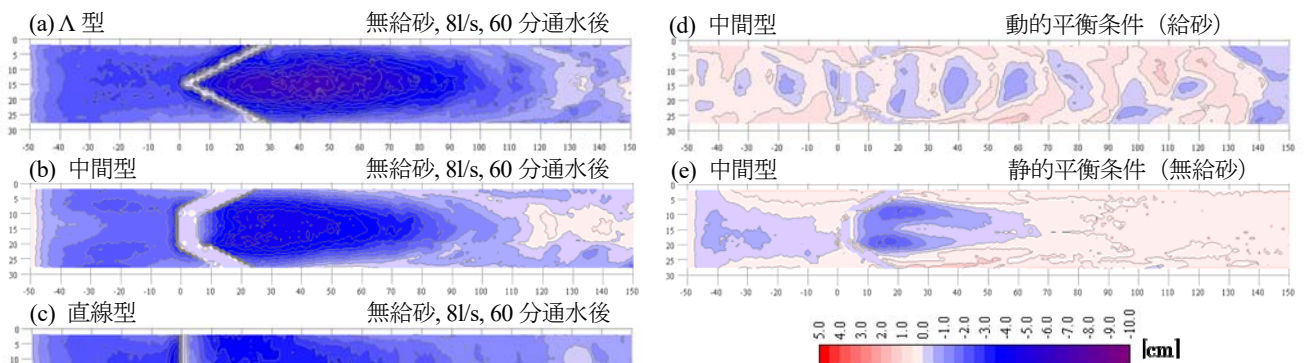
図3.1 通水後の河床変動量（模型形状及び洗掘条件の比較）
