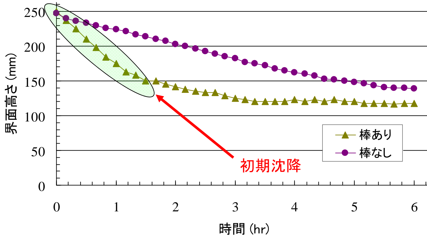
みずみち棒の有無による沈降曲線 ( \phi 18\text{mm} 、 0.84 \text{ min}^{-1} )
