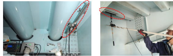
鋼床版の下側に超音波センサを設置し、調査している様子
