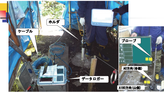
挿入式孔内傾斜計の測定状況
