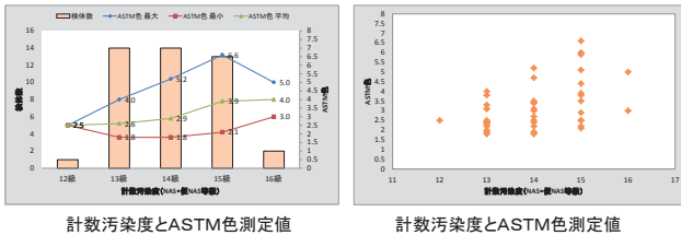
計数汚染度とASTM色測定値
