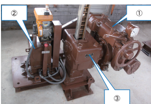
樋門開閉装置 (ラック式)
