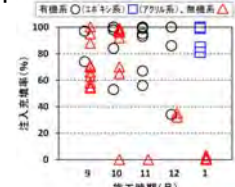
深さ10cmまでの注入材の注入充填率 (注入充填率が低いケースも多い)
