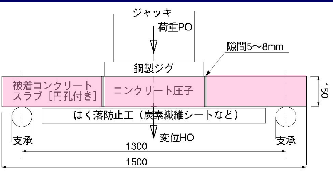
断面図
