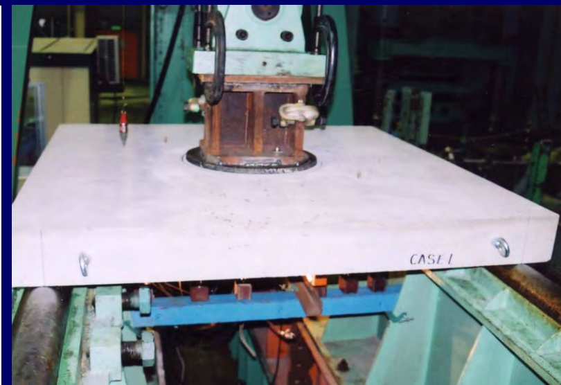
載荷状況
