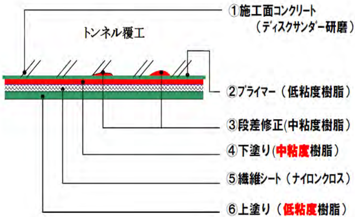
NAV工法の構造
