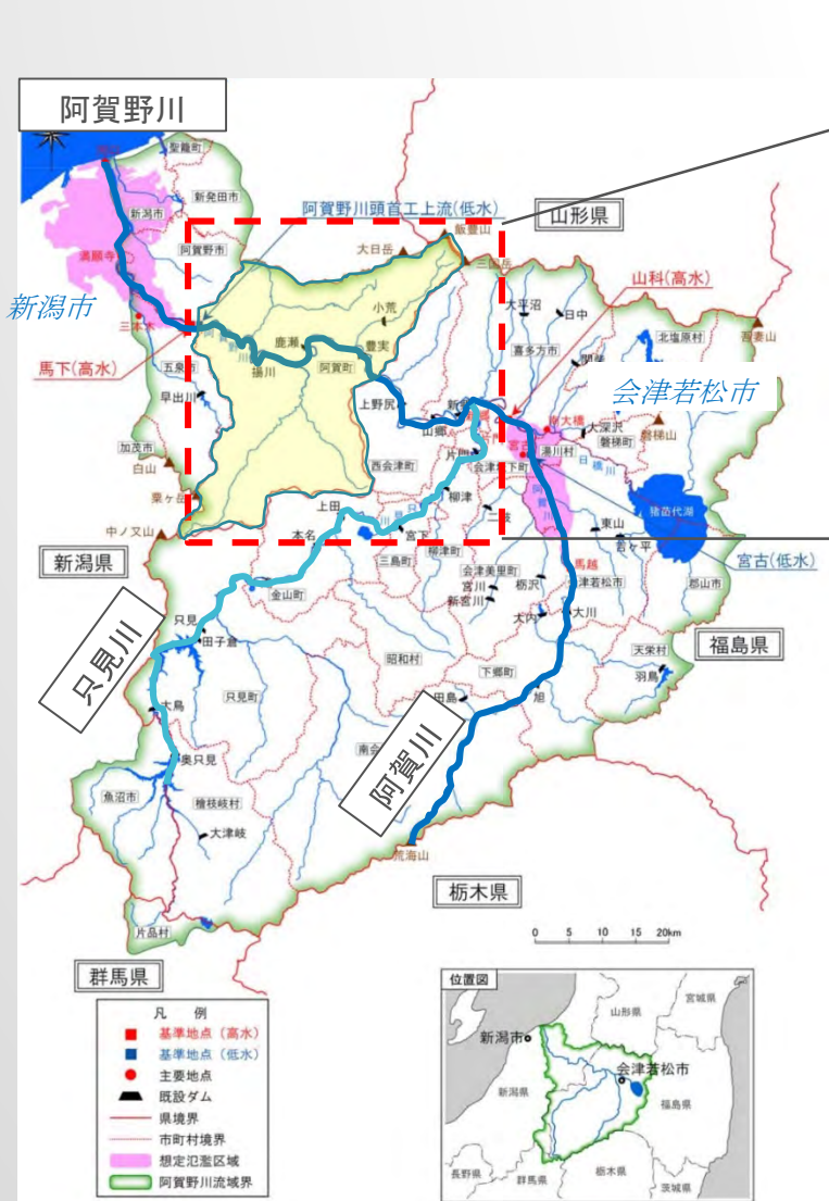
阿賀野川流域概要図 (流域面積約7,700km 2 )
