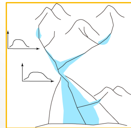
RRIモデル (一体的なアプローチ)
