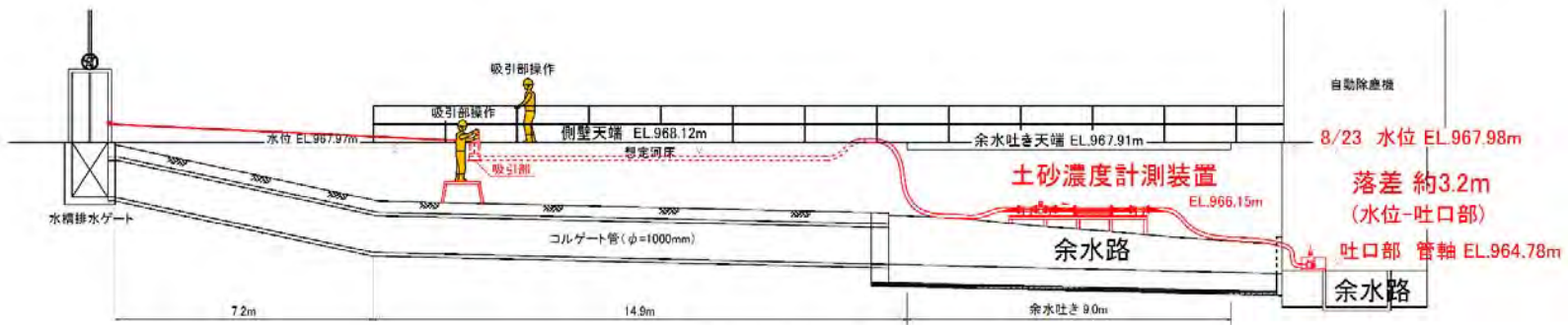
[ 縦断図 ]
