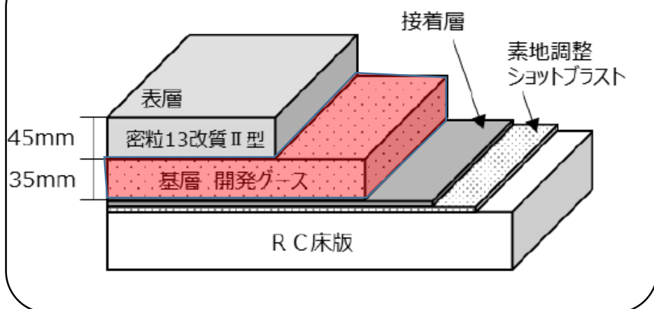
舗装構成（打換え後）
