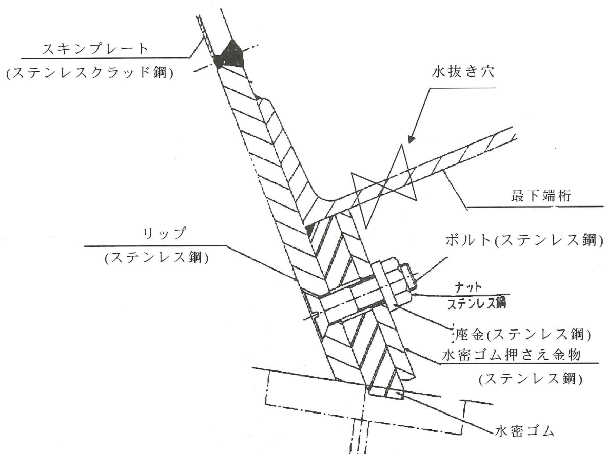
図解-3.7 扉体下部例（クレストラジアルゲートの場合）
