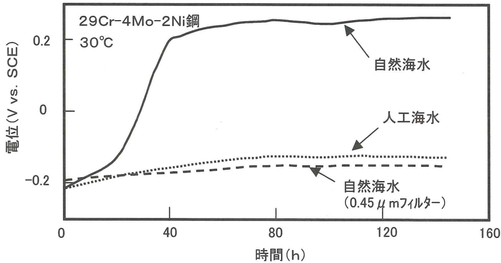
図解-2. 41 自然海水および人工海水中でのステンレス鋼の自然電位変化
