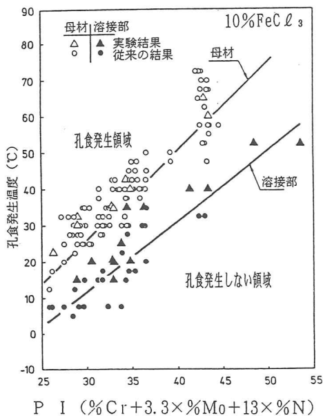
図解-2.16 P I と孔食発生温度との関係
