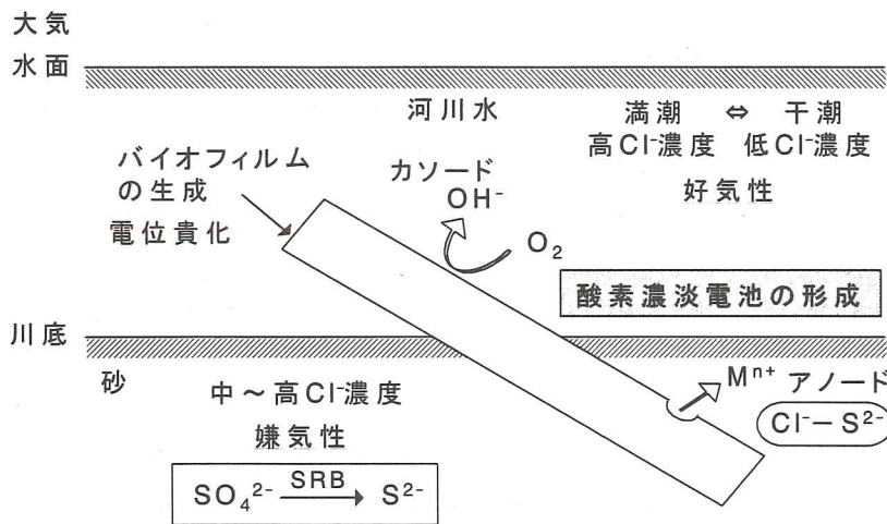
図解-2.47 一部が川底に埋まったステンレス構造物のマクロセル形成による孔食発生メカニズム
