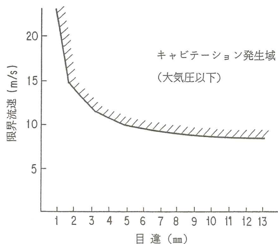
図解-3.12 余盛高さとキャビテーション発生限界流速
