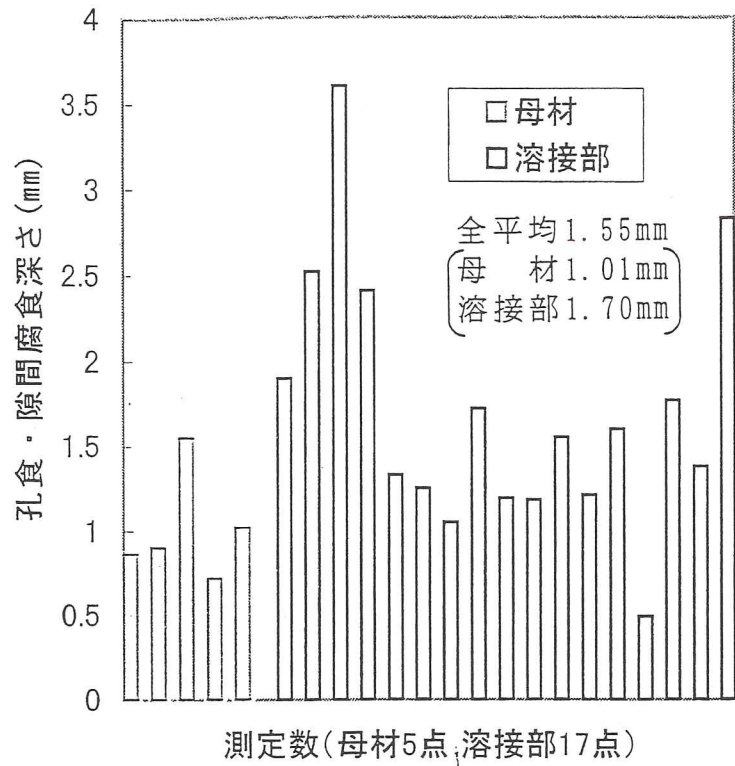
図解-2.45 板状大型試験片(土中設置試験片)〔下段〕・上面の孔食・すき間腐食測定結果 (SUS304, H9年7月10日~H9年10月29日)
