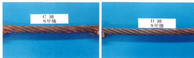
写真解-3.1 暴露試験結果（亜鉛めっき製ワイヤロープ・浸漬8年）
