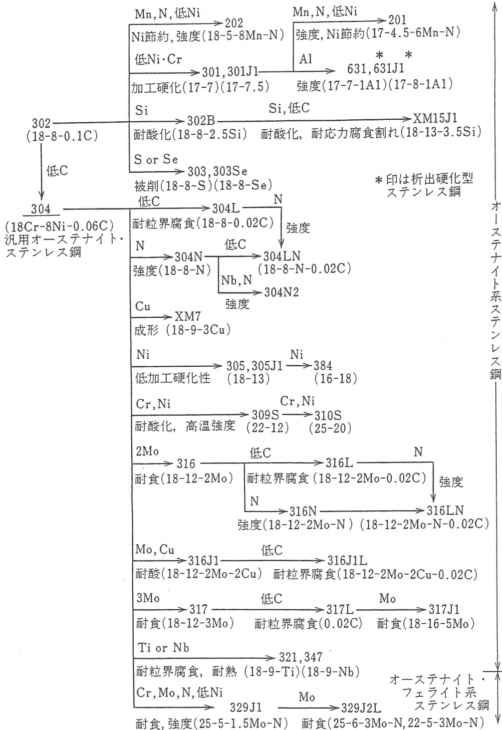
図解-2.2 Fe-Cr-Ni系ステンレス鋼の系統図
