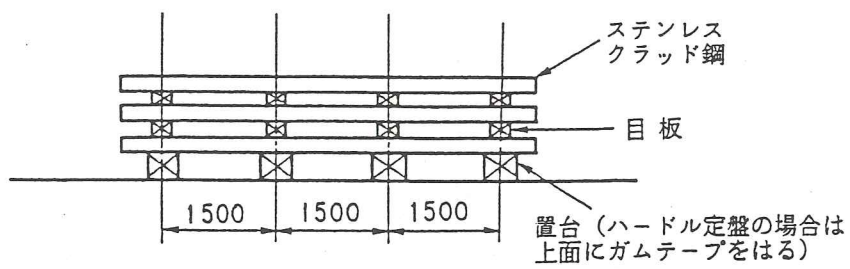
図解-4.2 ステンレスクラッド鋼の保管例
