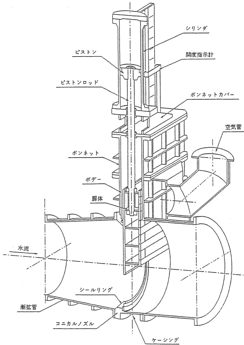
図解-5.6 バルブ例 (ジェットフローゲートの例)
