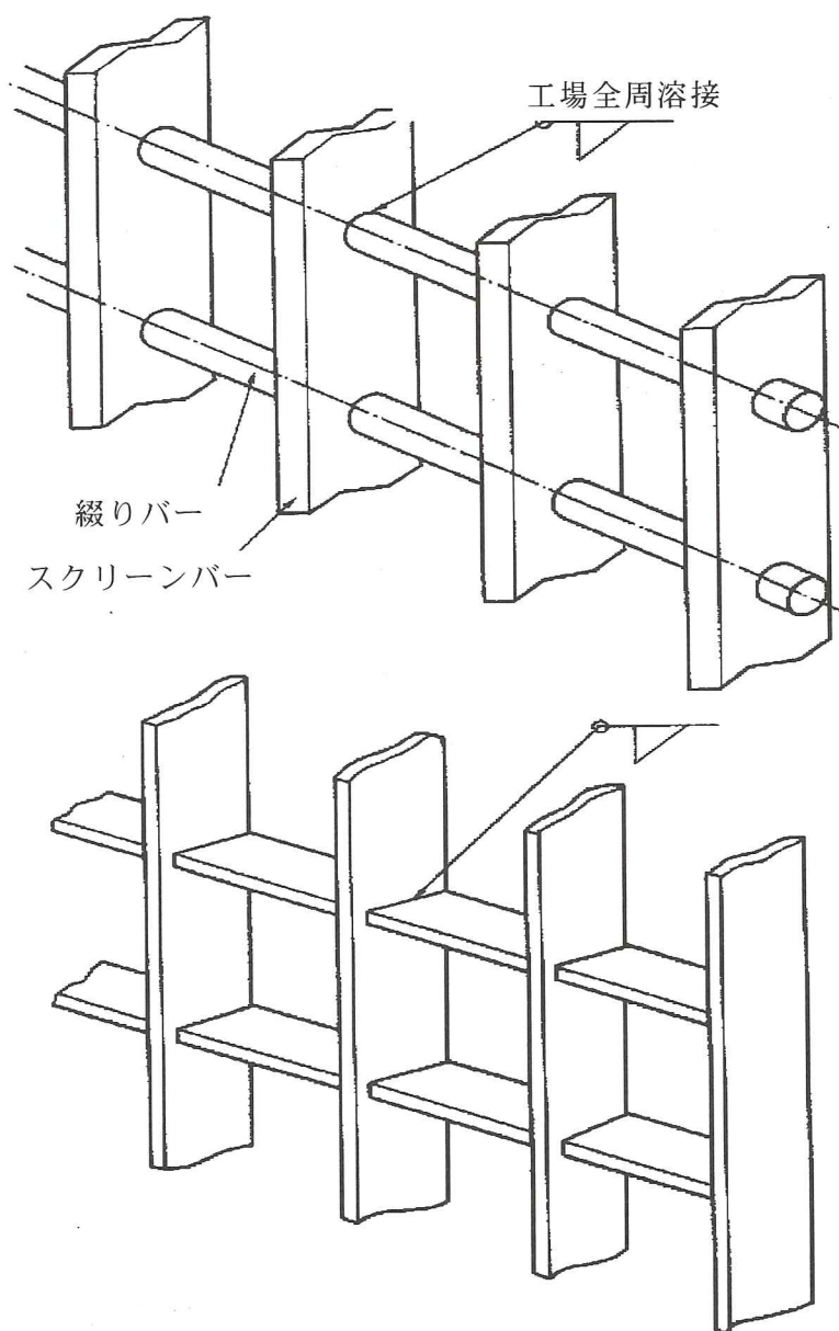
図解-3.15 スクリーンパネルの構造(上:綴りバー方式、下:溶接構造方式)
