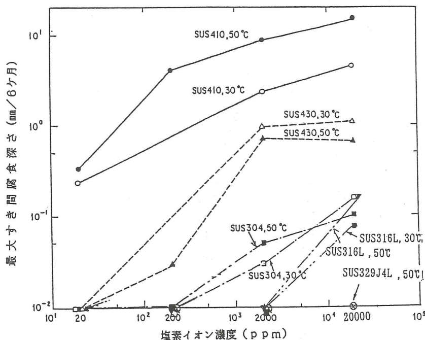
図解-3.17 すき間腐食深さに及ぼす塩素イオン濃度の影響
