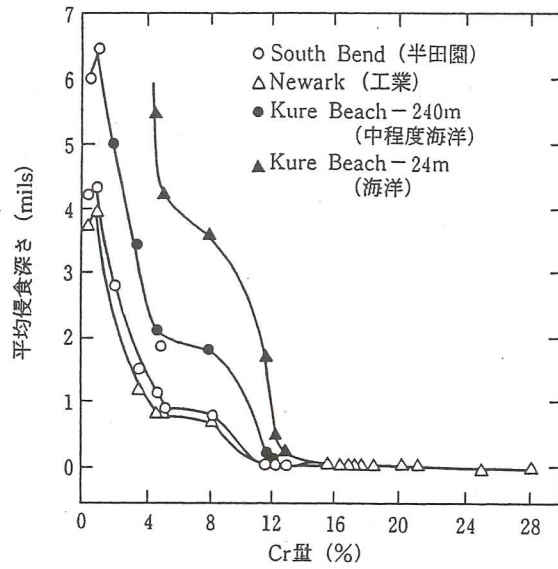
図解-2.3 Fe-Cr合金の8年間大気暴露結果 (ステンレス鋼便覧-第3版)
