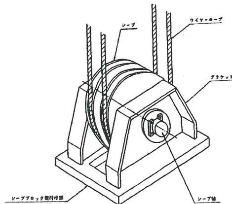
図解-5.2 扉体に付いたシーブブロックの例
