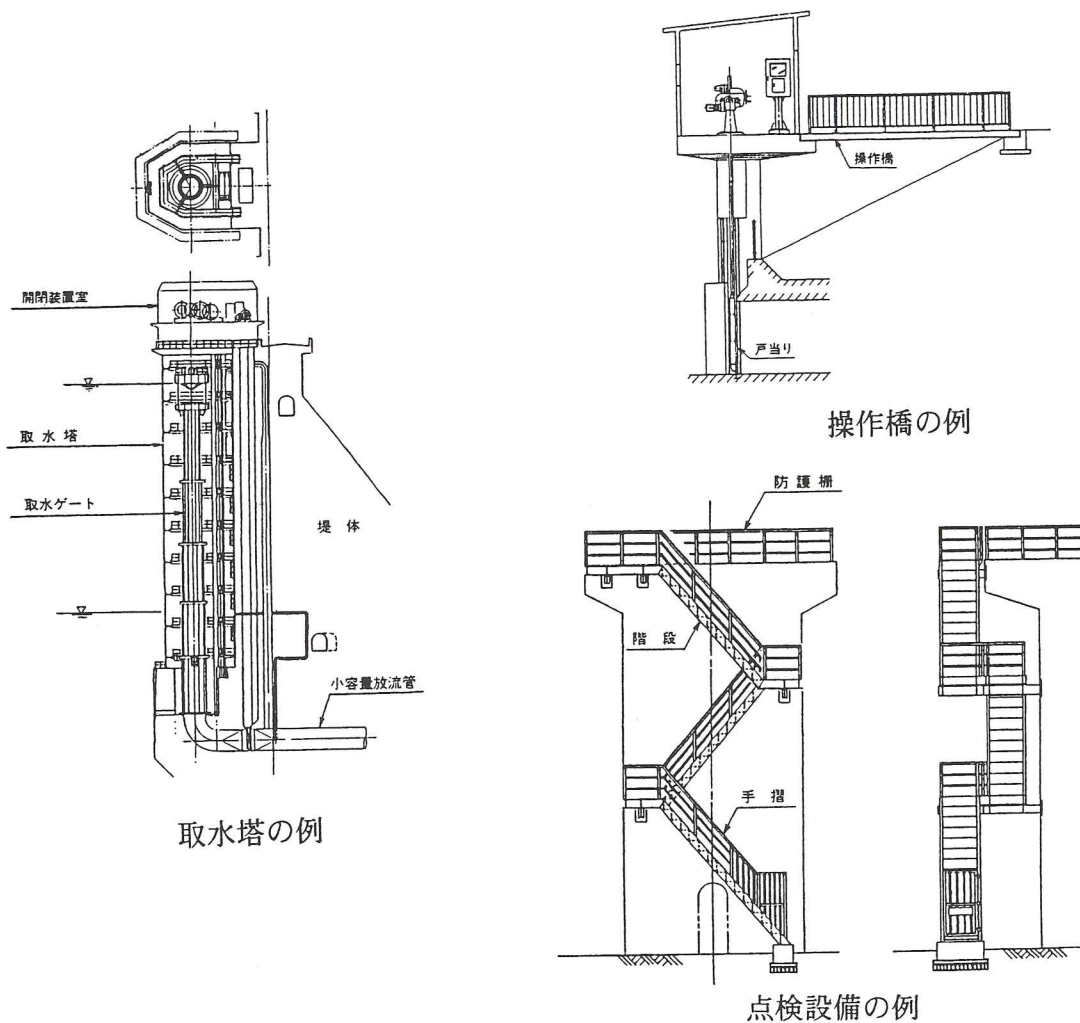
図解-5.7 その他の設備の例
