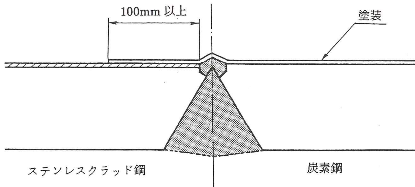
図解－5.9 異種金属接触部の塗装の塗り越し
