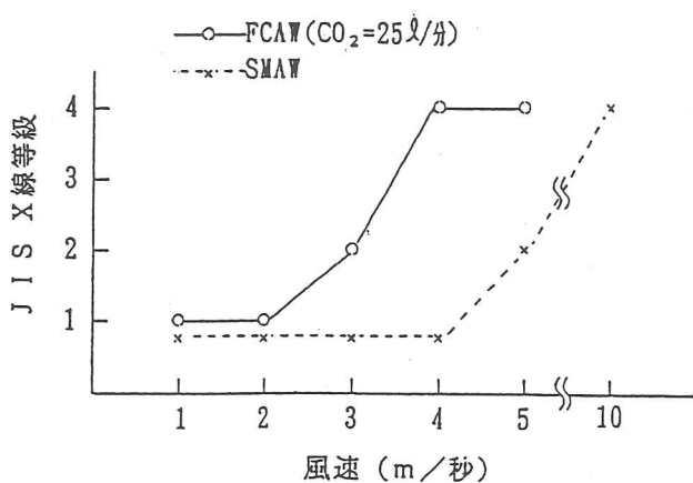
図解-4.8 溶接欠陥と風速の関係
