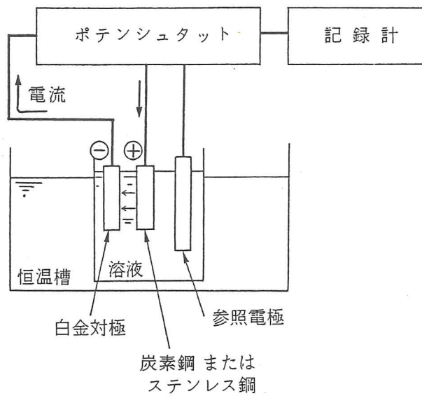
図解-2.27 分極測定の方法
