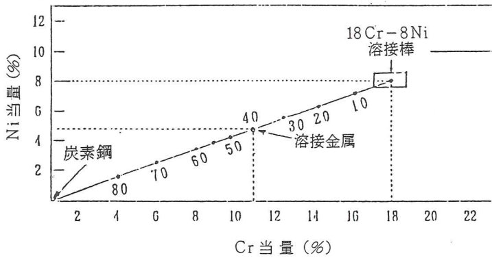
図解 4.13 炭素鋼とステンレス鋼の異材継手溶接
