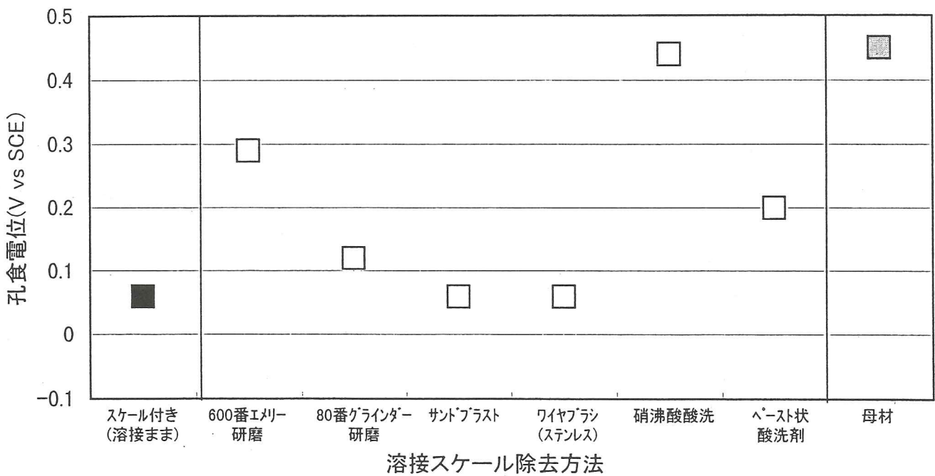
図解-2.40 耐孔食性に及ぼす溶接スケール除去方法の効果 [SUS329J4L, TIG共金溶接材, 人工海水, 80°C] (幸英昭: 材料と環境 40 (1991))
