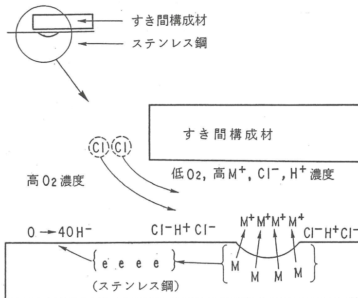
図解-2.32 すき間内部での腐食反応の概念図 (防食技術便覧)
