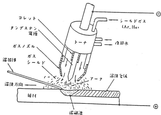
図解-4.6 各種溶接法の概略図
