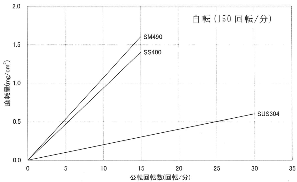
図解-2.10 鋼材の土砂摩擦
