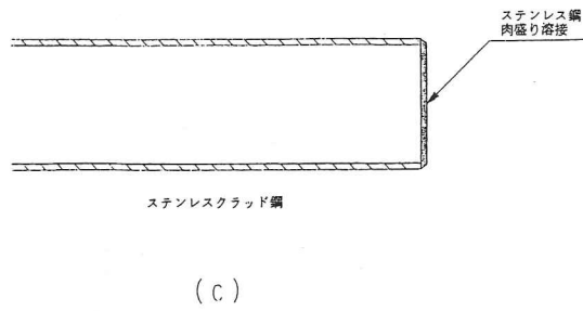
図解-5.12 ステンレスクラッド鋼の端面処理
