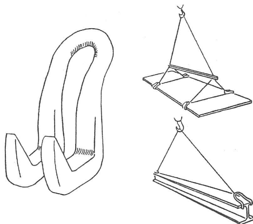
図解-4.15 ハッカーの例
