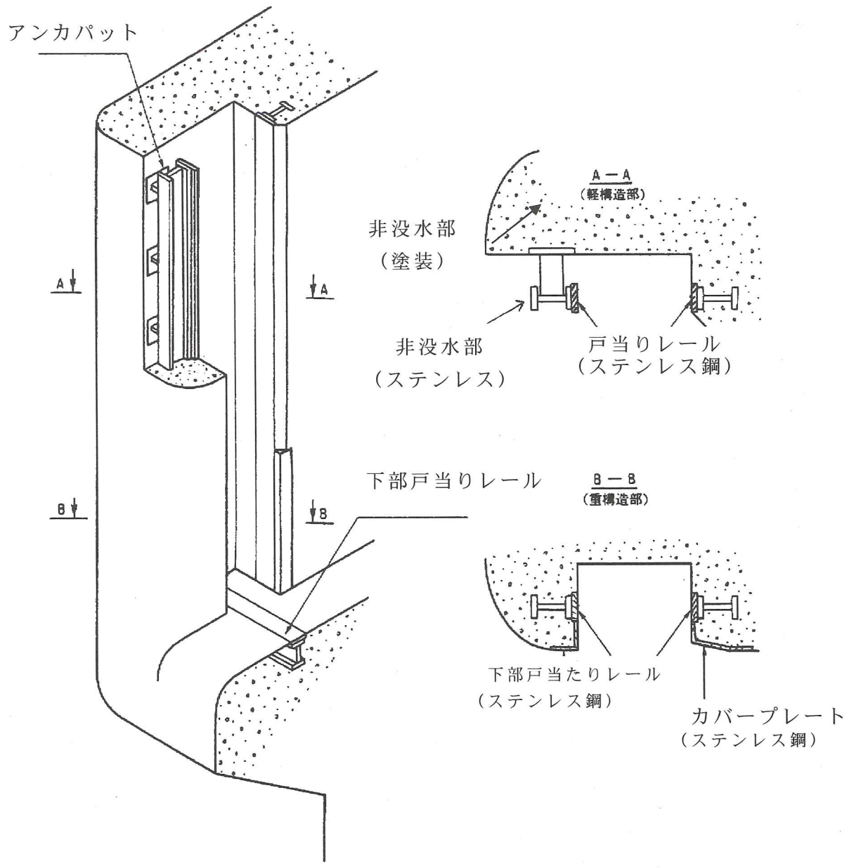
図解-3.9 戸当り例 (ローラゲートの場合)
