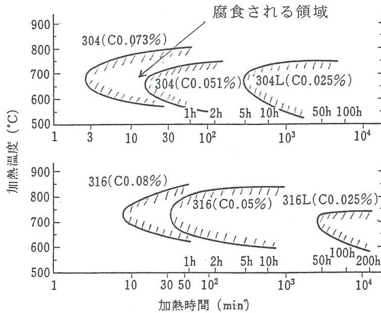
図解-2.18 SUS304・SUS316 系ステンレス鋼のT T S 曲線 (硫酸・硫酸銅試験) ハッチ部：鋭敏化域
