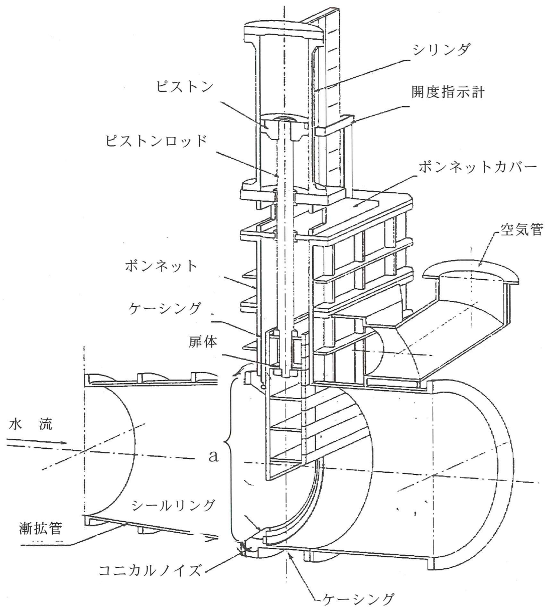
図解-3.13 バルブ (ジェットフローゲートの場合)
