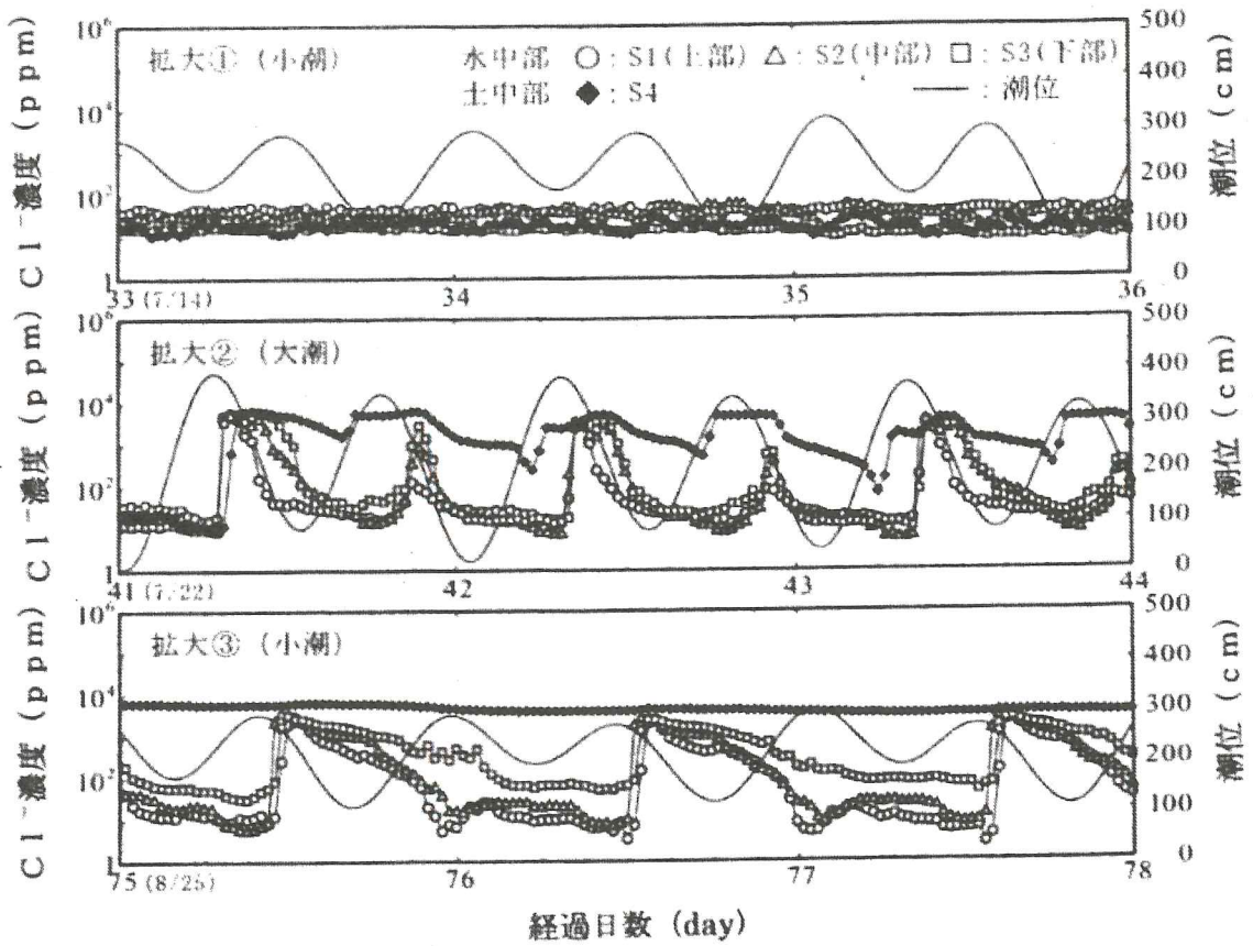
図解-3.19 河川の汽水域における潮位と水中、土中の塩化物イオン濃度の変化 (守屋ら、第50回材料と環境討論会、p.117, B-104, (2003))
