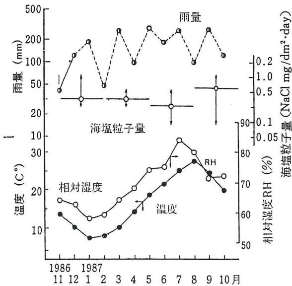
図解-2.13 駿河湾海洋技術総合研究施設における気象データ 御前崎測候所
