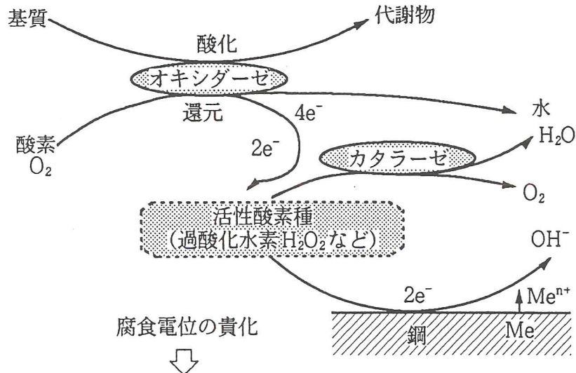
図解-2. 42 海水中におけるステンレス鋼の微生物腐食メカニズム (好気性バクテリアによる微生物腐食)
