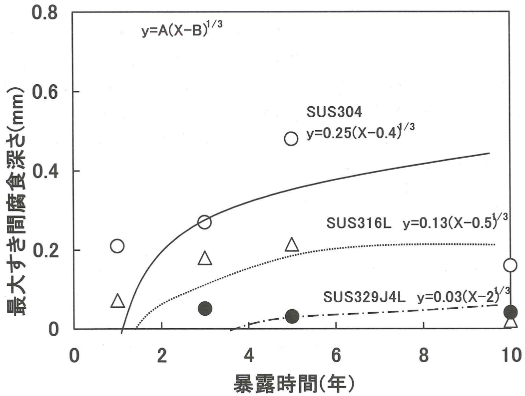
図解-2.33 最大すき間腐食深さ暴露時間依存性
