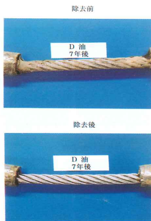
写真解-3.2 暴露試験結果 (ステンレス製ワイヤロープ・浸漬7年)
