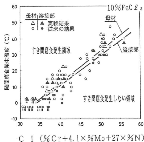
図解-2.17 C I とすき間腐食発生温度との関係
