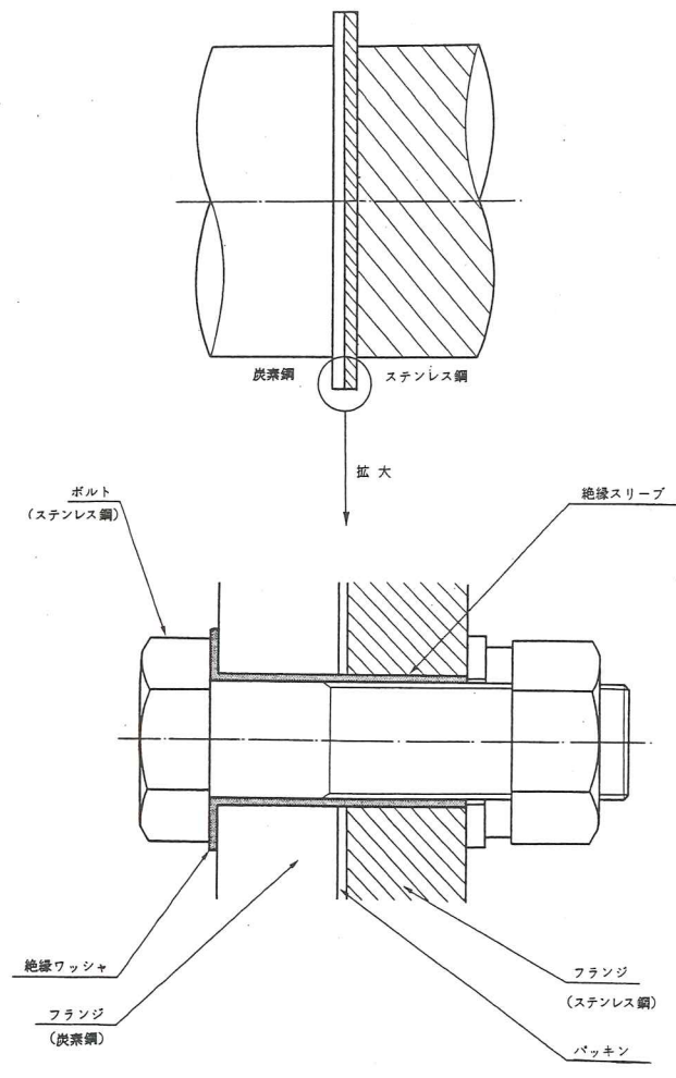
図解 - 5.11 フランジ接合部の絶縁
