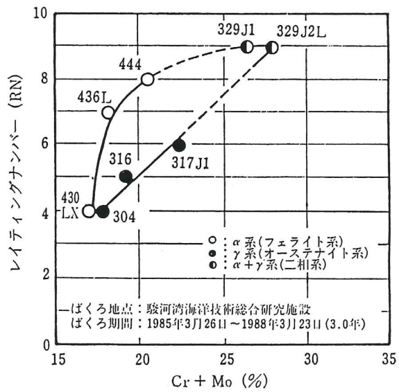
図解-2.14 無塗装ステンレ鋼の実海域ばくろ試験における耐さび性と合金成分との関係
