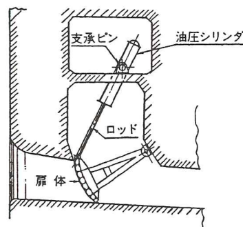
図解－5.5 油圧式開閉装置の例
