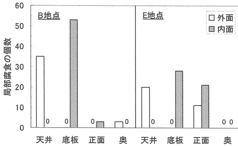
(a) 孔食の発生個数
