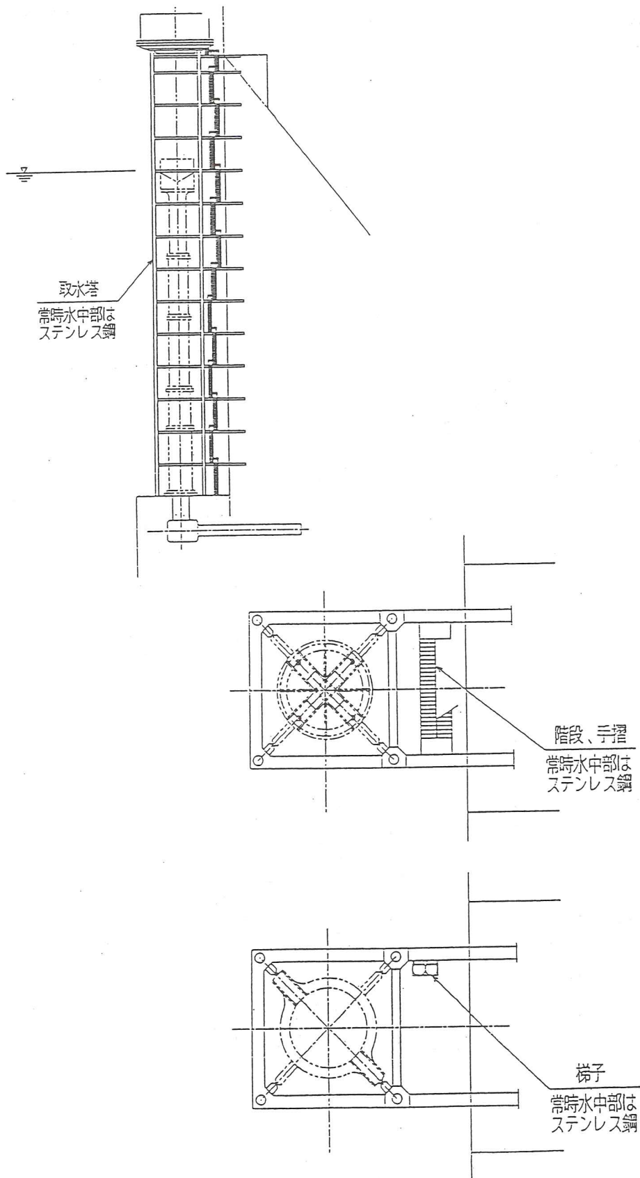
図解-3.16 鋼製取水塔（堤体付きの例）
