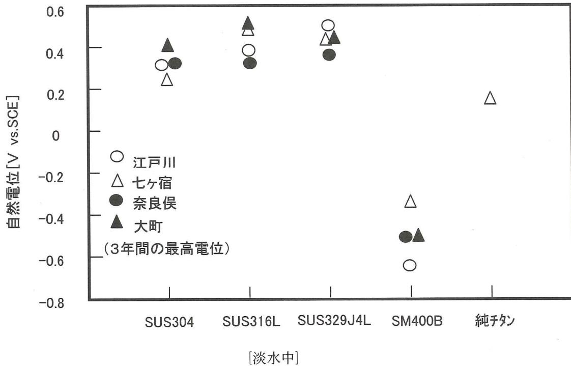
図解-2.20 各種金属およびステンレス材料の自然水中での自然電位
