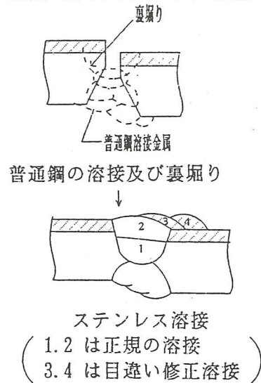
図解-4.7 目違いが大きい場合の溶接方法の例
