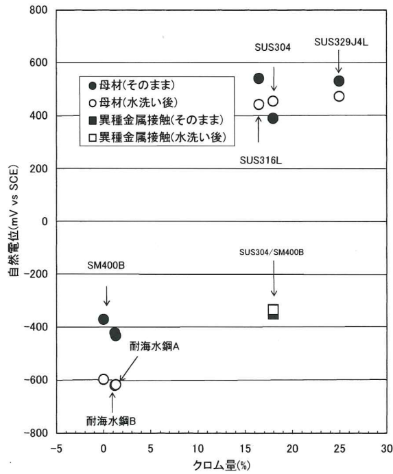
図解-2.44 母材腐食試験における自然電位 (江戸川上流水中部)
