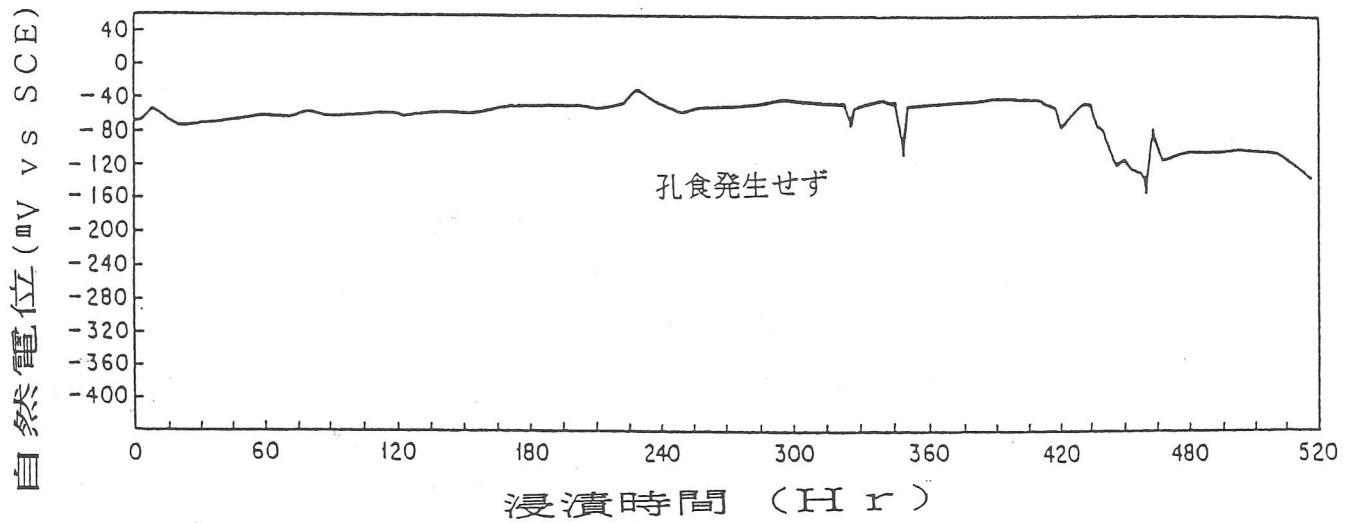
図解-2.36 20ppmCl - 単味溶液中での SUS304 の自然電位の経時変化
