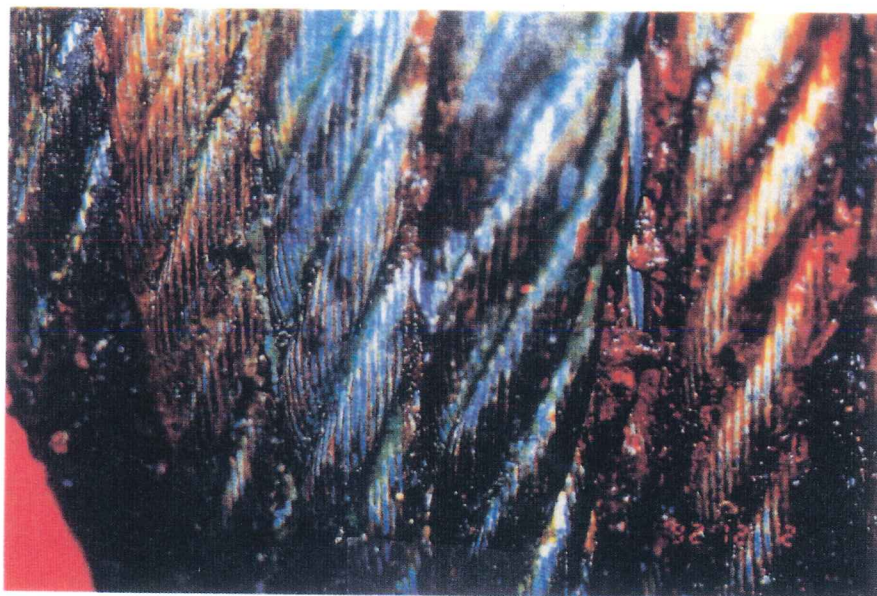
写真解-5.4 ワイヤロープ(常時水中部)の素線切れの例
