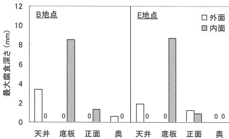
(b) 最大孔食深さ
