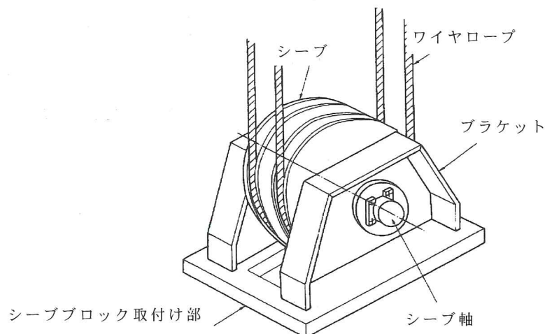
図解-3.8 シーブブロックの例
