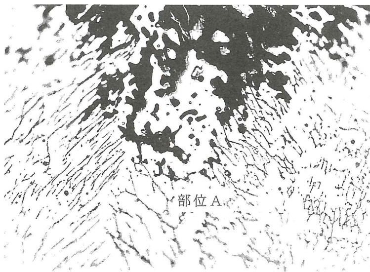
写真解-2.8 板状大型試験片(土中設置試験片)〔上段・外面〕の溶接部に発生した孔食・すき間腐食測定結果
