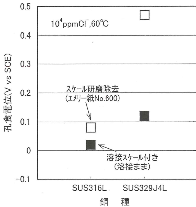
図解-2.39 ステンレス鋼の熱影響部の溶接スケールによる耐孔食性の劣化 (TIG共金溶接材) (ステンレス鋼便覧第3版)
