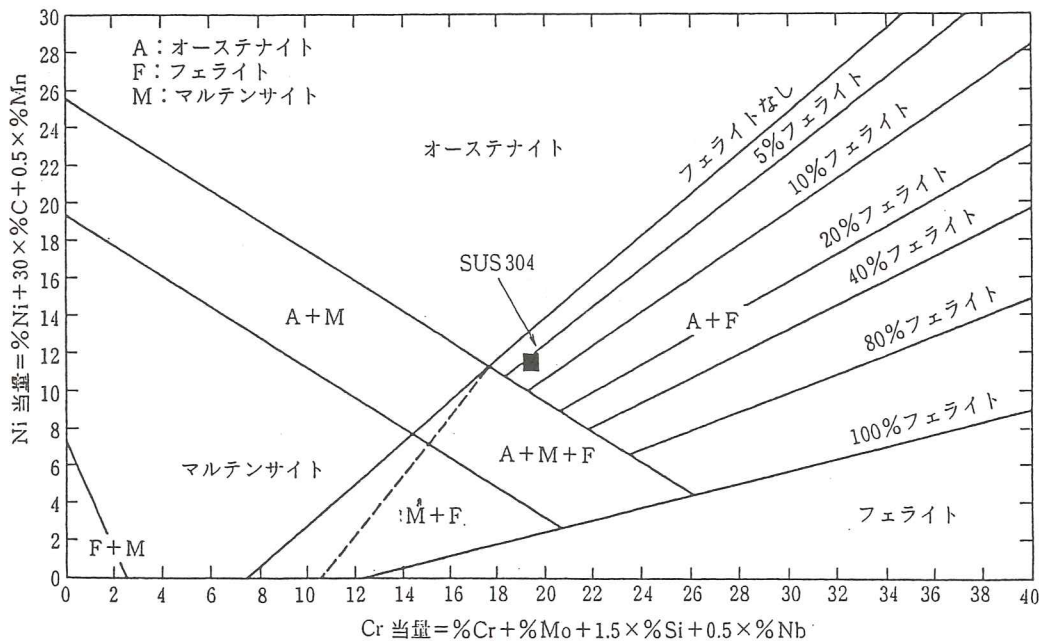
図解-2.4 シェフラーの組織状態図 (ステンレス鋼便覧-第3版)
