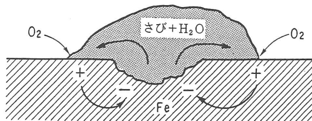
図解-2.34 鉄の表面に存在するさびによって形成された通気差電池(腐食反応とその制御)
