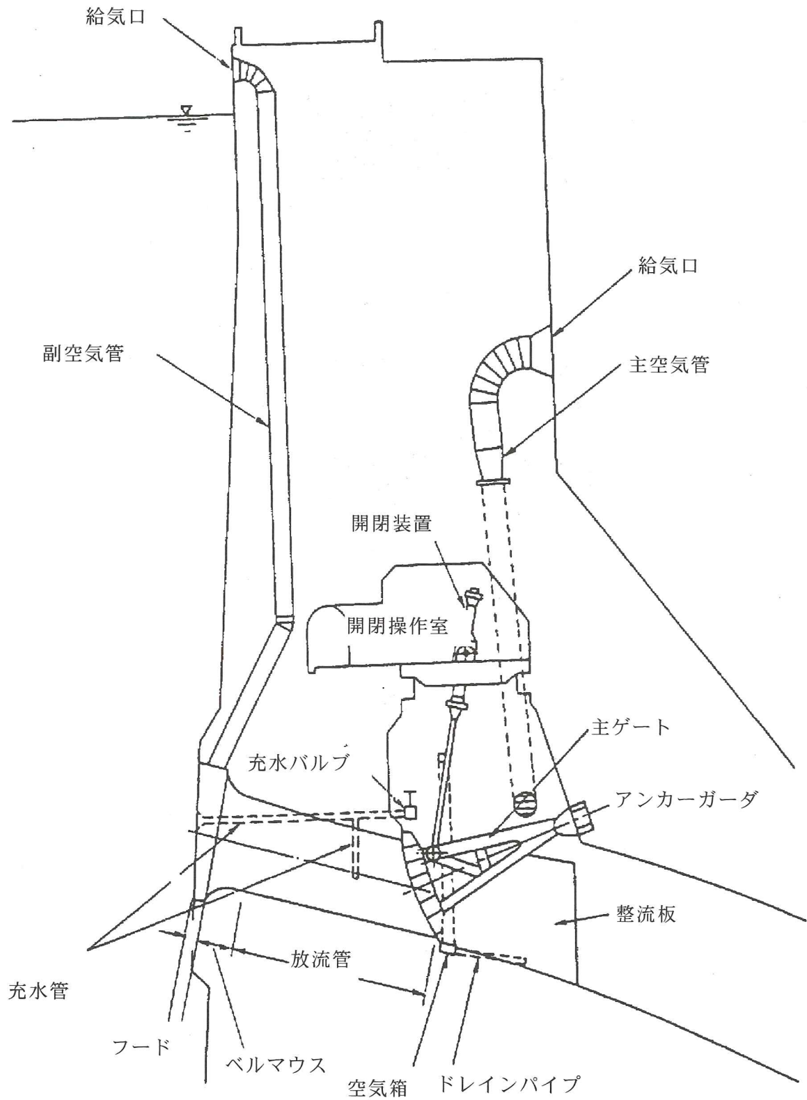
図解-3.10 大容量放流管の構成 (部分管路型の例)
