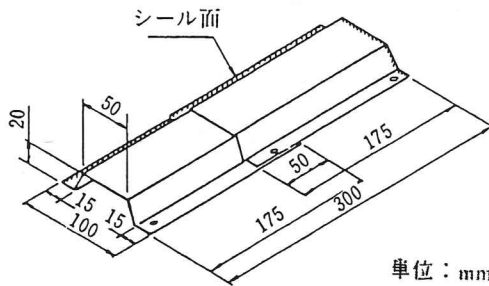
実海域ばくろ試験用試料形状
