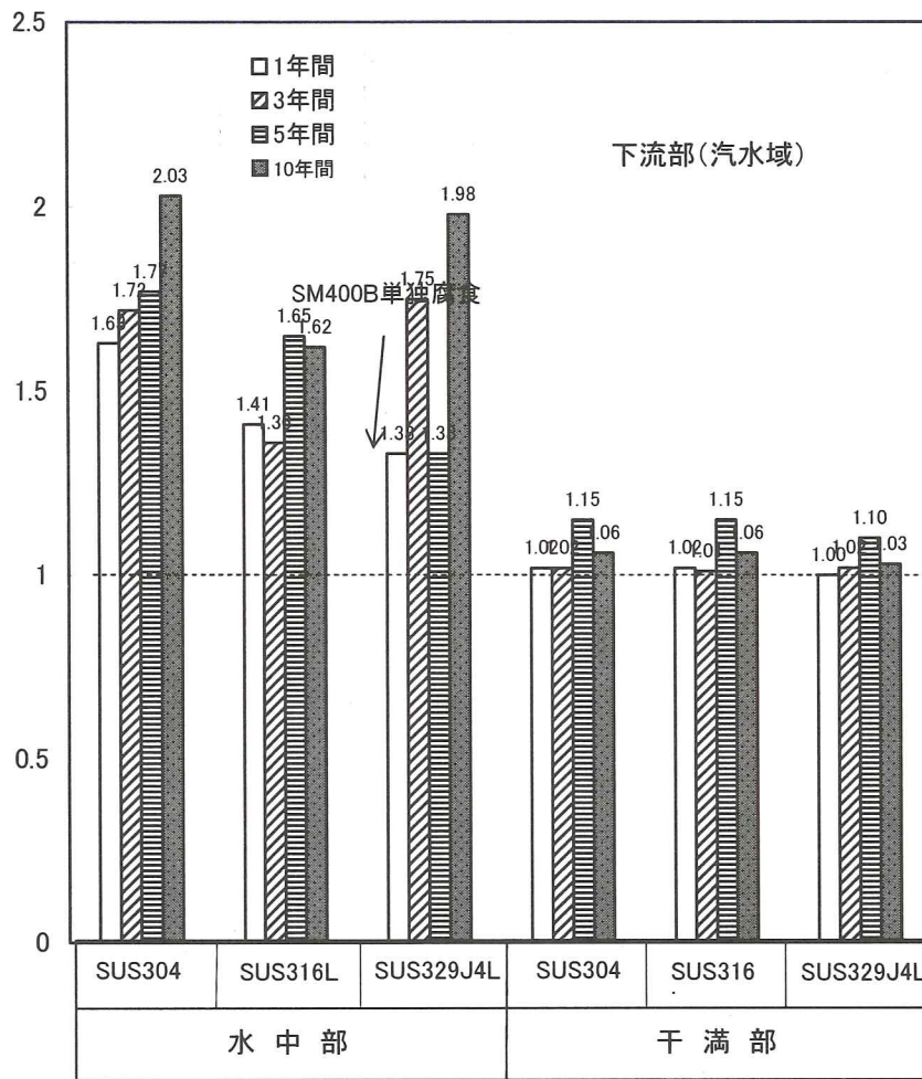
図解-2. 31 SM400B の異種金属接触腐食による相手材(カソード材料)に及ぼす腐食性の倍率 [下流部(汽水域), SUS/SM400B の面積比=1 : 1]
