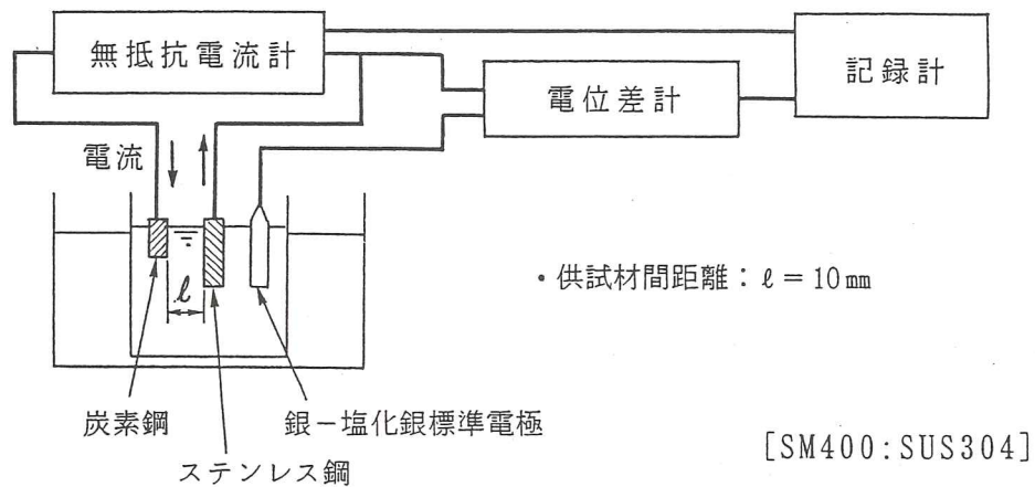
図解-2.25 カップル電流試験の試験方法
