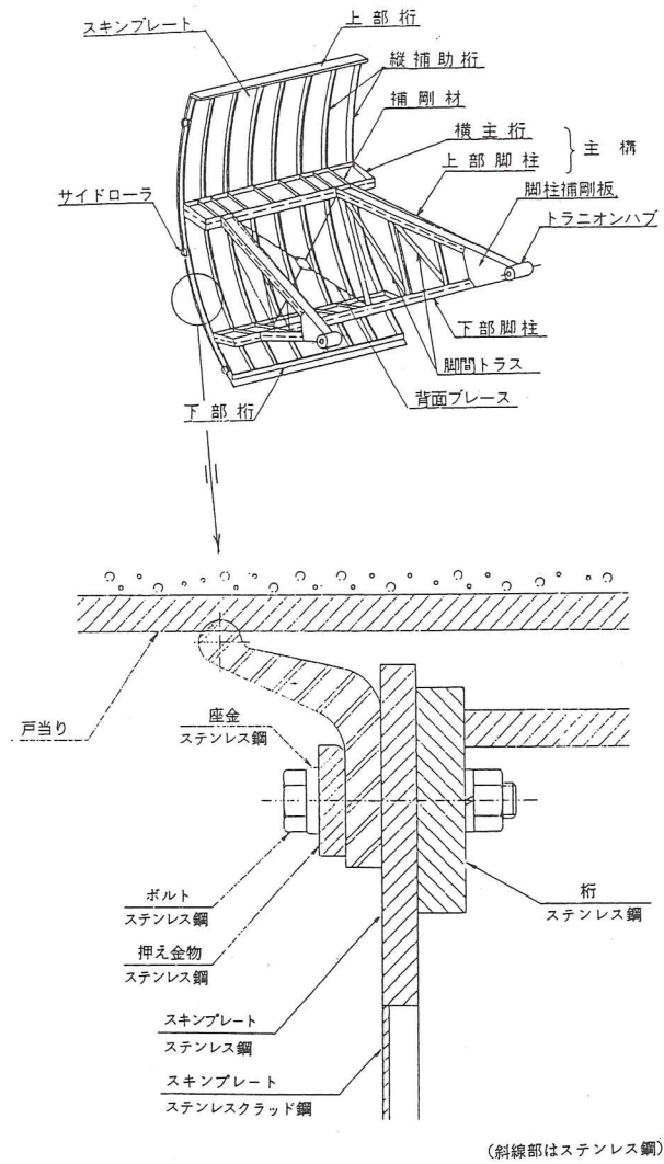
図解 - 5.10 水門扉側部水密部 (水密ゴム押さえ金物と固定ボルト)
