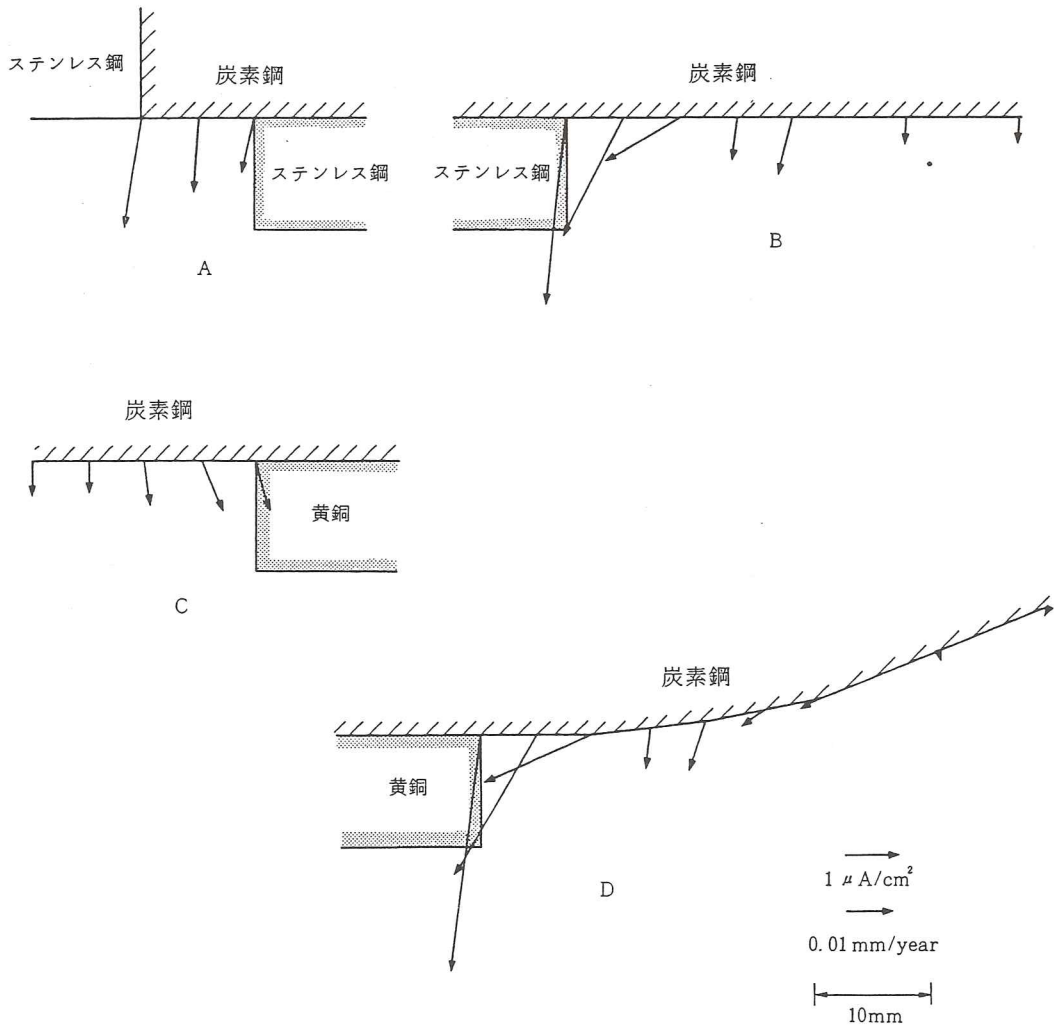
図解-2. 29 戸当り部の電位分布および腐食電流の計算結果
