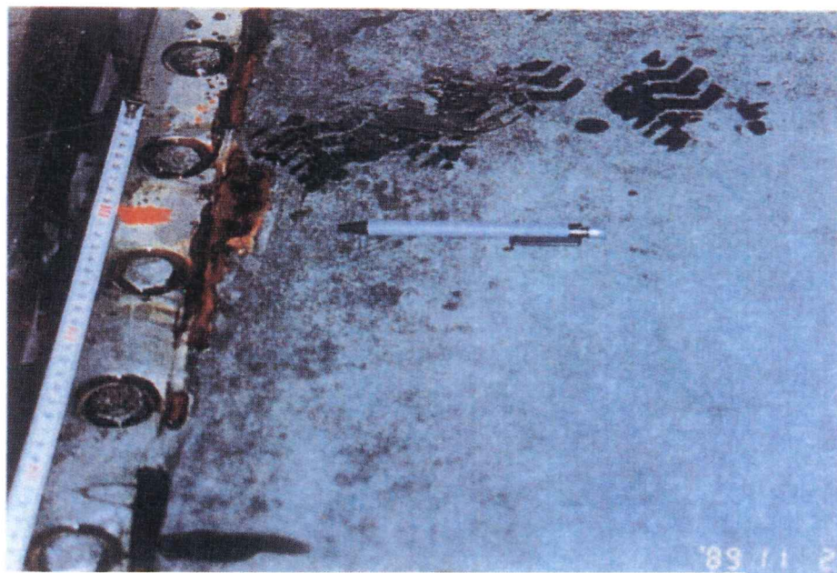
写真解－5.9 異種金属接触腐食の事例
