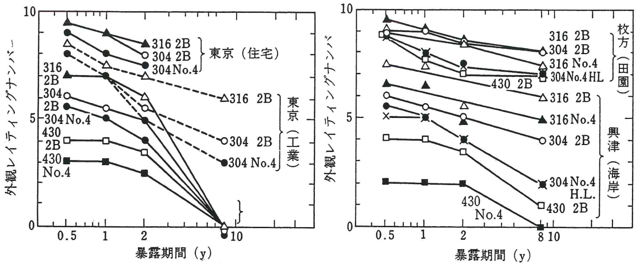
図解-2.12 各種環境におけるステンレス鋼の耐候性 (外観レーティングナンバー経時変化) (ステンレス鋼便覧第3版)
