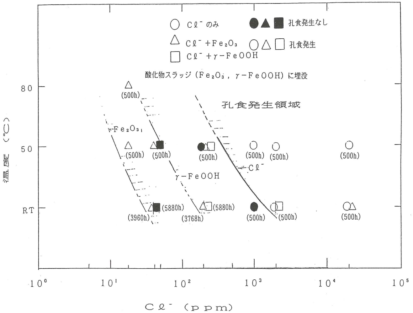
図解-2.35 SUS304の孔食感受性に及ぼすもらい錆の影響
