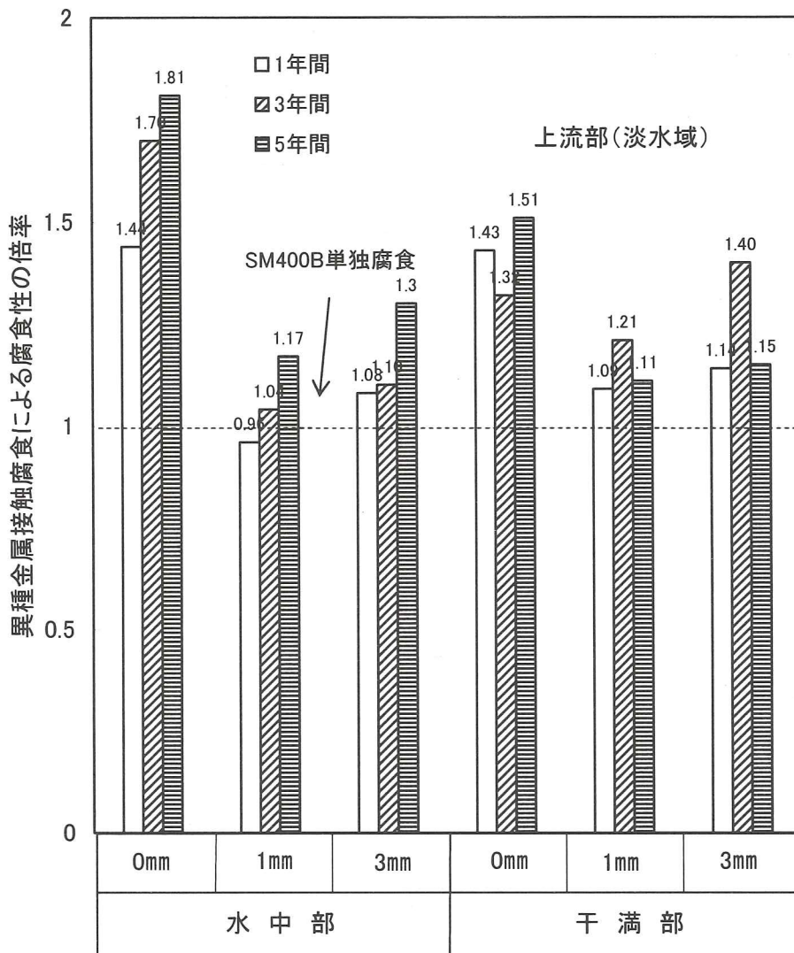
図解-2.30 SM400Bの異種金属接触腐食によるすき間距離に及ぼす腐食性の倍率 [上流部(淡水域), SUS304/SM400Bの面積比=1:1]
