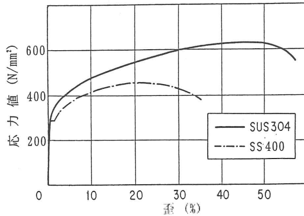
図解-2.7 応力／ひずみ曲線
