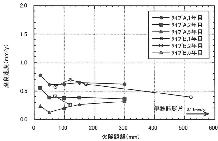
図解-3.1 塗装端からの欠陥距離とその位置での腐食 100mm 以上
