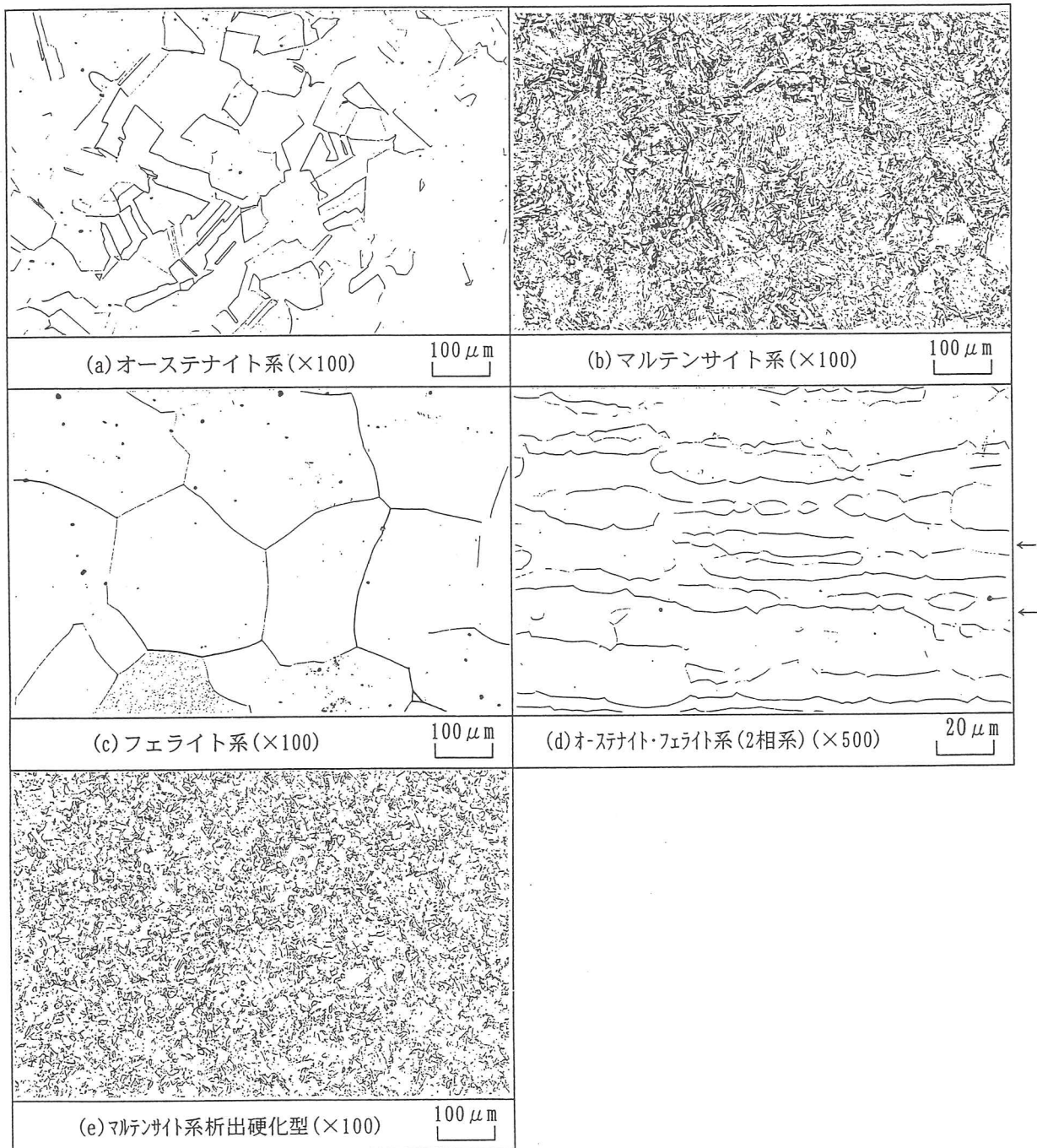
写真解-2.1 ステンレス鋼の顕微鏡組織の分類
