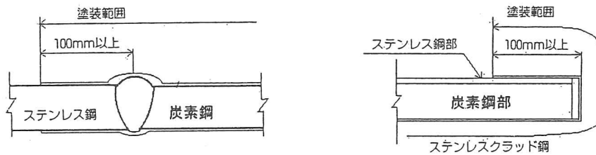
図解-5.8 ステンレス鋼と炭素鋼の接触部の塗装例
