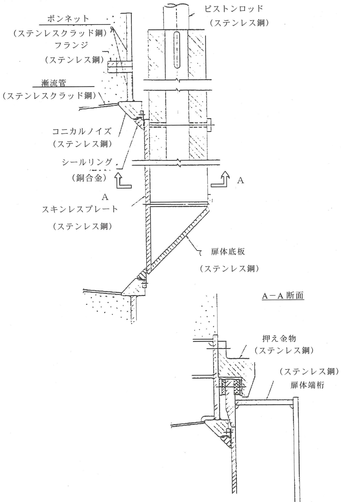
図解-3.14 扉体緒および水密部例 (ジェットフローゲートの場合)
