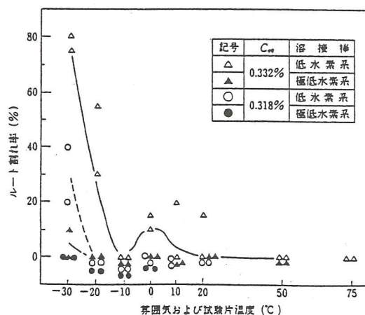
図解-4.9 低温雰囲気における溶接割れ試験結果
