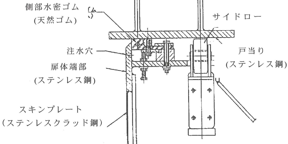
図解-3.6 扉体端部の例 (高圧ラジアルゲートの例)
