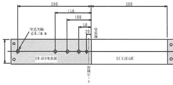
タイプ A 暴露試験片 (炭素鋼側塗装)
