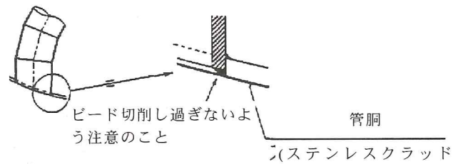
管胴継手部詳細
