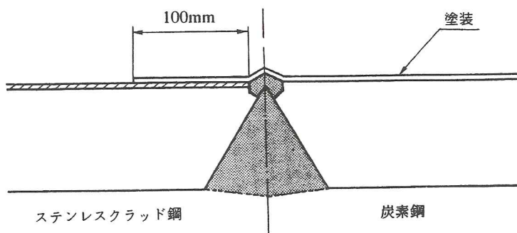
図解-3.2 塗装の塗り越し
