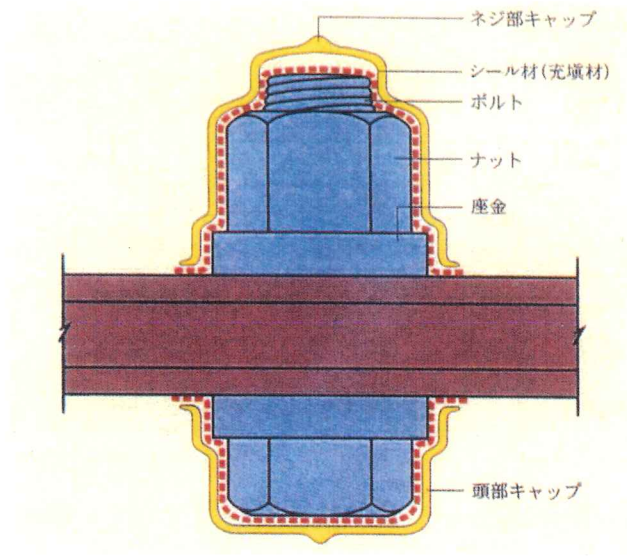
図解 - 5.13 ボルトキャップの取付状況
