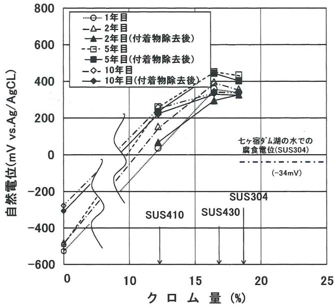
図解-2.43 七ヶ宿ダム湖暴露試験 10年経過までの自然電位測定結果
