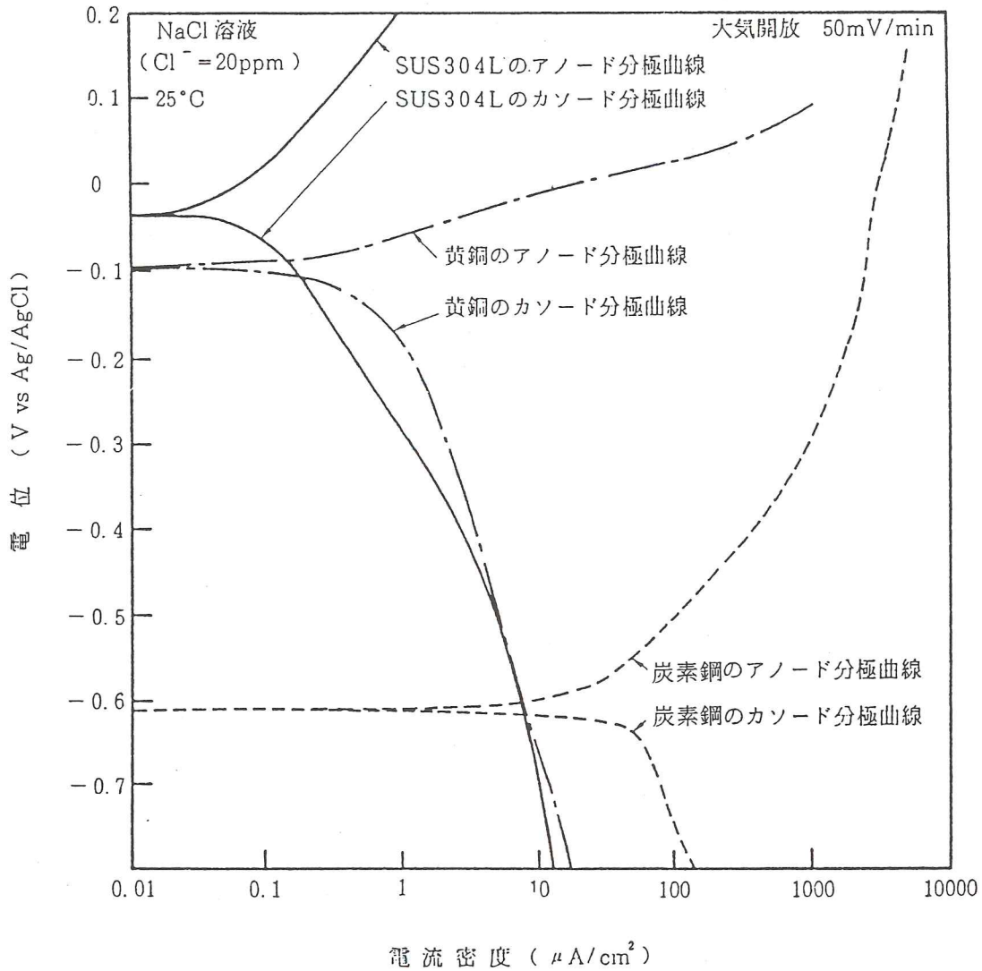
図解-2.28 分極測定結果 (20ppm NaCl 溶液中)
