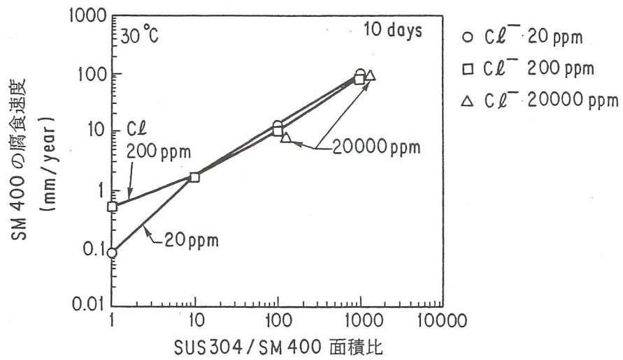
図解-2.26 異種金属接触腐食に与える面積比（ステンレス鋼：炭素鋼）の影響
