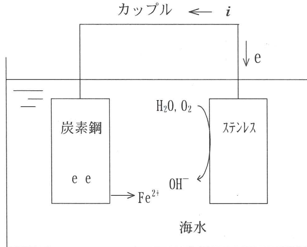
図解-2.21 異種金属接触腐食現象
