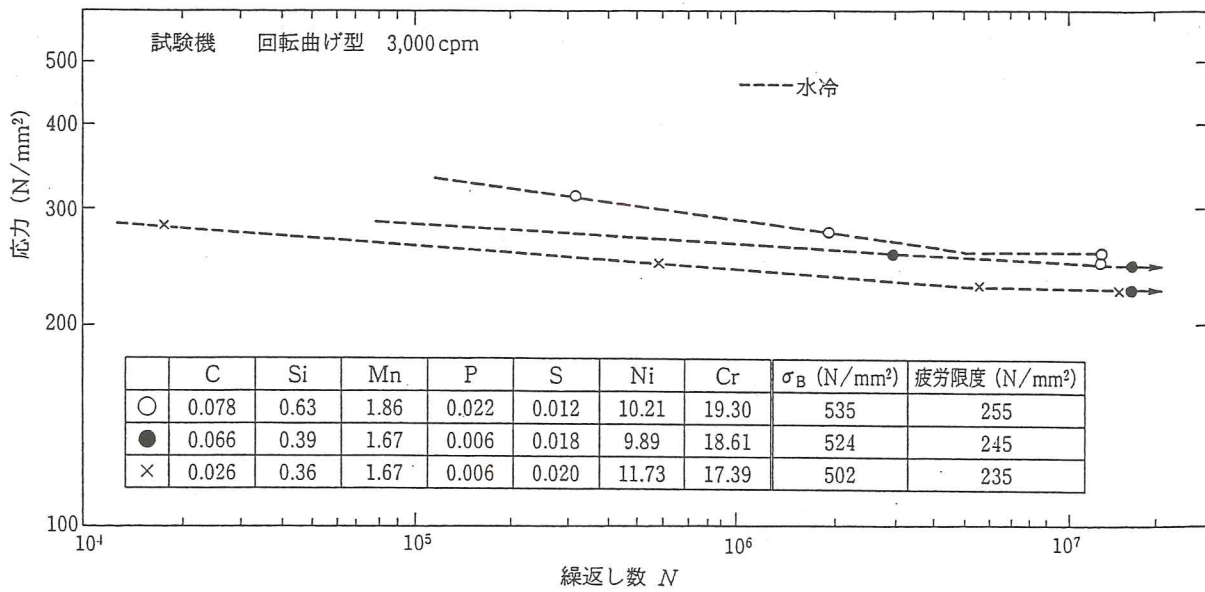
図解-2.8 SUS304 の S-N 曲線
