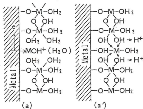
図解-2.11 結合水を考慮した不動態皮膜モデル (柴田俊夫：岡本剛教授退官記念論文集、P65 (1969))
