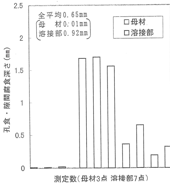
図解-2.46 板状大型試験片(水中設置試験片)・内面 孔食・すき間腐食測定結果 (SUS304, H9年7月10日~H9年10月29日)
