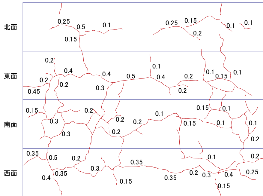
89093 5A ひび割れ状況 c3
