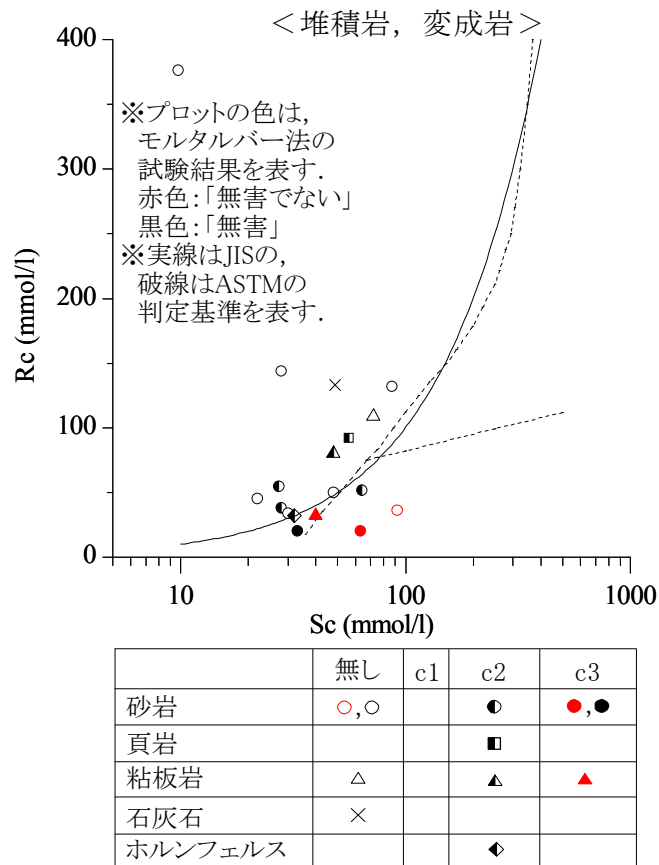
図-5.3.1 堆積岩, 変成岩のアルカリシリカ反応性試験結果と暴露供試体のひび割れ状況の関係 (アルカリ量 5\text{kg/m}^3 )
