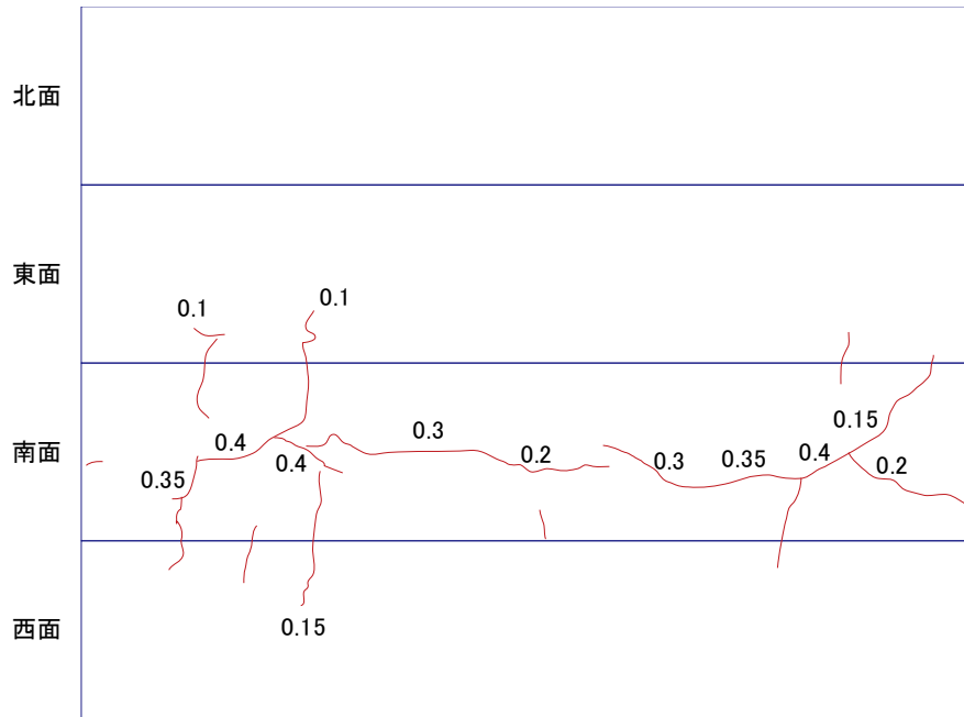
89093 3B ひび割れ状況 c3
