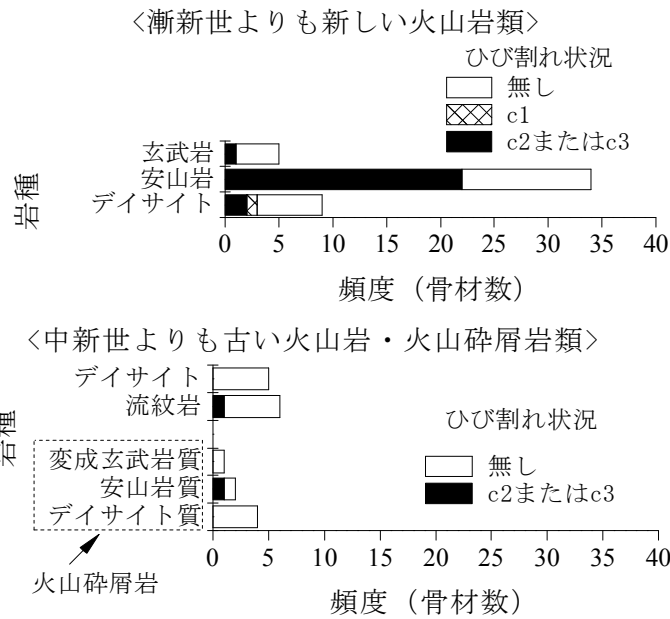
※図中に示さないものとして、地質年代が推定できなかった骨材が、安山岩に2試料、デイサイトに1試料あった。 図-5.2.2 地質時代で区分した火山岩、火山碎屑岩の暴露供試体のひび割れ状況 (アルカリ量 5\text{kg/m}^3 )
