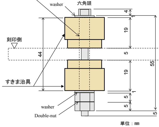
図 3.2.4 すき間治具詳細
