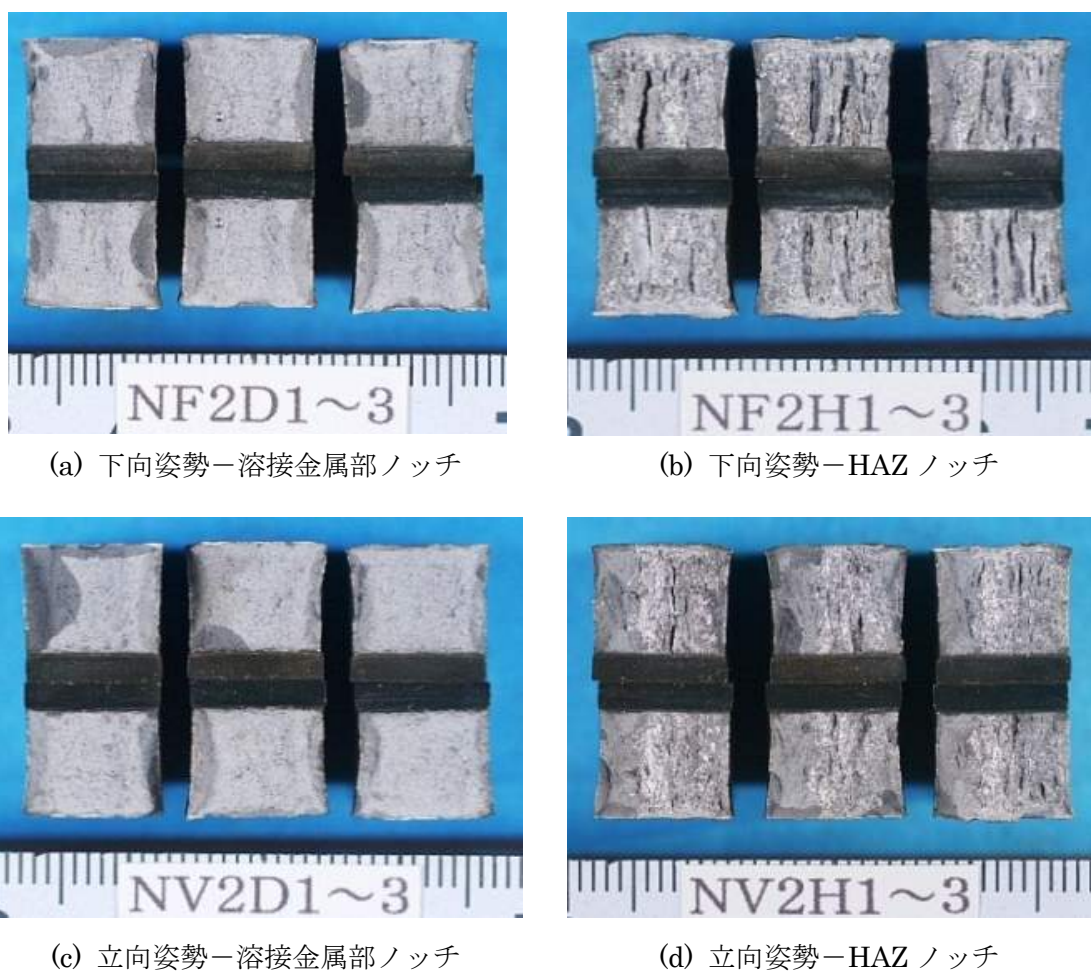
図 2.3.9 シャルピー衝撃試験片の破面
