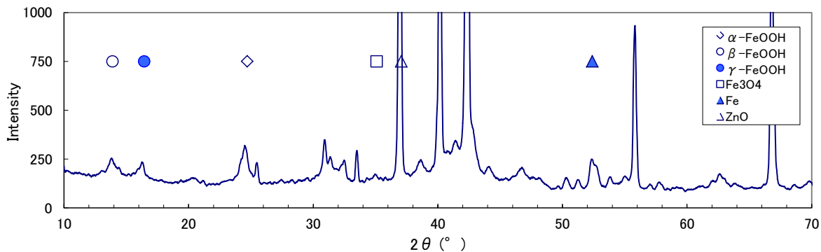
図 3.6.4 暴露 1 年後の SM400B に生じたさびの X 線回折パターン
