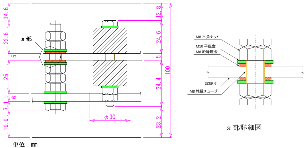
図 3.2.7 試験片締結部構造
