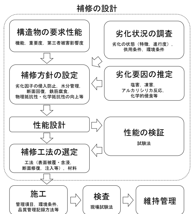
解説 図-2.4.1 補修工法検討の流れ
