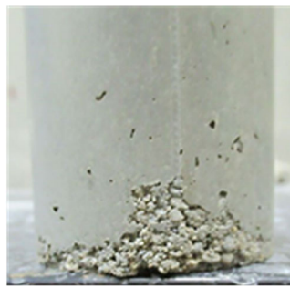
(2) 乾式吹付け工法 (豆板発生の場合)
