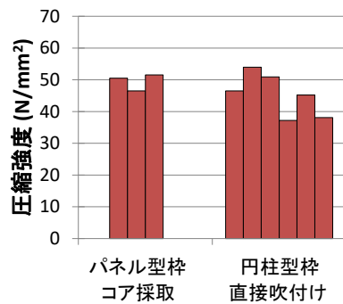
(2) 乾式吹付け工法
