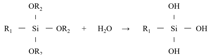
a. 第一段階: 加水分解反応
