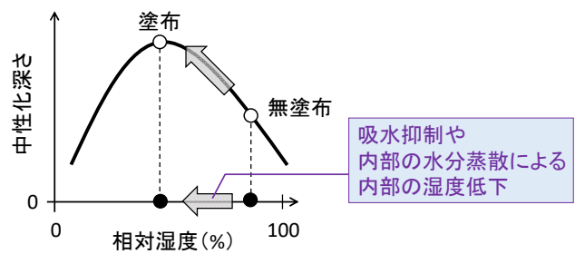
解説 図-5.3.5 シラン系表面含浸材塗布箇所の中性化促進要因〔含〕 6)
