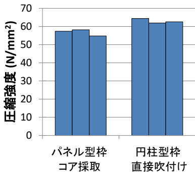
(1) 湿式吹付け工法
