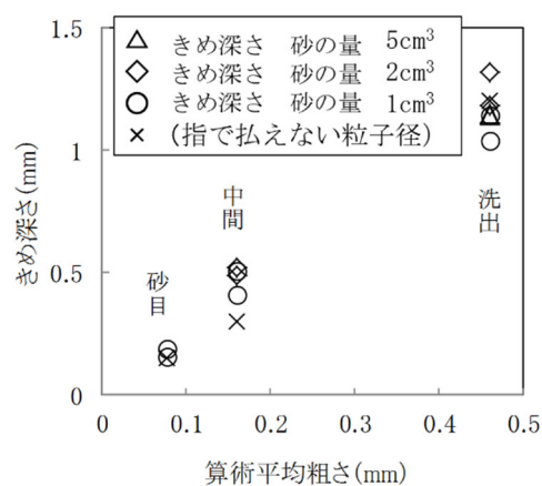
解説 図-2 算術平均粗さときめ深さ、指で払えない砂の粒子径の関係
