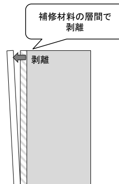
解説 図-2.1.7 塗り重ねた新設塗膜の 既設塗膜からの剥離〔被〕
