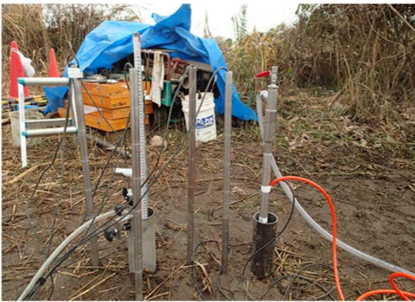
図-4 現地試験状況
