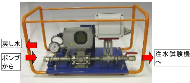
図-6 流量制御装置
