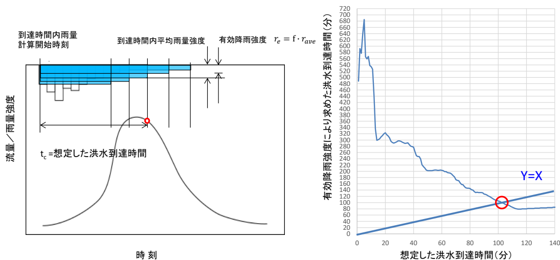
図 3-2-3 洪水到達時間の求め方
