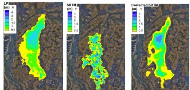
図-14 破堤9時間後の洪水氾濫シミュレーション結果 (LP データ (左)、SRTM 補正前 (中央)、SRTM 補正後 (右))
