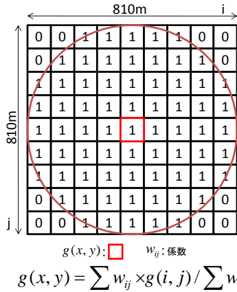
図-9 適用した9×9のローパスフィルタの係数
