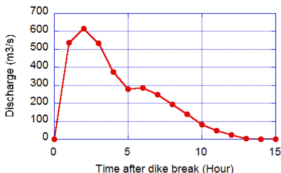
図-3 破堤流量のハイドログラフ
