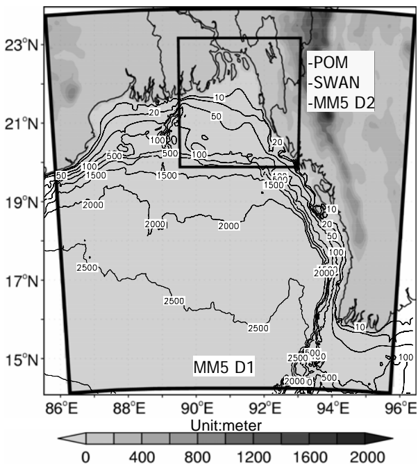
図-7 計算領域
