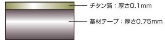
チタン箔シートの構成
