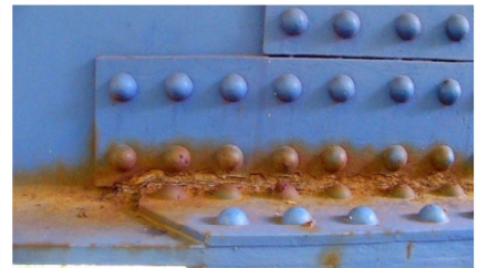
継手部（連結板）
