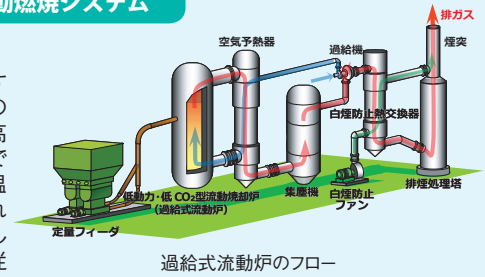
過給式流動炉のフロー
