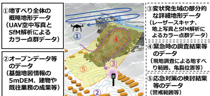
地すべり災害対応のBIM/CIMモデルの構成
