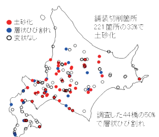
橋梁床版の土砂化・層状ひび割れが顕在化
