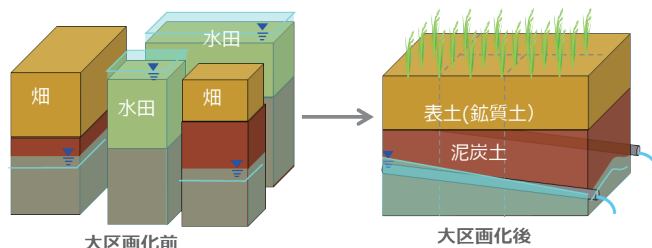
利用履歴の異なる圃場の大区画化に伴い発生する不同沈下への対応
