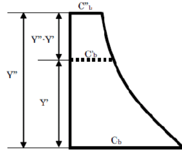
図 1 浮遊砂濃度分布図
