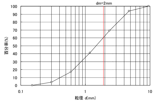
図-4 実験使用土砂の粒径分布
