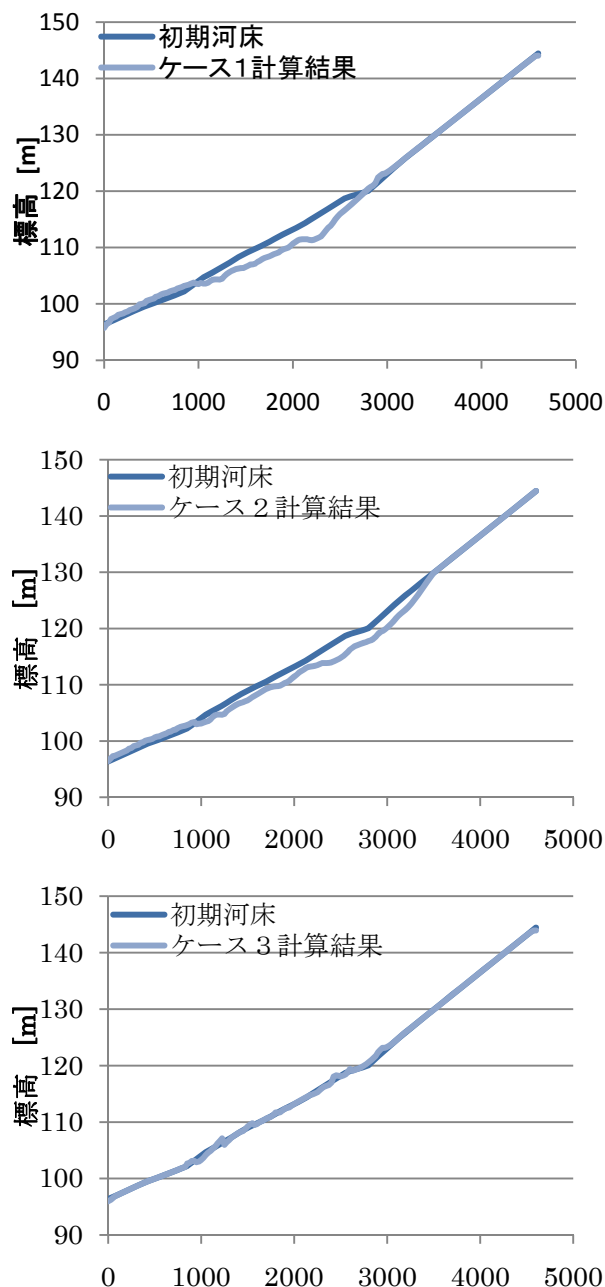
図-3 河床変動計算結果
