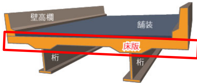
橋の構成(床版の位置)
