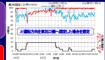
【風向固定の場合 目標VI 80%】
