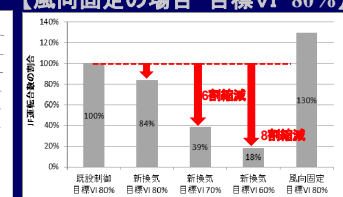
【JF運転時間の割合】
