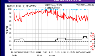
【新換気 目標VI 70%】
