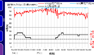
【新換気 目標VI 80%】
