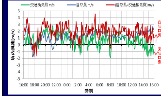
【風速成分(解析値)】
