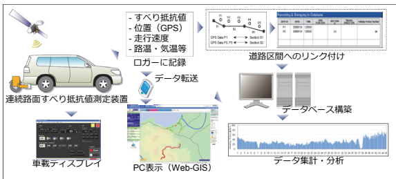
路面摩擦モニタリングシステム (特許公開2009-251741) システム構成図
