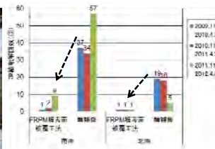
FRPM板で補修した場合と無補修の場合の水路躯体コンクリートの凍結融解回数※3
