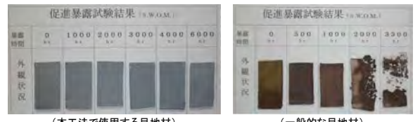
(本工法で使用する目地材) (一般的な目地材) ※JIS A 1415に準拠したサンシャインカーボンアークランプによる促進耐候性試験 10
