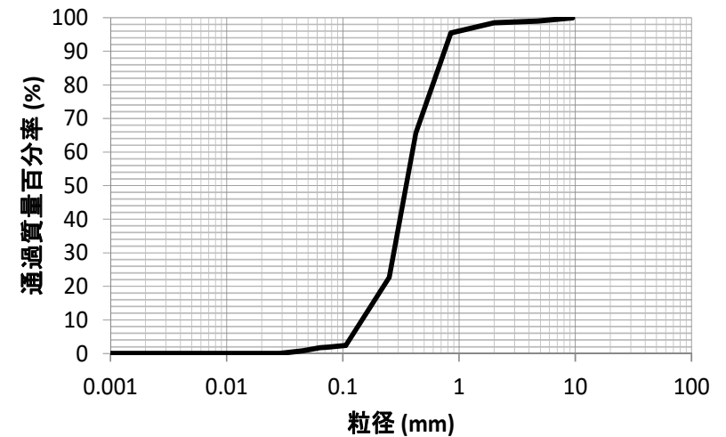
貯砂ダム上流の河床の粒径
