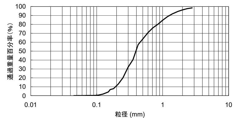
実験に用いた土砂の粒度分布
