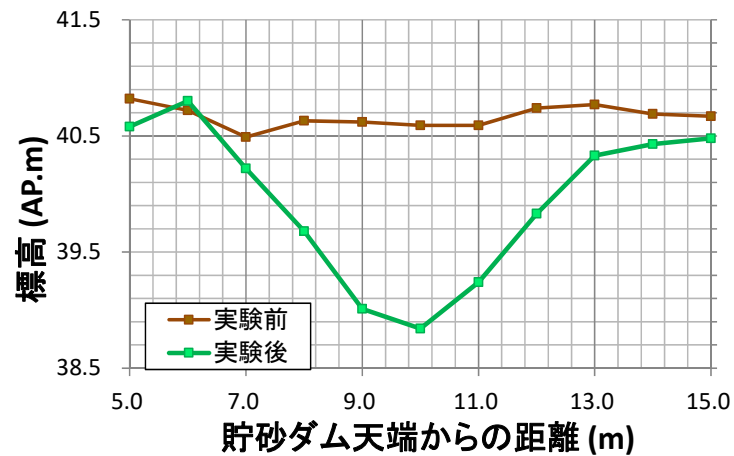
縦断面図
