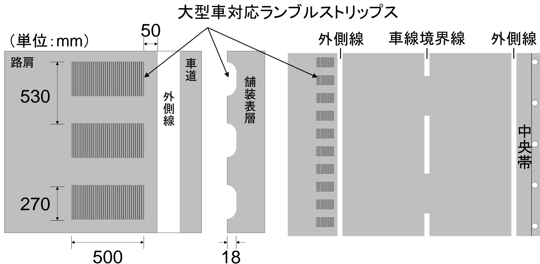
詳細図(推奨規格)
