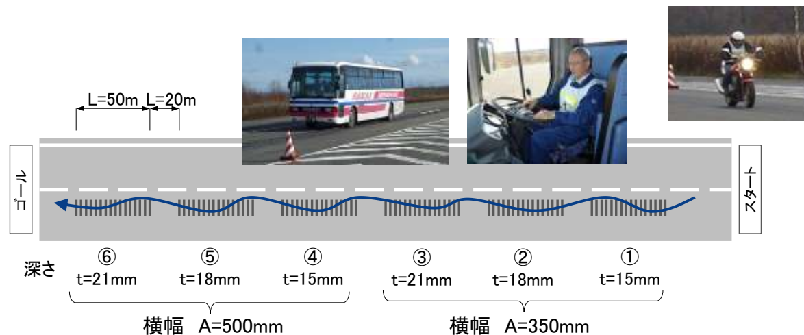
走行実験コース
