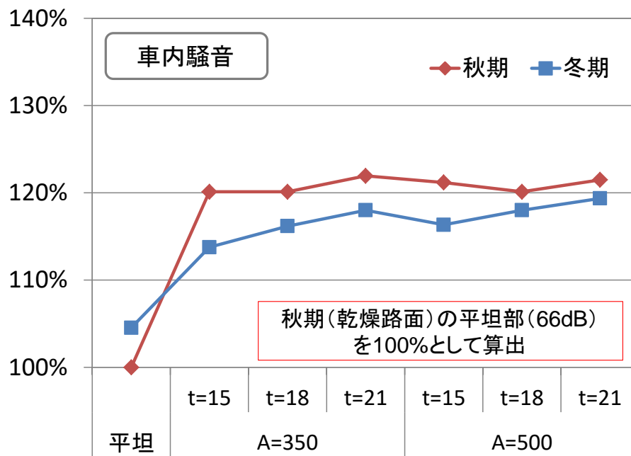
車内騒音(大型バス)
