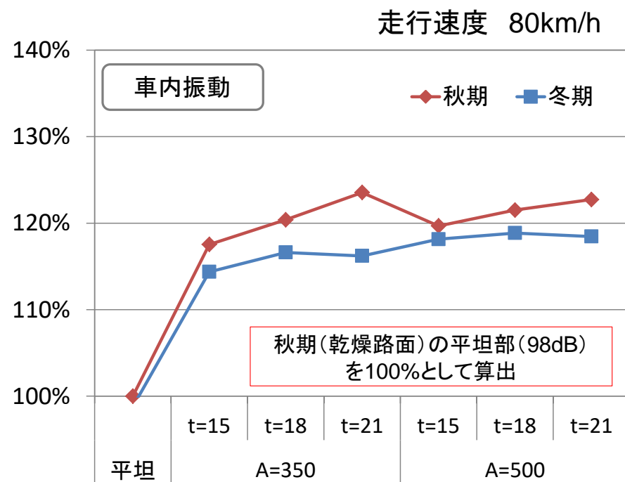
車内振動(大型バス)
