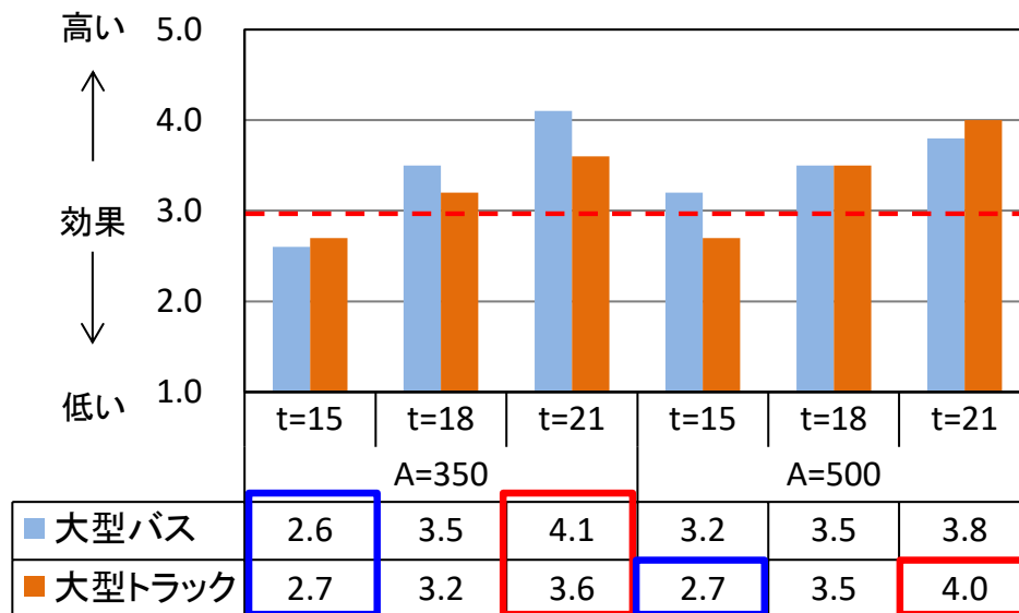
警告効果(冬期)
