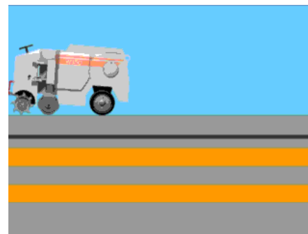
異径車輪による施工過程
