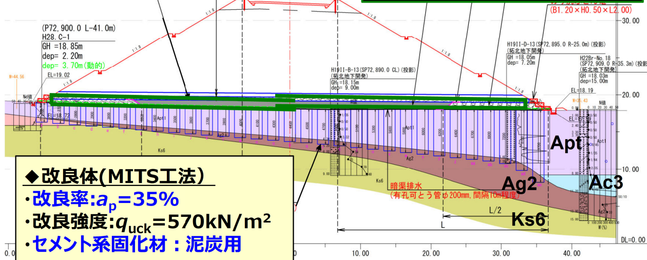
事例 1 : 対策工断面図 (SP=72,900)
