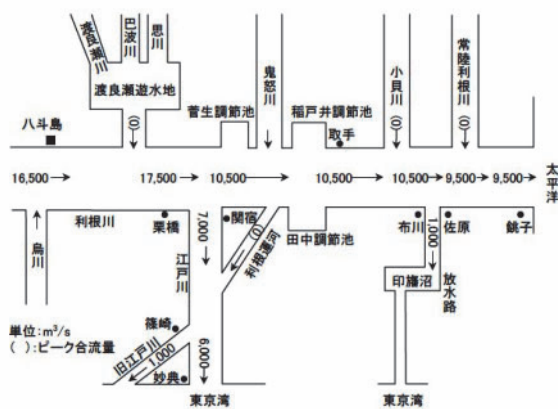
治水計画の例 (利根川の流量配分図)
