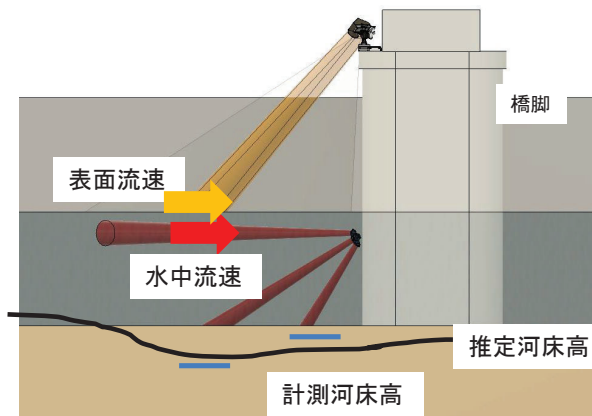
縦断面図
