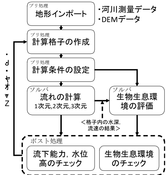
図-1 河道計画時に利用可能な環境評価ツールの概略
