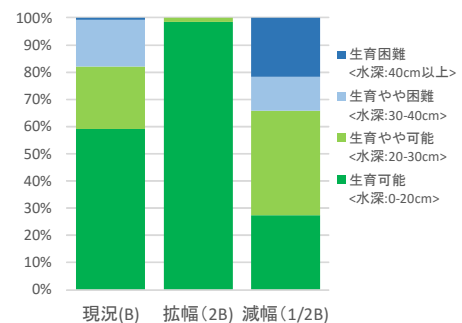
図-6 植物生育可否に関する評価
