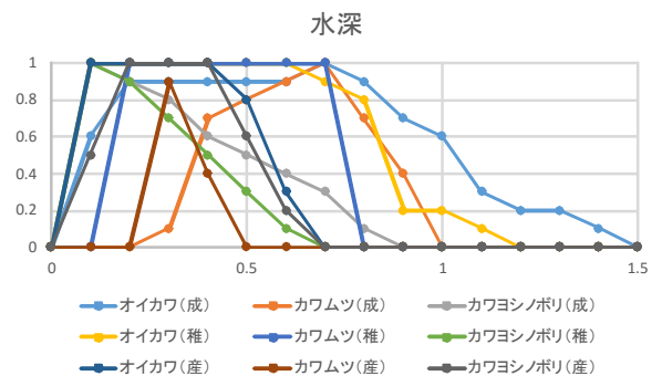
図-2 水深に対する生息場適性指数(例)
