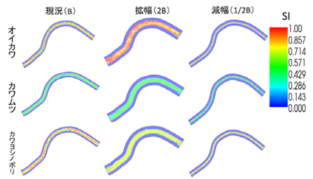
図-3 流速による評価結果例（成魚）
