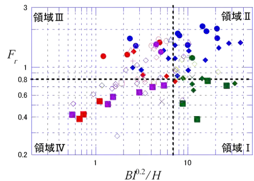
図-2 Bf^{0.2}/H とフルード数との関係
