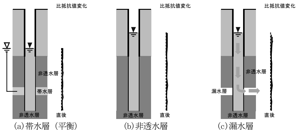
図解3-5 連続ステップ孔内試験での食塩検層（自然水位法）で流動が検出されない事例
