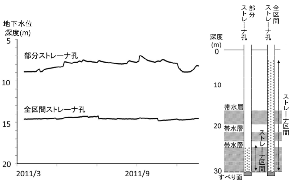
図1-1 部分ストレーナ孔、全区間ストレーナ孔による地下水観測例 (左：水位変動グラフ、右：観測孔の構造)
