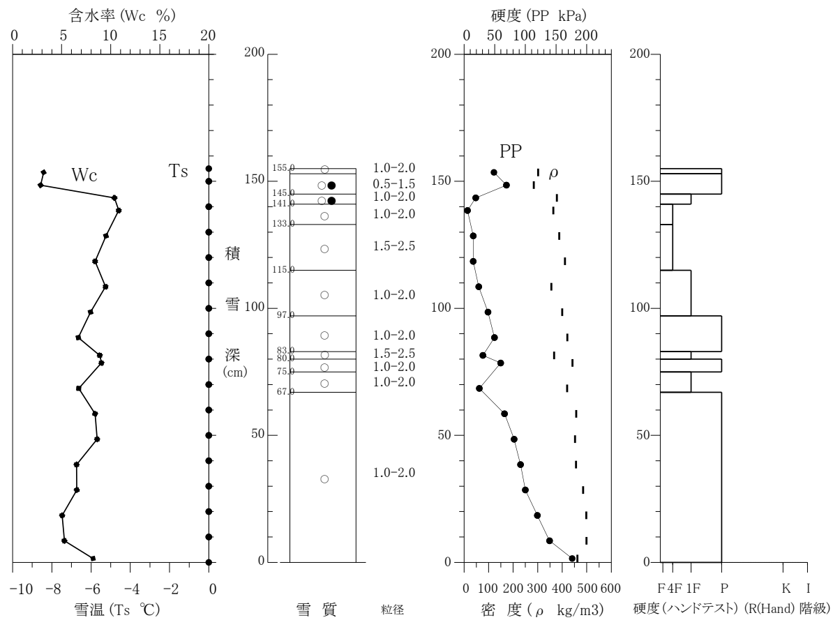
積雪断面観測値 (雪崩C構内 2015/02/05)
