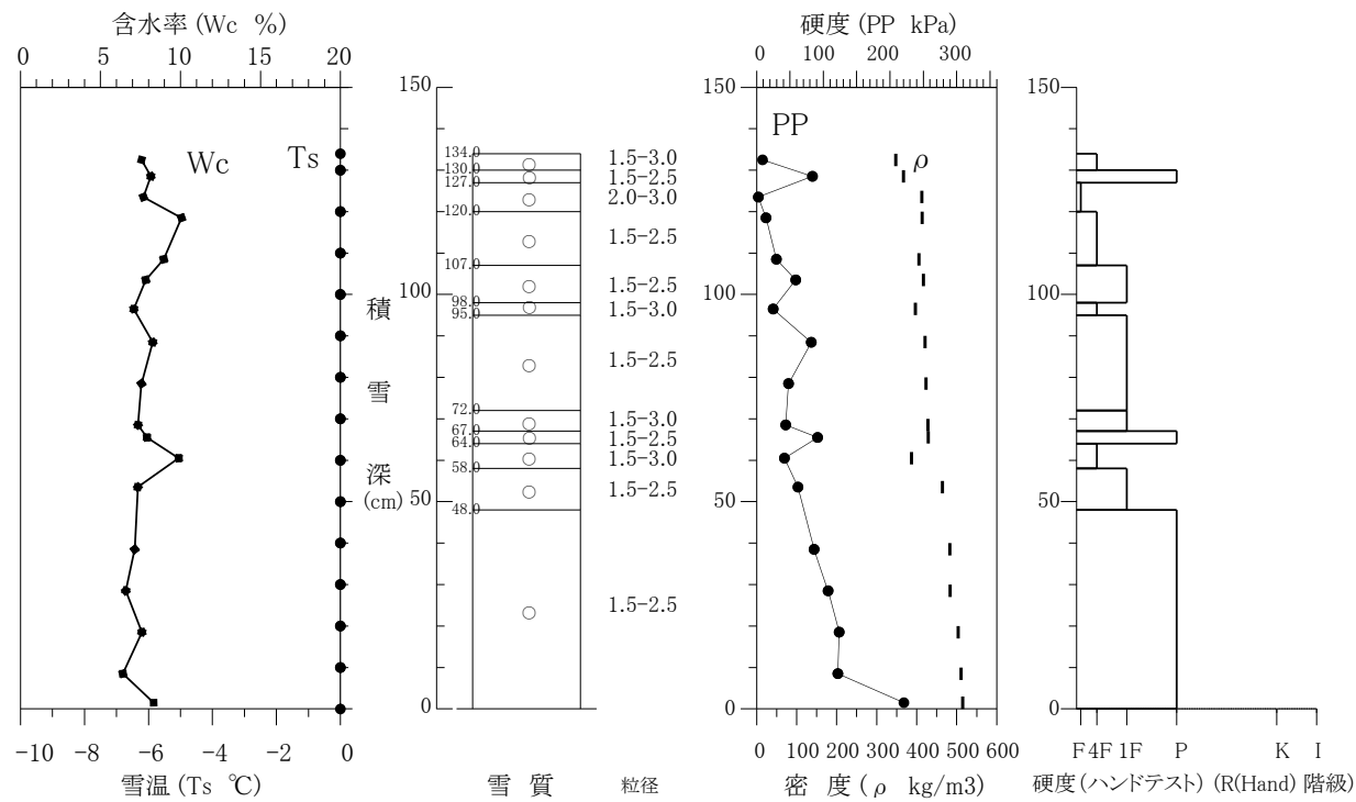
積雪断面観測値 (雪崩C構内 2015/02/25)
