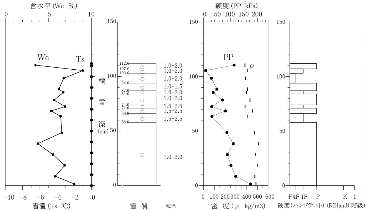
積雪断面観測値 (雪崩C構内 2015/03/05)
