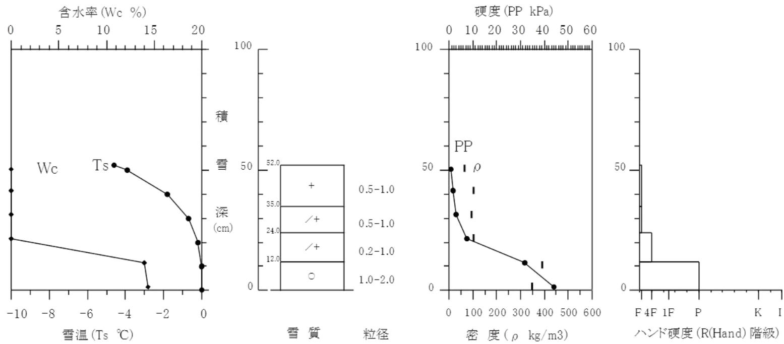
積雪断面観測値 (雪崩C構内 2016/02/16)
