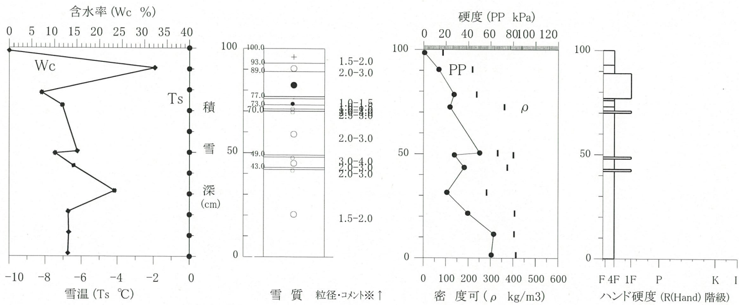
積雪断面観測値 (雪崩C構内 2017/02/15)
