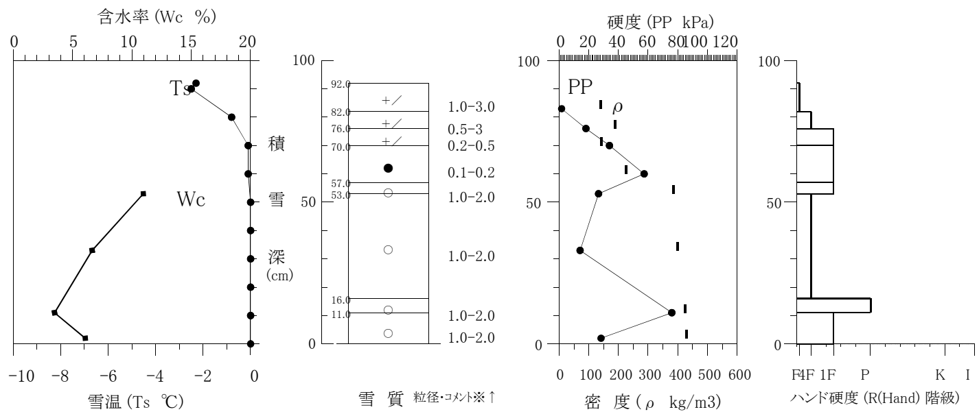
積雪断面観測値 (構内 2018/01/05)
