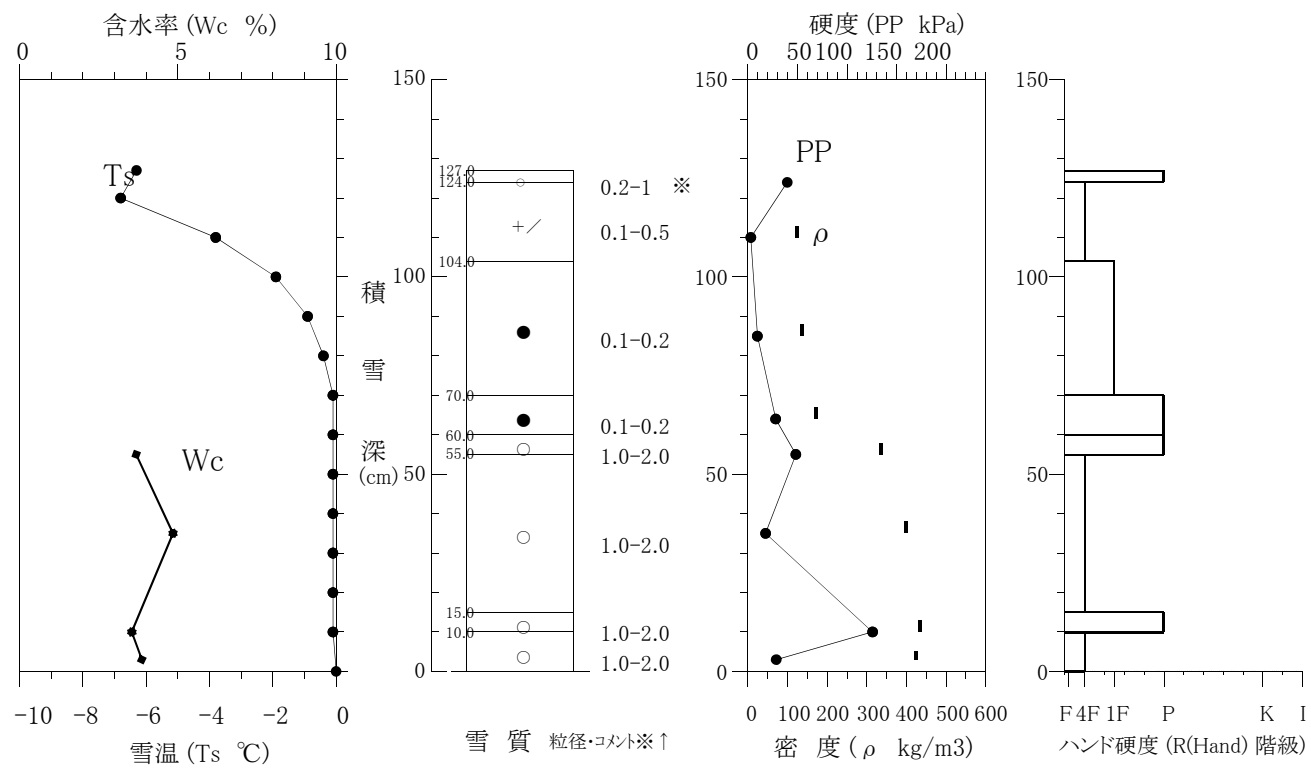
積雪断面観測値 (構内 2018/01/15)
