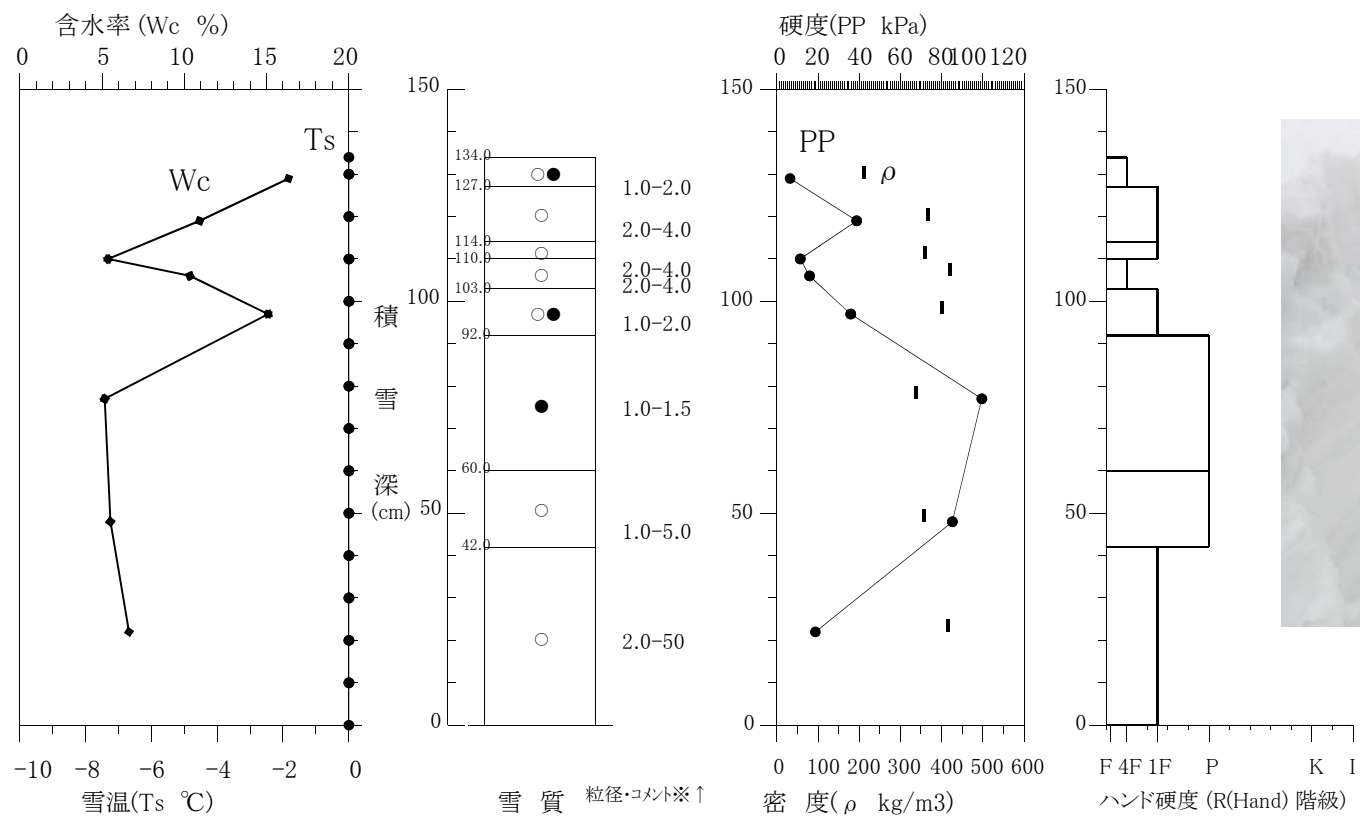
積雪断面観測値 (構内 2018/02/15)
