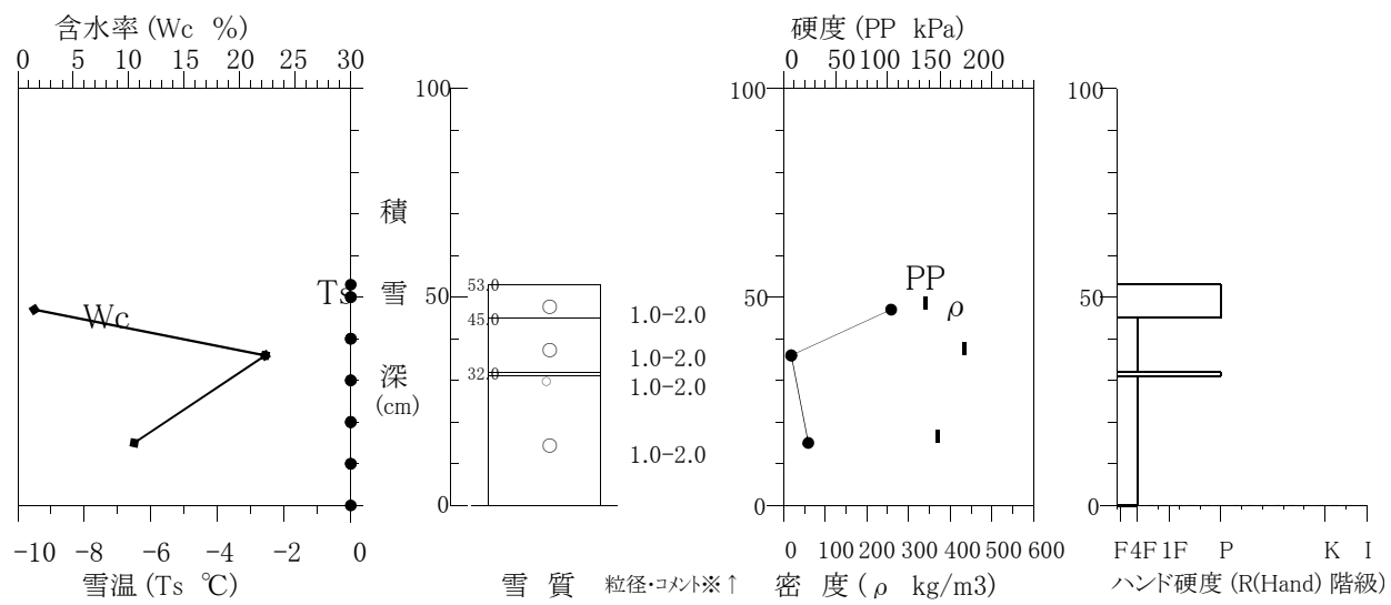
積雪断面観測値 (構内 2019/01/15)
